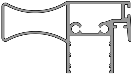
Sistem Kodu System Code 59-7007 Ağırlık (kg/mt) Weight (kg/mt) 1,128
