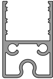
Sistem Kodu System Code 59-7009 Ağırlık (kg/mt) Weight (kg/mt) 0,671
