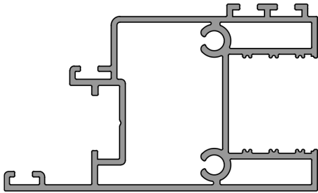
Sistem Kodu System Code 59-7012 Ağırlık (kg/mt) Weight (kg/mt) 1,173
