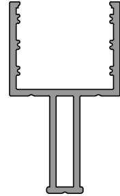
Sistem Kodu System Code 59-7011 Ağırlık (kg/mt) Weight (kg/mt) 0,498
