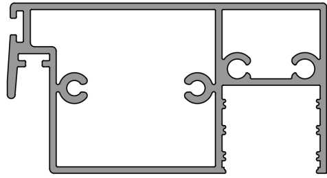
Sistem Kodu System Code 59-7008 Ağırlık (kg/mt) Weight (kg/mt) 1,396 ( 2" li kanat adaptörü )
