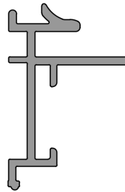
Sistem Kodu System Code 59-7013 Ağırlık (kg/mt) Weight (kg/mt) 0,495
