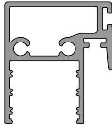
Sistem Kodu System Code 59-7010 Ağırlık (kg/mt) Weight (kg/mt) 0,807
