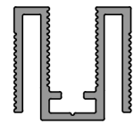
Sistem Kodu System Code 59-7015 Ağırlık (kg/mt) Weight (kg/mt) 0,353
