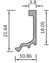
24 mm Cam Çıtası
