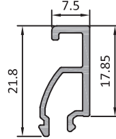
20 mm Cam Çıtası
