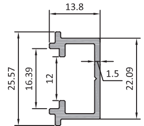
PVC İspanyolet Kanalı
