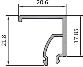
6 - 8 mm Cam Çıtası
