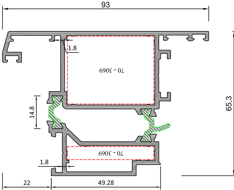
DIŞA AÇILIR KAPI KANADI
