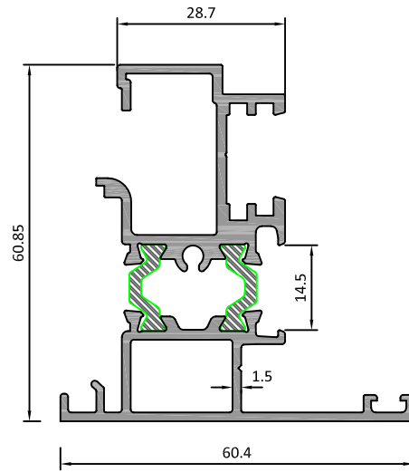
ÇİFT KANAT ADAPTÖRÜ (ALÜMİNYUM LEVYE KOL AKSESUARLI)
