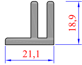
Sistem Kodu 50-1658 Ağırlık (kg/mt) 0,435
