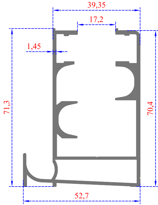
Sistem Kodu 41-2951 Ağırlık (kg/mt) 1,340
