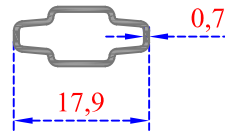
KAROLAJ ÇİTASI
