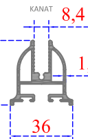
Sistem Kodu 41-2302 Ağırlık (kg/mt) 0,785
