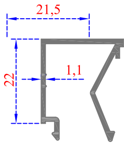
Sistem Kodu 49-4308 Ağırlık (kg/mt) 0,260
