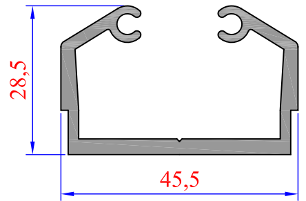
Sistem Kodu 50-1460 Ağırlık (kg/mt) 0,845
