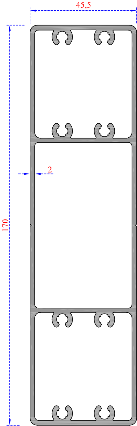
Sistem Kodu 50-1615 Ağırlık (kg/mt) 3,355
