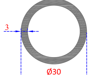
Sistem Kodu 22-209 Ağırlık (kg/mt) 0,690
