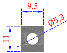
Sistem Kodu 58-2219 Ağırlık (kg/mt) 0,225
