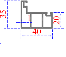
Sistem Kodu 41-2722 Ağırlık (kg/mt) 0,570
