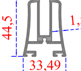
Sistem Kodu 41-2310 Ağırlık (kg/mt) 0,903
