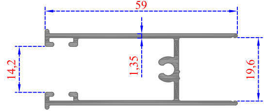
Sistem Kodu 54-4736 Ağırlık (kg/mt) 0,593
