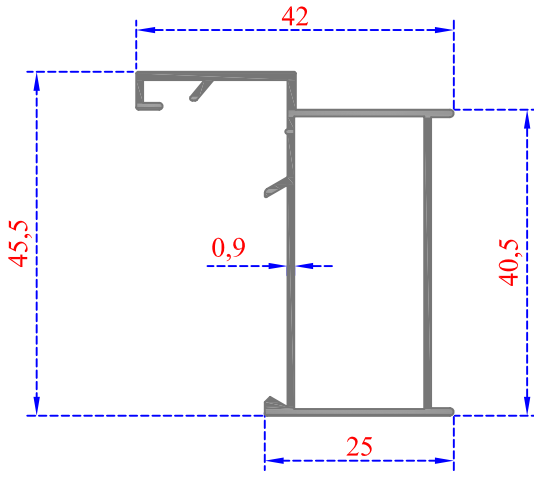
KASA
