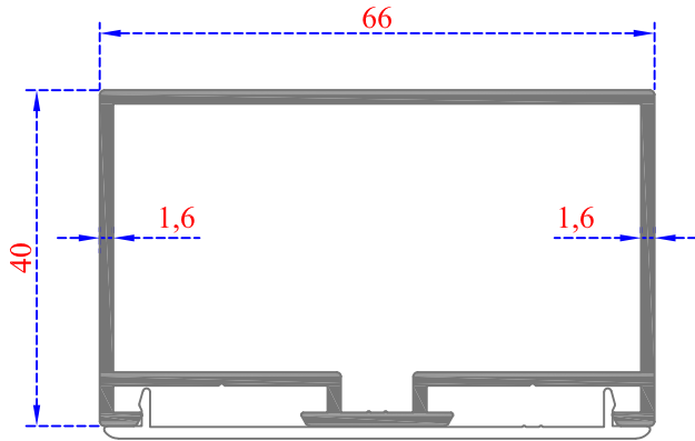
Sistem Kodu 54-4705
