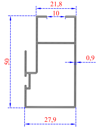
Sistem Kodu 49-4383 Ağırlık (kg/mt) 0,435
