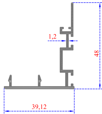
Sistem Kodu 49-4378 Ağırlık (kg/mt) 0,455
