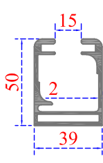
Sistem Kodu 41-2308 Ağırlık (kg/mt) 1,275
