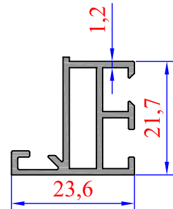
Sistem Kodu 50-1618 Ağırlık (kg/mt) 0,320
