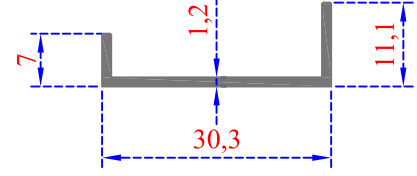
Sistem Kodu 24-312 Ağırlık (kg/mt) 0,150
