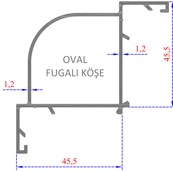
Sistem Kodu 34-1051 Ağırlık (kg/mt) 0,770
