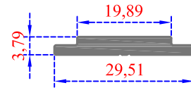
Sistem Kodu: 54-4807 Ağırlık (kg/mt) 0,260
