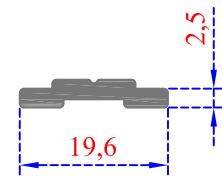
Sistem Kodu 49-4421 Ağırlık (kg/mt) 0,145
