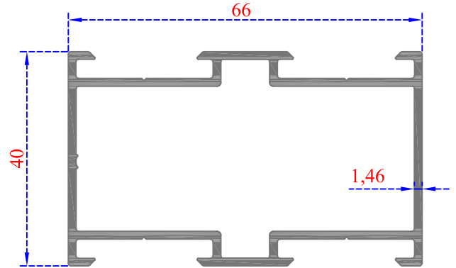
Sistem Kodu 54-4743
