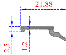
Sistem Kodu 54-4822 Ağırlık (kg/mt) 0,105
