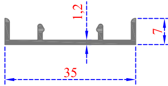
Sistem Kodu 38-1204 Ağırlık (kg/mt) 0,180
