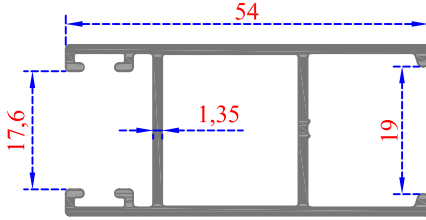
Sistem Kodu 54-4732 Ağırlık (kg/mt) 0,610
