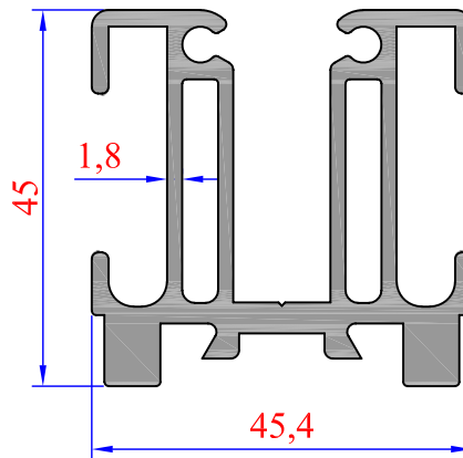
Sistem Kodu 50-1466 Ağırlık (kg/mt) 1,670
