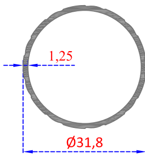
Sistem Kodu 80-5026 Ağırlık (kg/mt) 0,315
