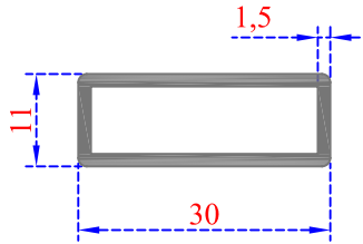
Sistem Kodu 20-117 Ağırlık (kg/mt) 0,315
