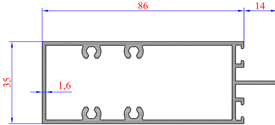
Sistem Kodu 50-1656 Ağırlık (kg/mt) 1,450
