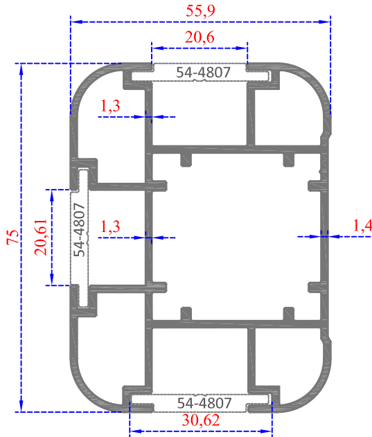
Sistem Kodu: 54-4806 Ağırlık (kg/mt) 1,685
