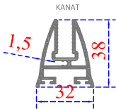
Sistem Kodu 41-2316 Ağırlık (kg/mt) 0,750
