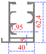
Sistem Kodu 41-2785 Ağırlık (kg/mt) 1,450
