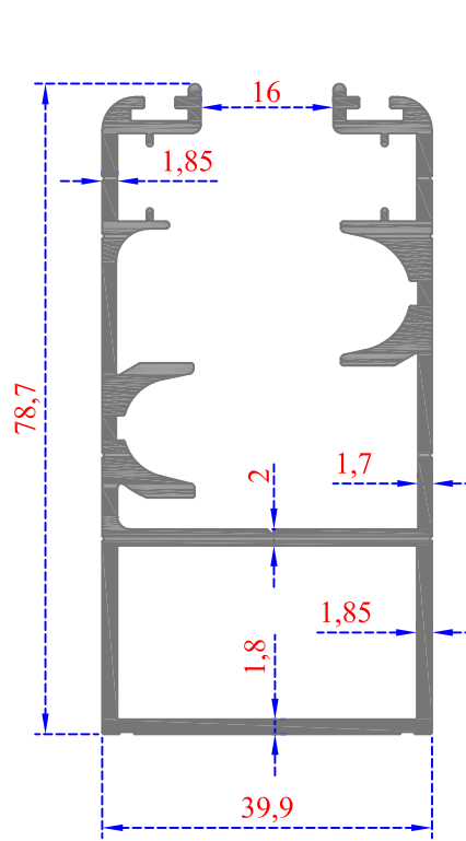
Sistem Kodu 41-2765 Ağırlık (kg/mt) 1,615
