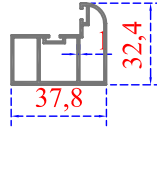
Sistem Kodu 41-2715 Ağırlık (kg/mt) 0,500
