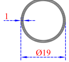
Sistem Kodu 22-257 Ağırlık (kg/mt) 0,155
