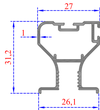
SÜRME DOLAP
