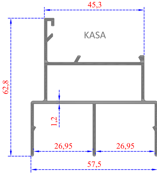
Sistem Kodu 45-1431 Ağırlık (kg/mt) 0,805
