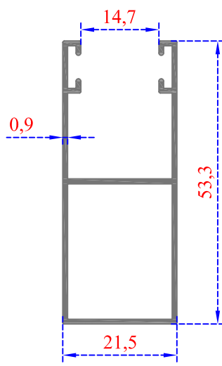
Sistem Kodu 38-1218 Ağırlık (kg/mt) 0,405
