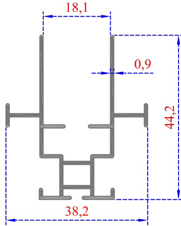
Sistem Kodu 40-1322 Ağırlık (kg/mt) 0,332
