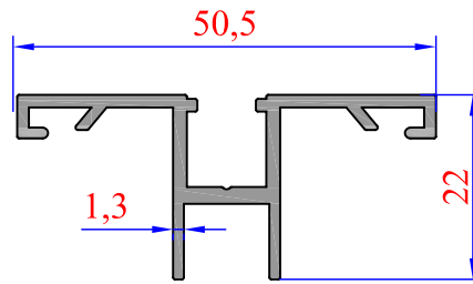
Sistem Kodu 50-1605 Ağırlık (kg/mt) 0,462
