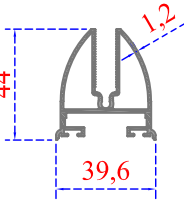
Sistem Kodu 41-2714 Ağırlık (kg/mt) 0,972
