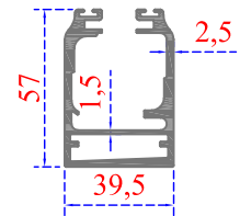
Sistem Kodu 41-2315 Ağırlık (kg/mt) 1,555
