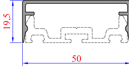
Sistem Kodu 50-1453 Ağırlık (kg/mt) 0,360
