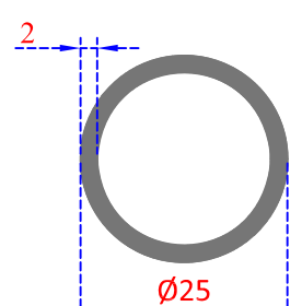
Sistem Kodu 22-263 Ağırlık (kg/mt) 0,392
