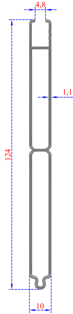
Sistem Kodu 49-4356 Ağırlık (kg/mt) 0,800
