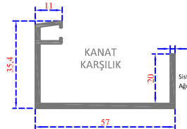
Sistem Kodu 41-2325 Ağırlık (kg/mt) 0,416
