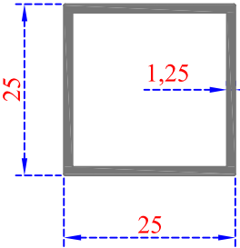
Sistem Kodu 20-126 Ağırlık (kg/mt) 0,325
