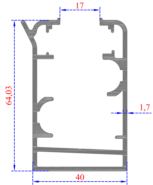
Sistem Kodu 41-2956 Ağırlık (kg/mt) 1,340
