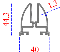
Sistem Kodu 41-2391-P Ağırlık (kg/mt) 0,920
