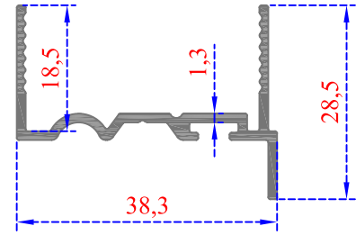
Sistem Kodu 41-2880 Ağırlık (kg/mt) 0,325
