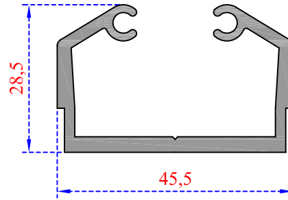
Sistem Kodu 50-1460 Ağırlık (kg/mt) 0,845
