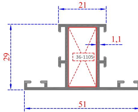
ORTA KAYIT
