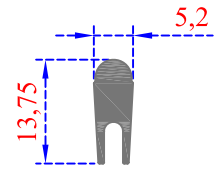
Sistem Kodu 46-2406 Ağırlık (kg/mt) 0,135
