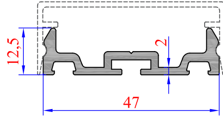
ALT ADAPTÖR
