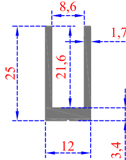
SÜRME - U -
