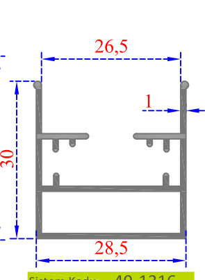
Sistem Kodu 40-1316 Ağırlık (kg/mt) 0,390
