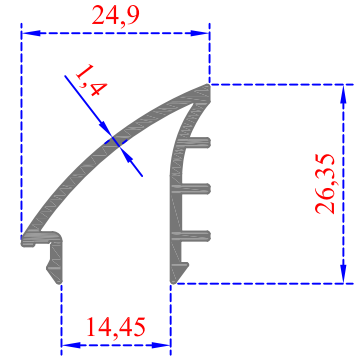
Sistem Kodu 58-2286 Ağırlık (kg/mt) 0,290
