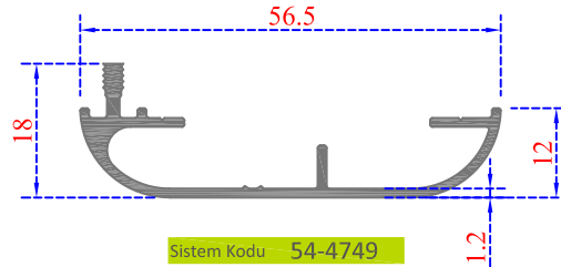
Sistem Kodu 54-4749 Ağırlık (kg/mt) 0,376
