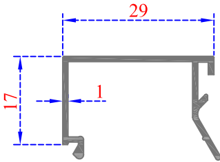
Sistem Kodu 34-1052 Ağırlık (kg/mt) 0,215
