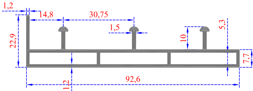
Sistem Kodu 41-2869 Ağırlık (kg/mt) 0,875
