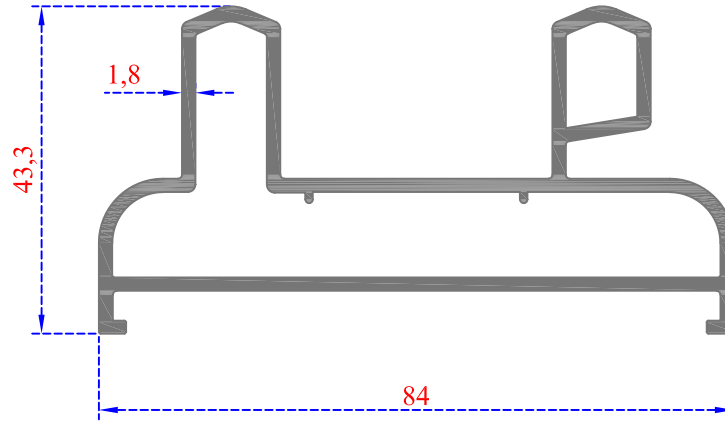
Sistem Kodu 49-4376 Ağırlık (kg/mt) 1,445
