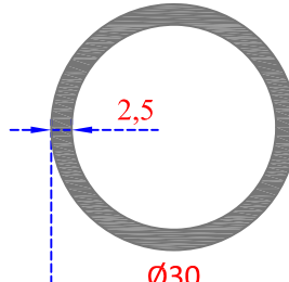
Sistem Kodu 22-201 Ağırlık (kg/mt) 0,586
