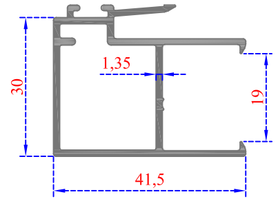
Sistem Kodu 54-4737 Ağırlık (kg/mt) 0,582
