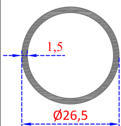
Sistem Kodu 22-217 Ağırlık (kg/mt) 0,330
