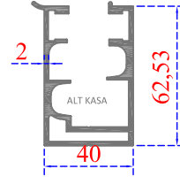
Sistem Kodu 41-2721 Ağırlık (kg/mt) 1,530
