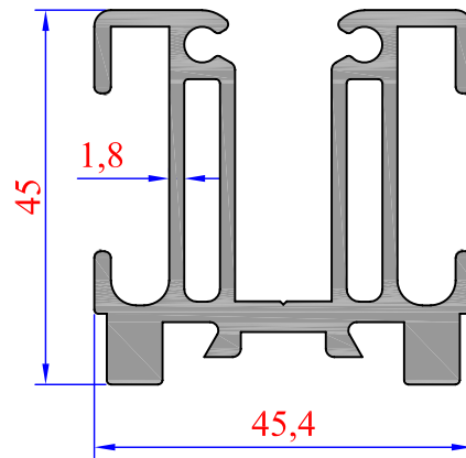
Sistem Kodu 50-1466 Ağırlık (kg/mt) 1,670
