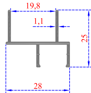
KAPI KARŞILIĞI
