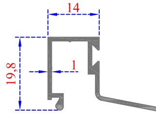
Sistem Kodu 34-1053 Ağırlık (kg/mt) 0,220
