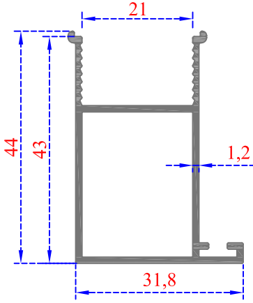
Sistem Kodu 41-2871 Ağırlık (kg/mt) 0,465
