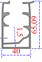
Sistem Kodu 41-2472 Ağırlık (kg/mt) 1,415
