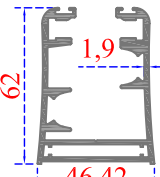
Sistem Kodu 41-2309 Ağırlık (kg/mt) 1,605
