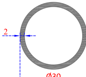
Sistem Kodu 22-200 Ağırlık (kg/mt) 0,480
