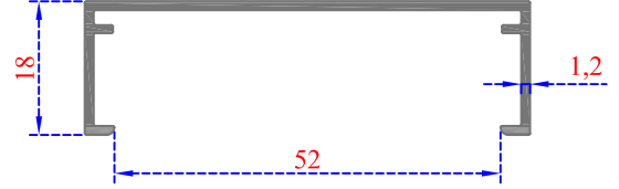
Sistem Kodu 50-1623 Ağırlık (kg/mt) 0,340
