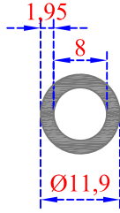
Sistem Kodu 22-239 Ağırlık (kg/mt) 0,166
