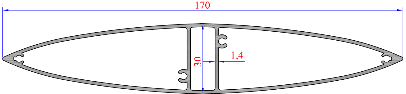
GÜNEŞ KIRICI
