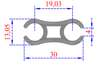
Sistem Kodu 57-2526 Ağırlık (kg/mt) 0,420
