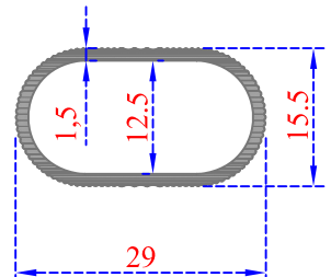
Sistem Kodu 22-231 Ağırlık (kg/mt) 0,290
