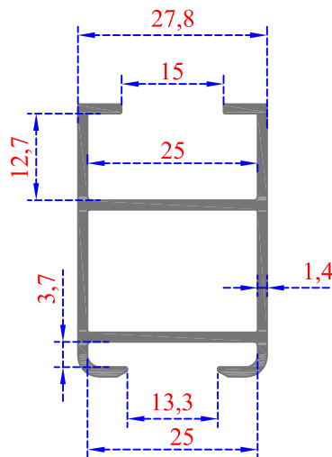
Sistem Kodu 39-1322 Ağırlık (kg/mt) 0,570
