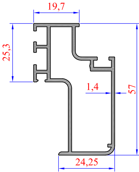
Sistem Kodu 50-1494 Ağırlık (kg/mt) 0,780
