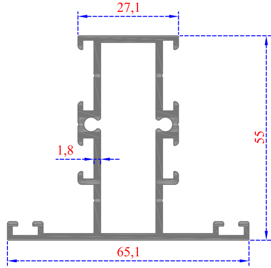
ORTA KAYIT
