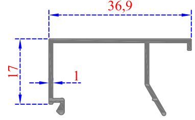
Sistem Kodu 34-1072 Ağırlık (kg/mt) 0,225
