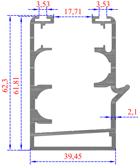
Sistem Kodu 41-2936 Ağırlık (kg/mt) 1,335
