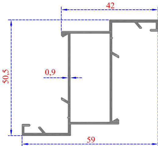
KANAT
