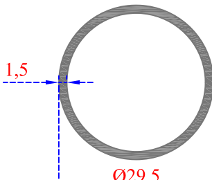
Sistem Kodu 22-230 Ağırlık (kg/mt) 0,360
