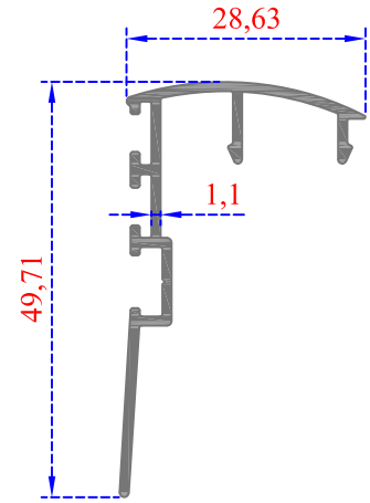
Sistem Kodu 49-4471 Ağırlık (kg/mt) 0.330
