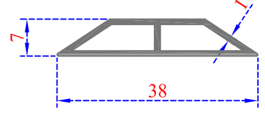
Sistem Kodu 80-5042 Ağırlık (kg/mt) 0,220
