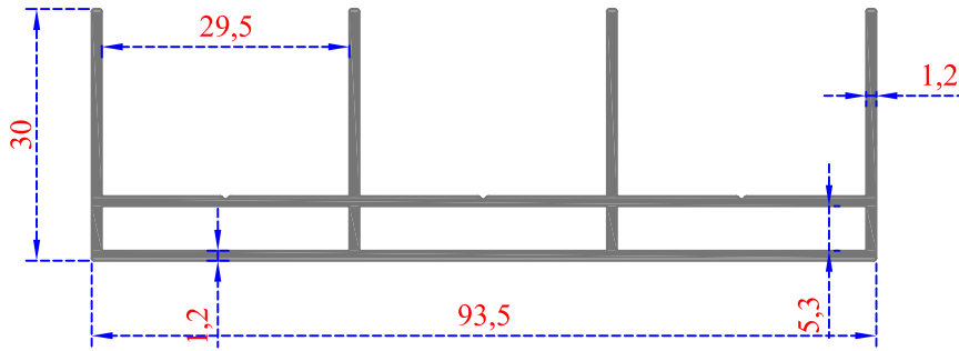
Sistem Kodu 41-2867 Ağırlık (kg/mt) 0,970
