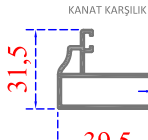
Sistem Kodu 41-2317 Ağırlık (kg/mt) 0,555
