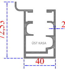
Sistem Kodu 41-2720 Ağırlık (kg/mt) 1,572
