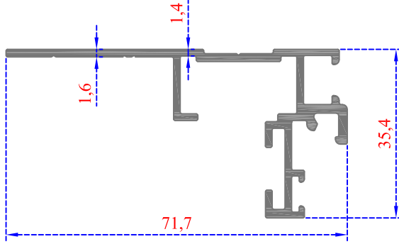
Sistem Kodu: 54-4833 Ağırlık (kg/mt) 0,720
