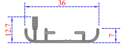
Sistem Kodu 54-4742 Ağırlık (kg/mt) 0,250
