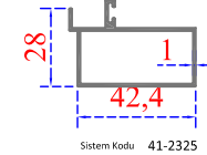
Sistem Kodu 41-2325 Ağırlık (kg/mt) 0,416
