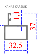
Sistem Kodu 41-2303 Ağırlık (kg/mt) 0,385
