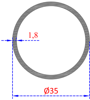
Sistem Kodu 22-234 Ağırlık (kg/mt) 0,510
