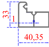
Sistem Kodu 41-2392-P Ağırlık (kg/mt) 0,441
