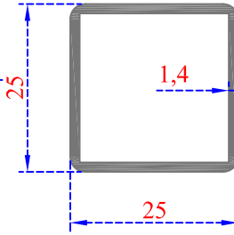
Sistem Kodu 20-131 Ağırlık (kg/mt) 0,350
