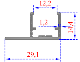
Sistem Kodu 54-4815 Ağırlık (kg/mt) 0,210
