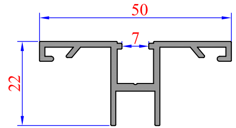
Sistem Kodu 50-1605 Ağırlık (kg/mt) 0,462
