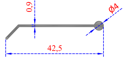
MENFEZ KANAT
