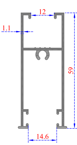
Sistem Kodu 54-4770 Ağırlık (kg/mt) 0,540
