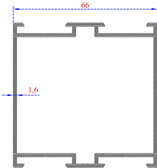
Sistem Kodu 54-4704
