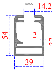
Sistem Kodu 41-2301 Ağırlık (kg/mt) 1,346
