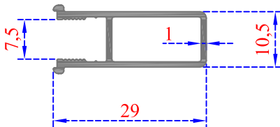
ÇERÇEVE DİKME
