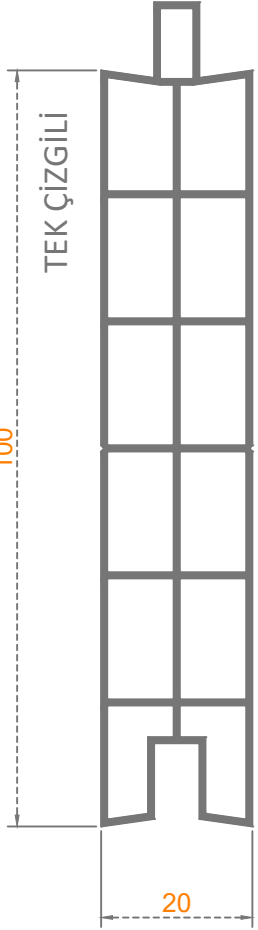
TEK ÇİZGİLİ ÇİFT ODACIKLI 10'LUK KAPI LAMBRI
