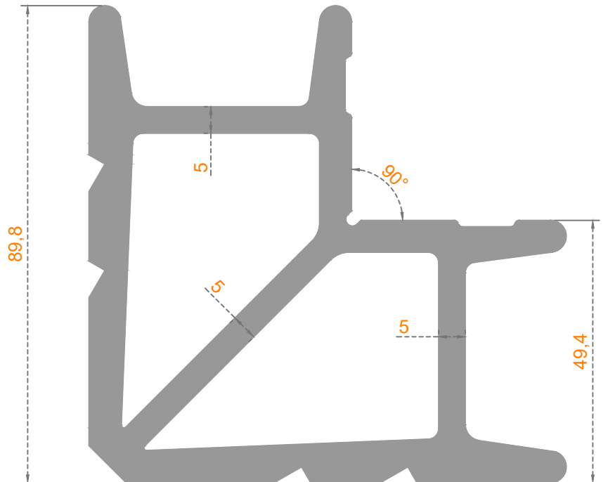
Sistem Kodu: 70-3059 Ağırlık (kg/mt) 6,240
