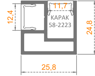
Sistem Kodu: 58-2223 Ağırlık (kg/mt) 0,395
