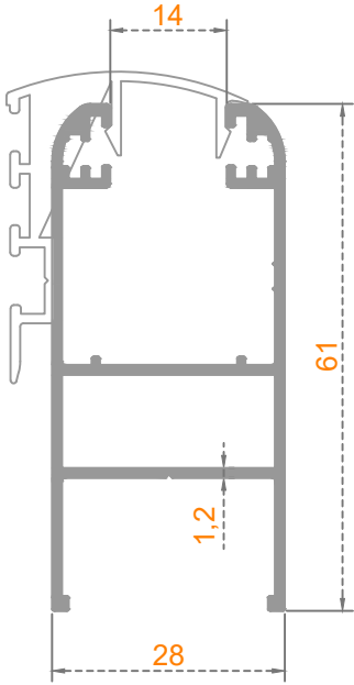
Sistem Kodu: 49-4351 Ağırlık (kg/mt) 0,695
