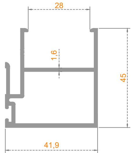
Sistem Kodu: 54-4821 Ağırlık (kg/mt) 0,860
