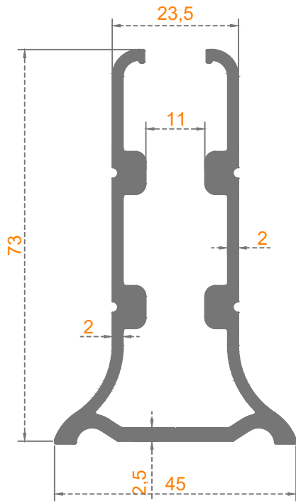
Sistem Kodu: 58-2311 Ağırlık (kg/mt) 1,490
