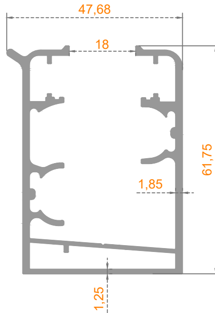
Sistem Kodu: 41-2945 Ağırlık (kg/mt) 1,250
