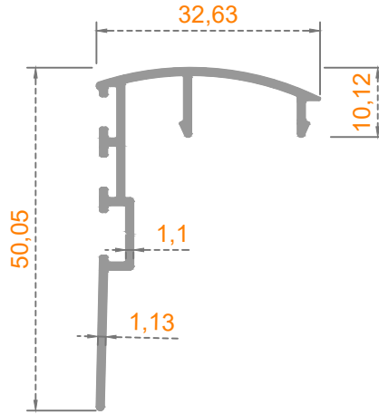
Sistem Kodu: 46-6021 Ağırlık (kg/mt) 0,342
