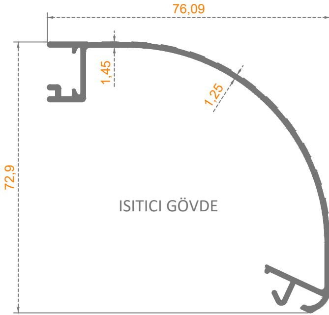
Sistem Kodu: 80-5007 Ağırlık (kg/mt) 0,685
