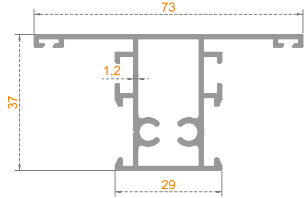
Sistem Kodu: 49-4409 Ağırlık (kg/mt) 0,840
