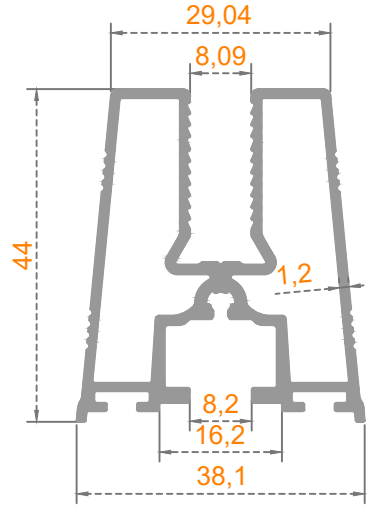
Profil Kodu: 41-2929 Ağırlık (kg/mt) 0,854
