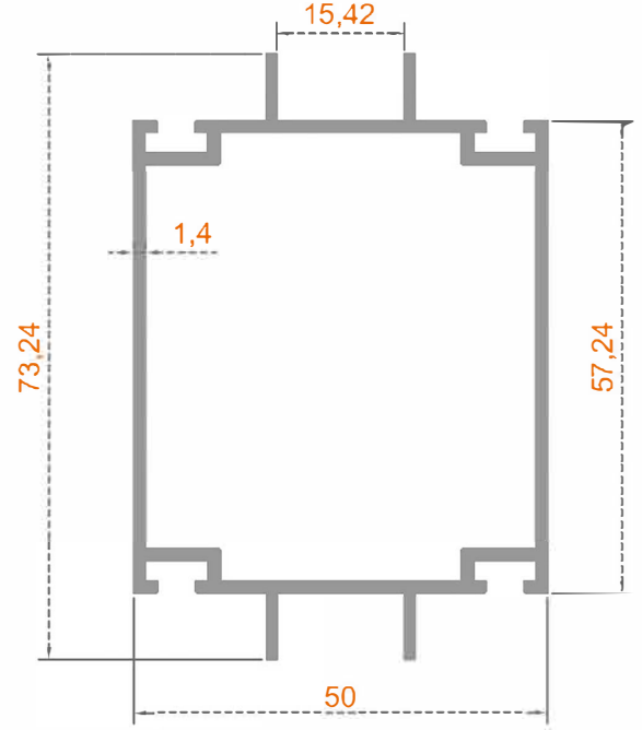
Sistem Kodu: 38-1241 Ağırlık (kg/mt) 1,005
