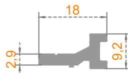
Sistem Kodu: 50-1620 Ağırlık (kg/mt) 0,195
