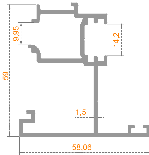
ÇİFT KANAT ADAPTÖRÜ (HAREKETLİ ORTA KAYIT)
