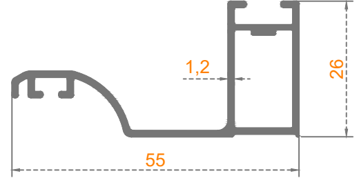
KÜÇÜK BAĞLI DİKME
