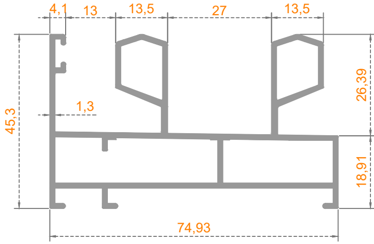
Profil Kodu: 47-4108 Ağırlık (kg/mt) 1,305
