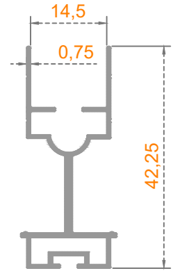
Sistem Kodu: 40-1328 Ağırlık (kg/mt) 0,295
