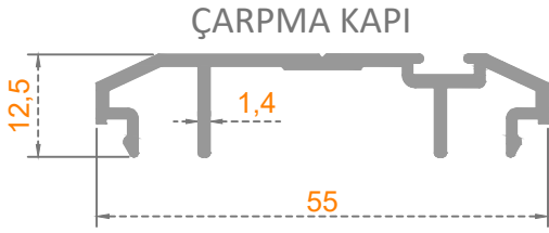
Sistem Kodu: 55-2119 Ağırlık (kg/mt) 0,410
