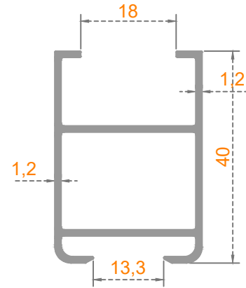
Sistem Kodu: 39-1313 Ağırlık (kg/mt) 0,485
