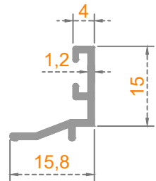
ISI CAM ÇITA
