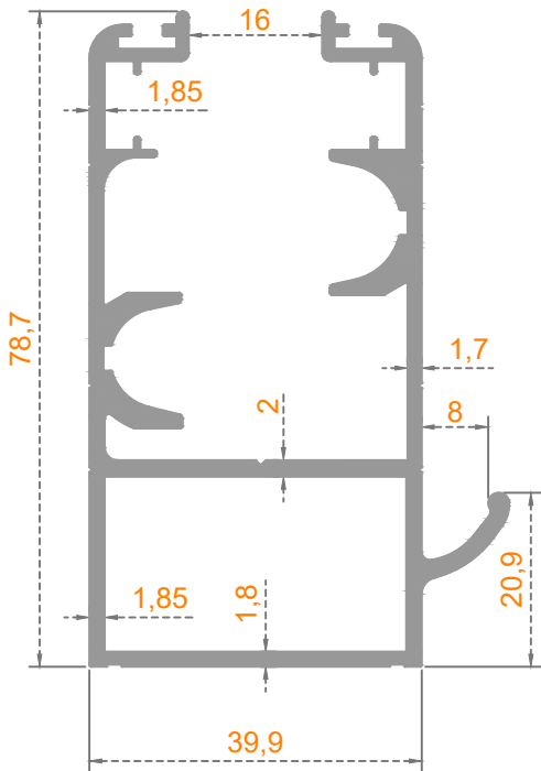
Sistem Kodu: 41-2964 Ağırlık (kg/mt) 1,690
