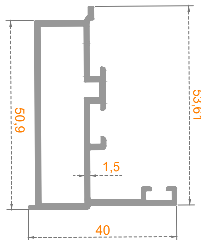
DIŞA AÇILIR KANAT ADAPTÖRÜ
