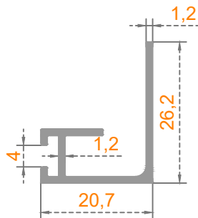
Sistem Kodu: 39-1319 Ağırlık (kg/mt) 0,230
