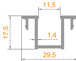
SÜRME TEK CAM ÇİTASI
