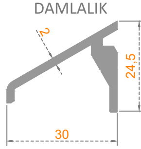
Sistem Kodu: 70-3024 Ağırlık (kg/mt) 0,400
