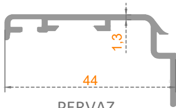
Sistem Kodu: 35-10836 Ağırlık (kg/mt) 0,300
