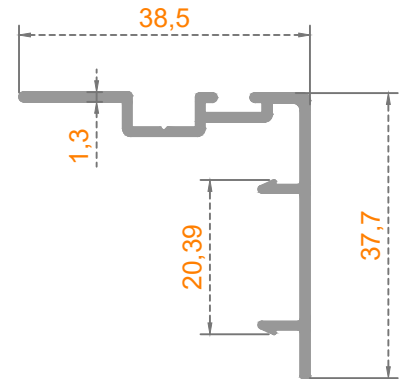
Profil Kodu: 47-4041 Ağırlık (kg/mt) 0,340
