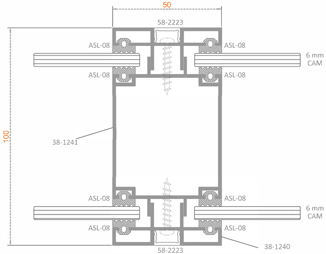
Sistem Kodu: 38-1272 Ağırlık (kg/mt) 1,010
