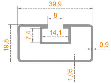
Sistem Kodu: 39-1327 Ağırlık (kg/mt) 0,376
