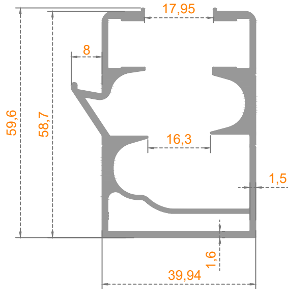
Profil Kodu: 41-2949 Ağırlık (kg/mt) 1,275
