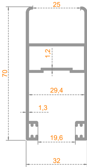
Profil Kodu: 47-4040 Ağırlık (kg/mt) 0,780
