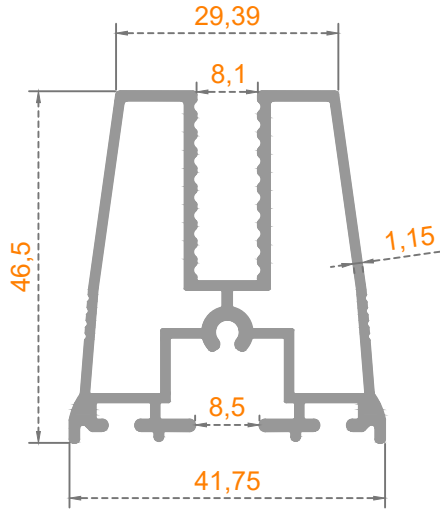
Profil Kodu: 41-2906 Ağırlık (kg/mt) 0,918
