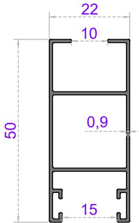
Sistem Kodu 49-4381 Ağırlık (kg/mt) 0,410
