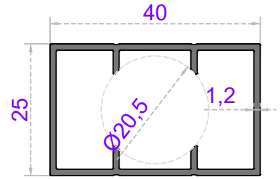
Sistem Kodu 58-2368 Ağırlık (kg/mt) 0,465
