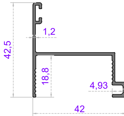
Sistem Kodu 41-2882 Ağırlık (kg/mt) 0,385
