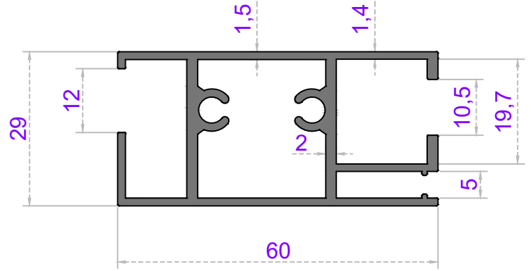
Sistem Kodu 39-1344 Ağırlık (kg/mt) 1,080
