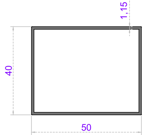
Sistem Kodu 20-228 Ağırlık (kg/mt) 0,556
