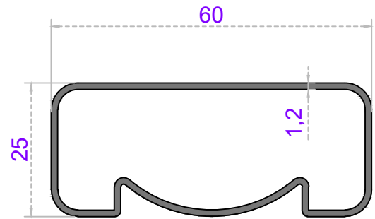
Sistem Kodu 58-2298 Ağırlık (kg/mt) 1,125
