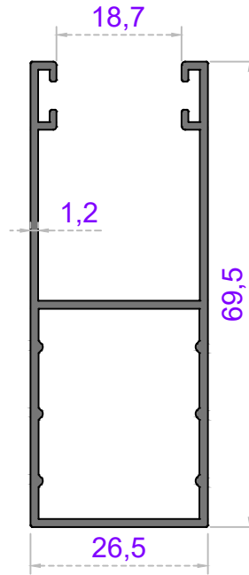
Sistem Kodu 38-1224 Ağırlık (kg/mt) 0,685
