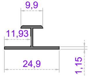
Sistem Kodu 39-1288 Ağırlık (kg/mt) 0,132
