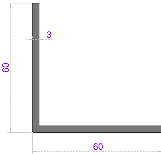
Sistem Kodu 24-314 Ağırlık (kg/mt) 0,955
