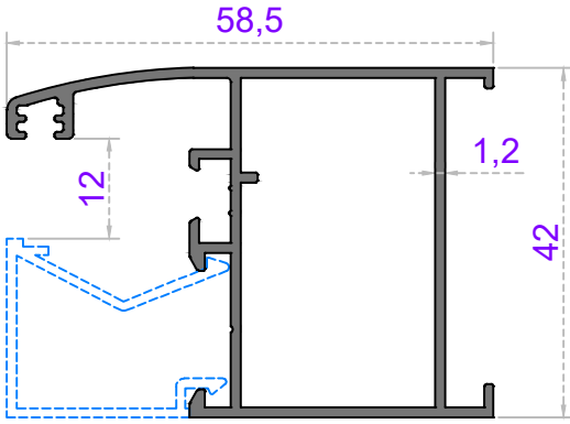
Sistem Kodu 49-4301 Ağırlık (kg/mt) 0,690
