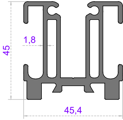
Sistem Kodu 50-1466 Ağırlık (kg/mt) 1,670
