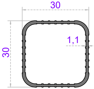
Sistem Kodu 20-191 Ağırlık (kg/mt) 0,370
