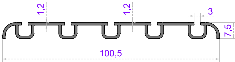
Sistem Kodu 41-2376 Ağırlık (kg/mt) 0,590
