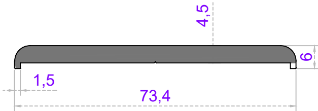
Sistem Kodu 58-2260 Ağırlık (kg/mt) 0,910
