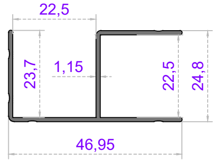
BAĞLI DİKME
