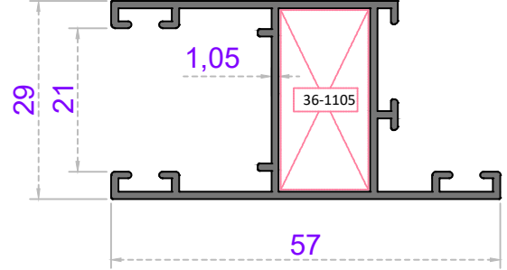
KANAT
