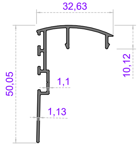
Sistem Kodu 46-6021 Ağırlık (kg/mt) 0,342
