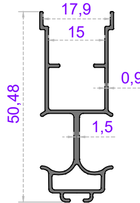
Sistem Kodu 40-1324 Ağırlık (kg/mt) 0,370
