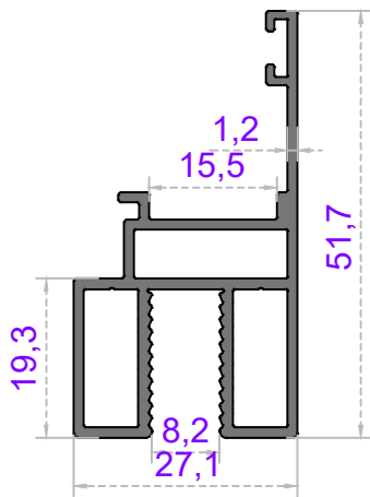
Sistem Kodu 41-2932 Ağırlık (kg/mt) 0,643
