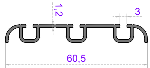
Sistem Kodu 41-2767 Ağırlık (kg/mt) 0,365
