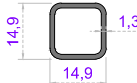
Sistem Kodu 58-2248 Ağırlık (kg/mt) 0,180
