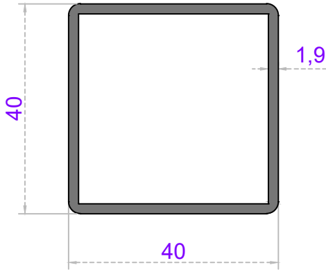
Sistem Kodu 20-134 Ağırlık (kg/mt) 0,773
