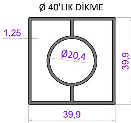
Sistem Kodu 58-2296 Ağırlık (kg/mt) 0,810
