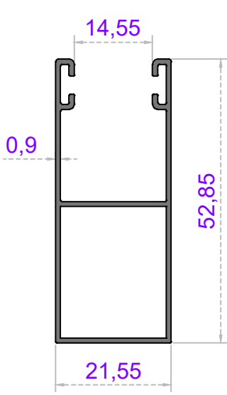
Sistem Kodu 38-1235 Ağırlık (kg/mt) 0,430
