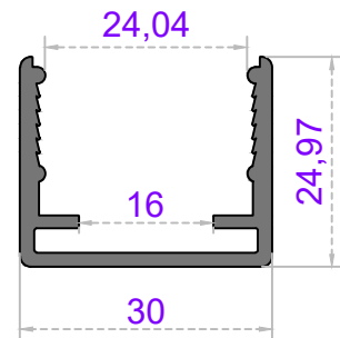
Sistem Kodu 58-2414 Ağırlık (kg/mt) 0,461
