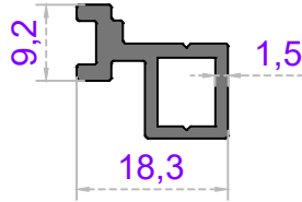
Sistem Kodu 50-1612 Ağırlık (kg/mt) 0,260
