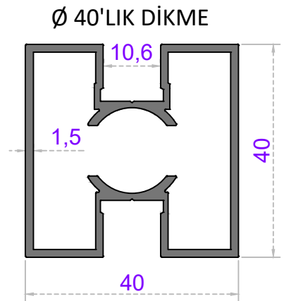
Sistem Kodu 58-2206 Ağırlık (kg/mt) 0,872
