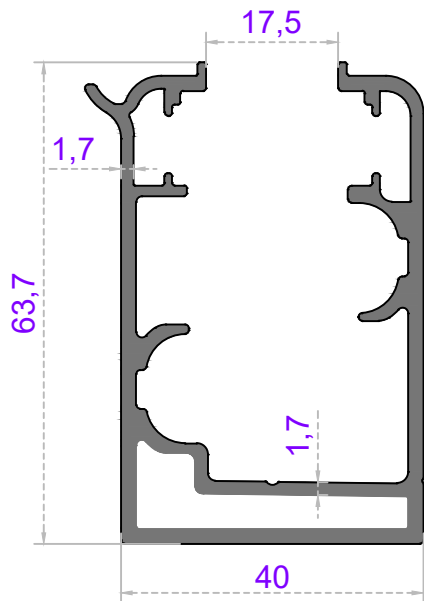
Sistem Kodu 41-2928 Ağırlık (kg/mt) 1,373
