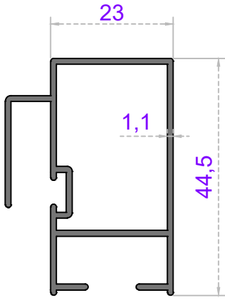
KANAT ORTA
