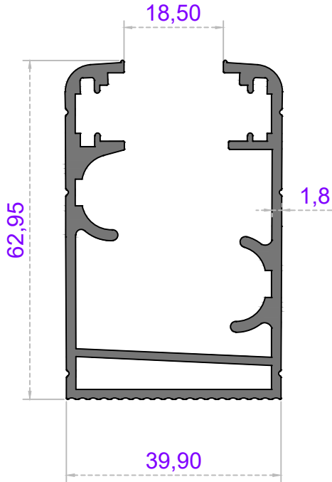
Sistem Kodu 41-2342 Ağırlık (kg/mt) 1,345
