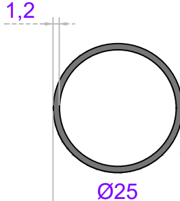
Sistem Kodu 22-262 Ağırlık (kg/mt) 0,245
