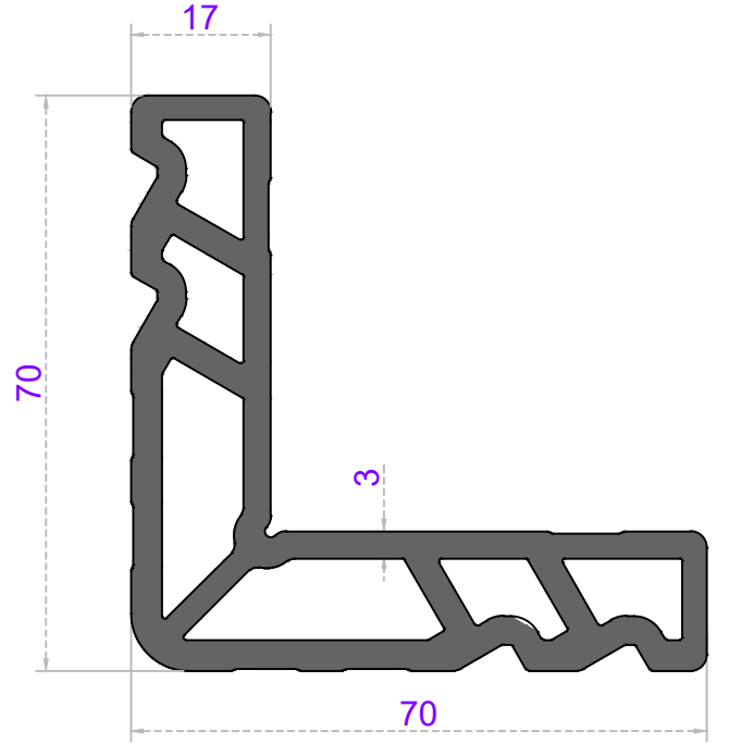
Sistem Kodu 70-3067 Ağırlık (kg/mt) 2,490
