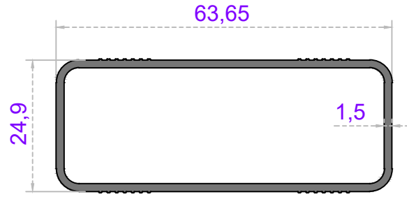
Sistem Kodu 20-189 Ağırlık (kg/mt) 0,685
