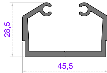
Sistem Kodu 50-1460 Ağırlık (kg/mt) 0,845
