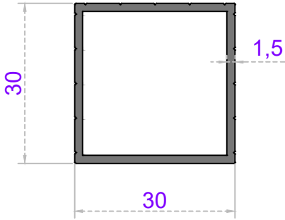
Sistem Kodu 20-127 Ağırlık (kg/mt) 0,465
