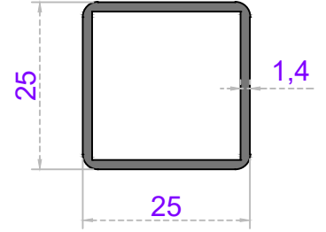
Sistem Kodu 20-131 Ağırlık (kg/mt) 0,350
