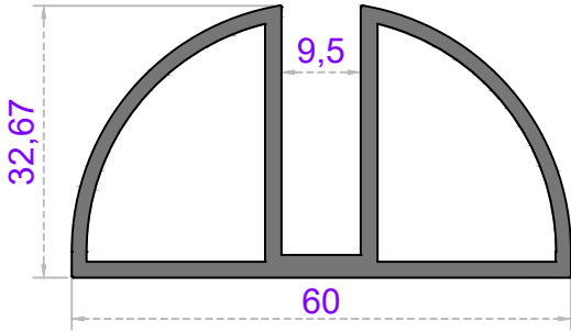
Ø60'LIK YARIM DİKME
