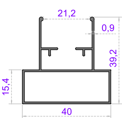
Sistem Kodu 40-1312-Ö Ağırlık (kg/mt) 0,435
