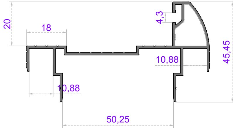
Sistem Kodu 39-1323 Ağırlık (kg/mt) 0,660
