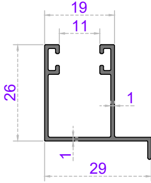
Sistem Kodu 58-2300 Ağırlık (kg/mt) 0,275
