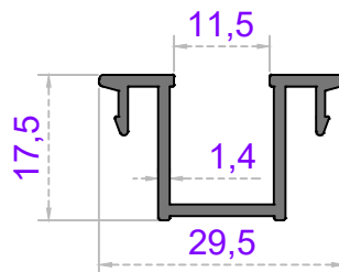
Sistem Kodu 47-4036 Ağırlık (kg/mt) 0,280
