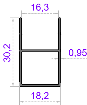
Sistem Kodu 40-1329 Ağırlık (kg/mt) 0,235
