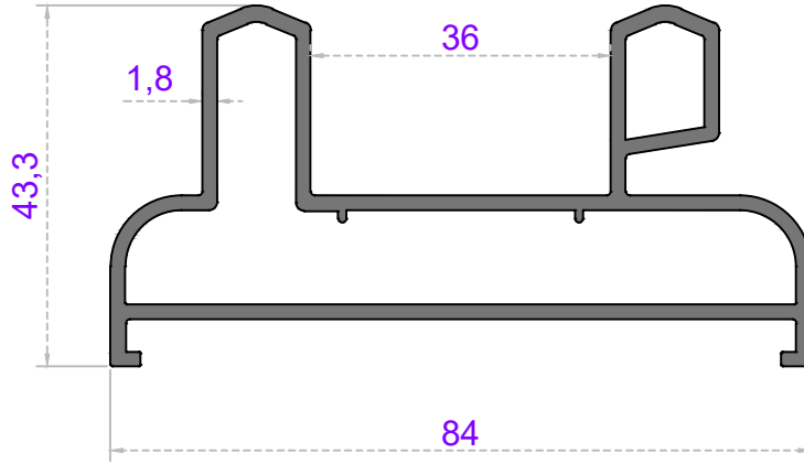
Sistem Kodu 49-4376 Ağırlık (kg/mt) 1,445
