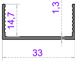
Sistem Kodu 41-2881 Ağırlık (kg/mt) 0,206
