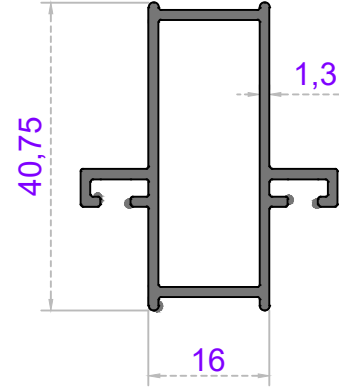
KİLİT PROFİLİ
