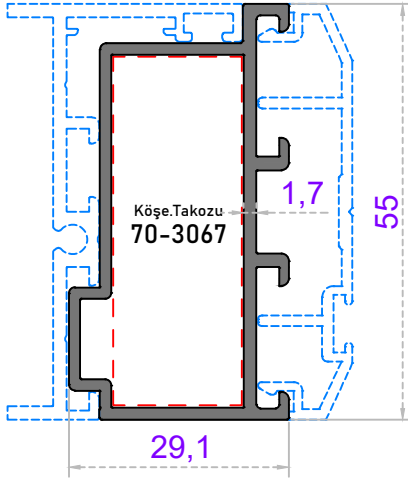
ÇARPMA KAPI DESTEK PRF
