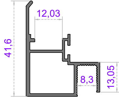
Sistem Kodu 80-5259 Ağırlık (kg/mt) 0,486
