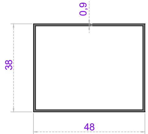
Sistem Kodu 20-113 Ağırlık (kg/mt) 0,415
