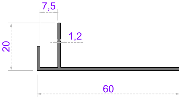
Sistem Kodu 26-415 Ağırlık (kg/mt) 0,290
