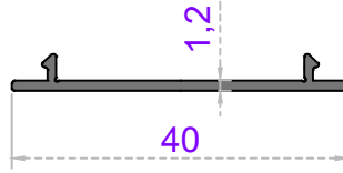
Sistem Kodu 50-1624 Ağırlık (kg/mt) 0,150
