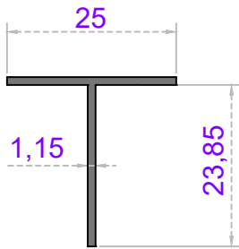
Sistem Kodu 26-400 Ağırlık (kg/mt) 0,155
