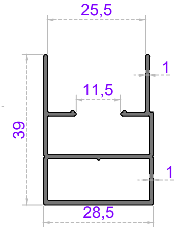
Sistem Kodu 40-1325 Ağırlık (kg/mt) 0,400
