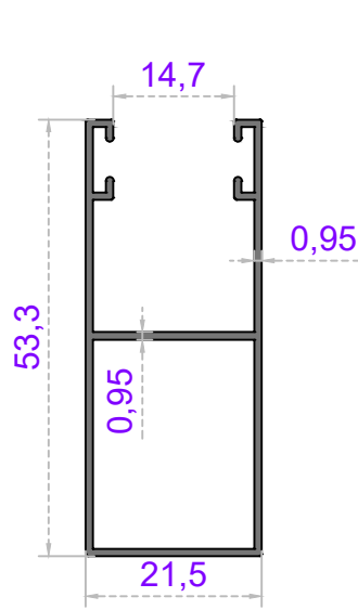
Sistem Kodu 38-1218 Ağırlık (kg/mt) 0,422
