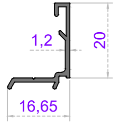
Sistem Kodu 47-4032 Ağırlık (kg/mt) 0,140
