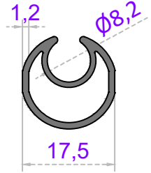
Sistem Kodu 57-2509 Ağırlık (kg/mt) 0,215
