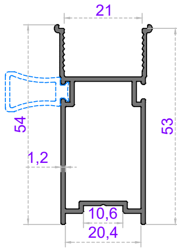
Sistem Kodu 41-2872 Ağırlık (kg/mt) 0,520
