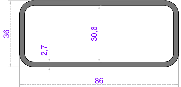
80 x 30 DİRSEK
