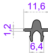
Sistem Kodu 64-1581 Ağırlık (kg/mt) 0,110
