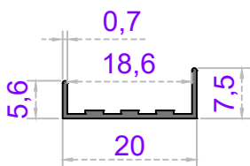
Sistem Kodu 48-4238 Ağırlık (kg/mt) 0,070
