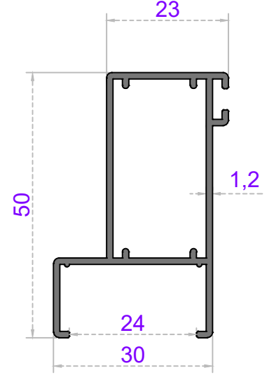
ISICAMLI KANAT YAN
