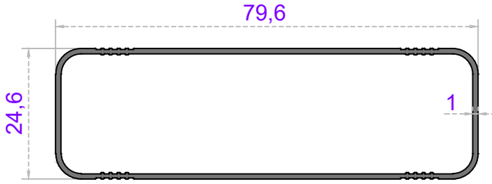
Sistem Kodu 20-188 Ağırlık (kg/mt) 0,545
