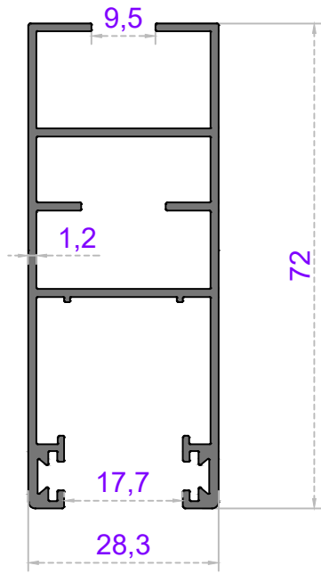
Sistem Kodu 53-4581 Ağırlık (kg/mt) 0,845
