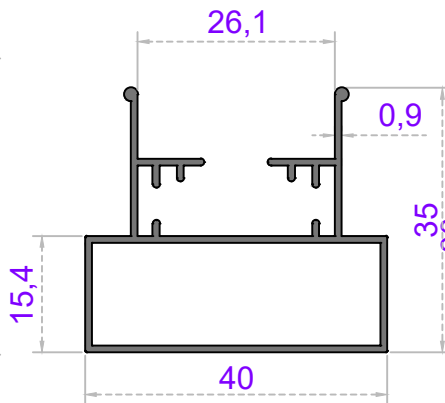
Sistem Kodu 40-1313-Ö Ağırlık (kg/mt) 0,440
