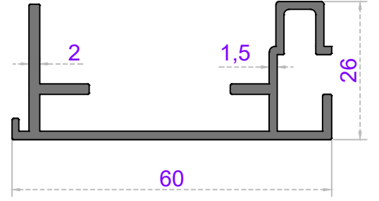
Sistem Kodu 56-1509 Ağırlık (kg/mt) 0,695
