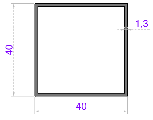
Sistem Kodu 20-226 Ağırlık (kg/mt) 0,550
