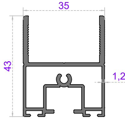
Sistem Kodu 41-2962 Ağırlık (kg/mt) 0,799
