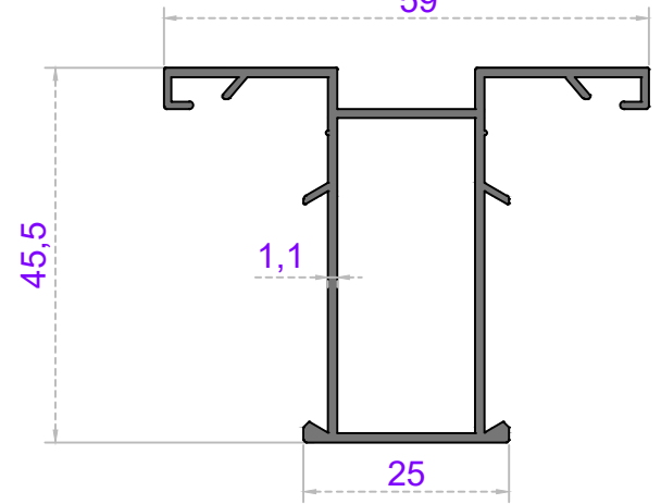
ORTA KAYIT
