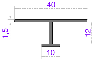
Sistem Kodu 26-411 Ağırlık (kg/mt) 0,270
