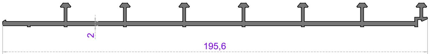
Sistem Kodu 50-1628 Ağırlık (kg/mt) 1,390
