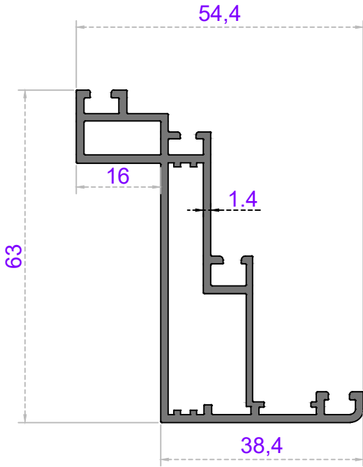
Sistem Kodu 50-1674 Ağırlık (kg/mt) 0,945
