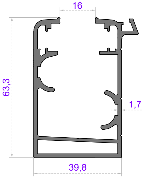
Sistem Kodu 41-2967 Ağırlık (kg/mt) 1,400
