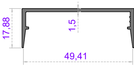
Sistem Kodu 54-4795 Ağırlık (kg/mt) 0,337
