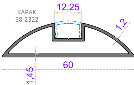
Sistem Kodu 58-2319 Ağırlık (kg/mt) 0,495
