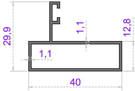
Sistem Kodu 41-2453 Ağırlık (kg/mt) 0,383
