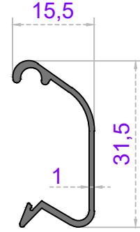
ÖZEL KASA ÇİTASI
