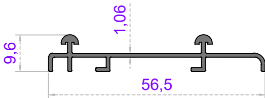
SÜRME DOLAP
