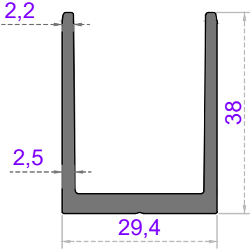
SİSTEM - U -
