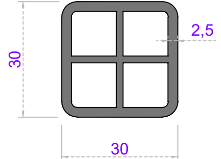
Sistem Kodu 20-154 Ağırlık (kg/mt) 0,945
