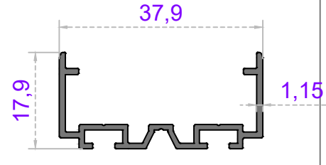
Sistem Kodu 41-2961 Ağırlık (kg/mt) 0,290
