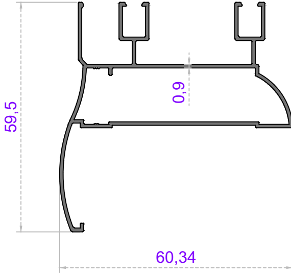
Sistem Kodu 49-4379 Ağırlık (kg/mt) 0,630
