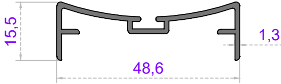
ÇARPMA KAPI İÇ
