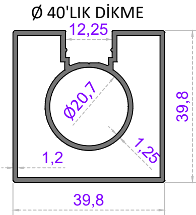
Sistem Kodu 58-2222 Ağırlık (kg/mt) 0,770
