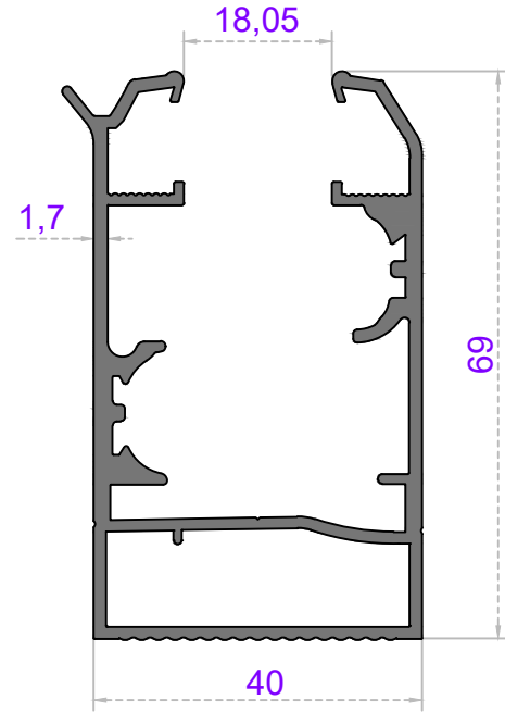
Sistem Kodu 41-2966 Ağırlık (kg/mt) 1,316
