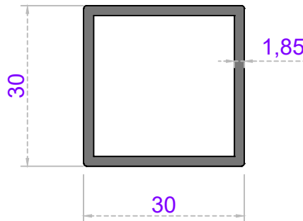
Sistem Kodu 20-149 Ağırlık (kg/mt) 0,565
