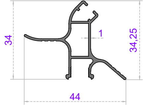
KÖŞE GİRİŞ KANAT ÇEKME
