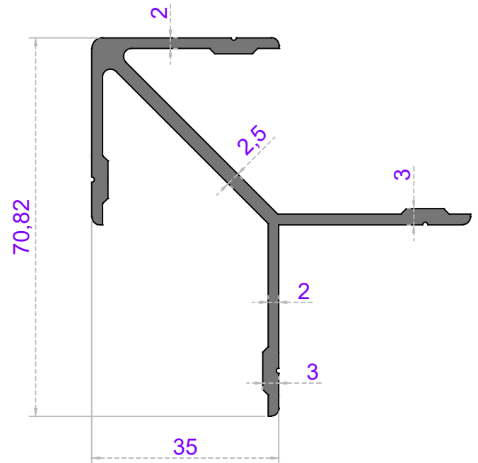
C-60 ÇAVUŞ
