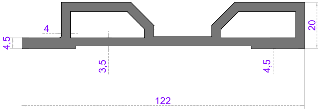
İSKELE PROFİLLER
