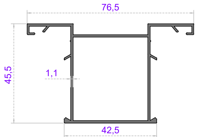
ORTA KAYIT
