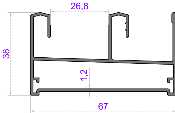
Sistem Kodu 49-4355 Ağırlık (kg/mt) 0,955
