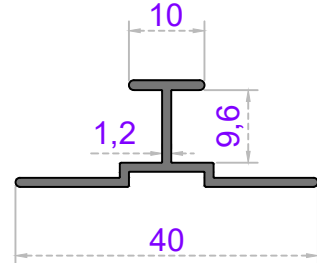
Sistem Kodu 26-419 Ağırlık (kg/mt) 0,220
