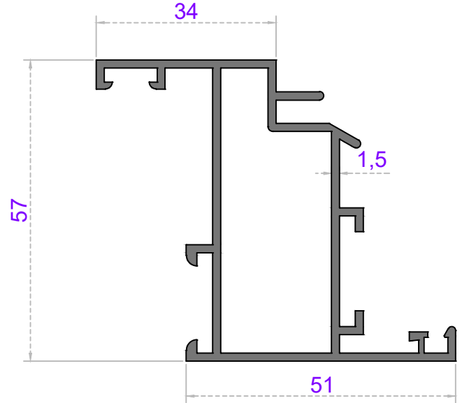
KANAT
