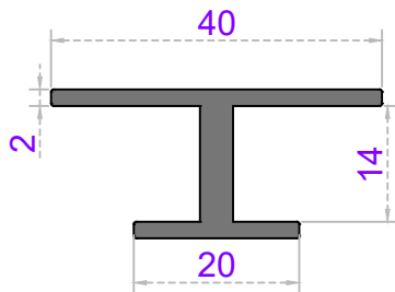
Sistem Kodu 26-408 Ağırlık (kg/mt) 0,480
