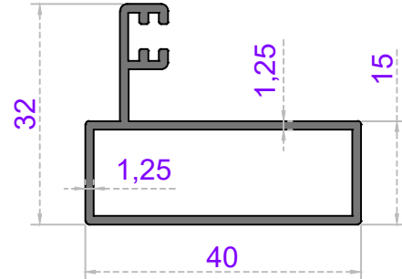
Sistem Kodu 41-2351 Ağırlık (kg/mt) 0,473
