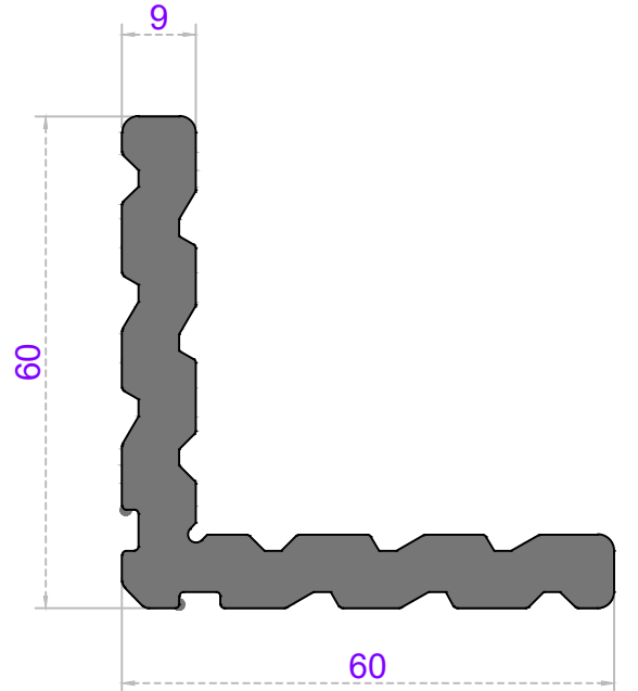
Sistem Kodu 50-1471 Ağırlık (kg/mt) 2,350
