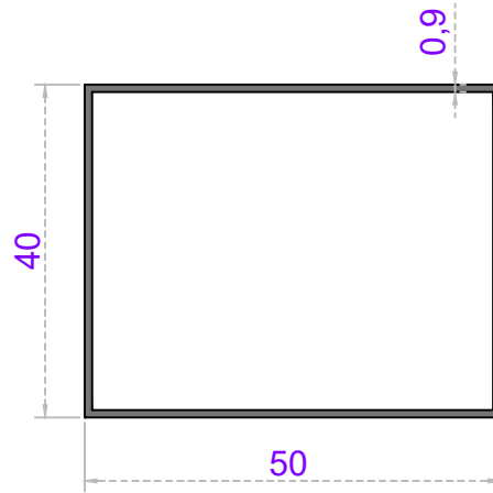
Sistem Kodu 20-104 Ağırlık (kg/mt) 0,440
