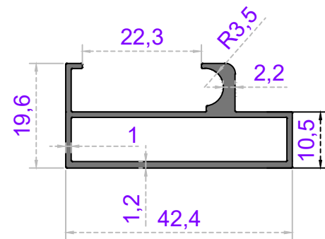
Sistem Kodu 65-1920 Ağırlık (kg/mt) 0,415
