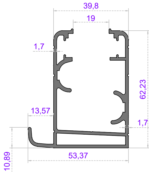
Sistem Kodu 41-2841 Ağırlık (kg/mt) 1,345
