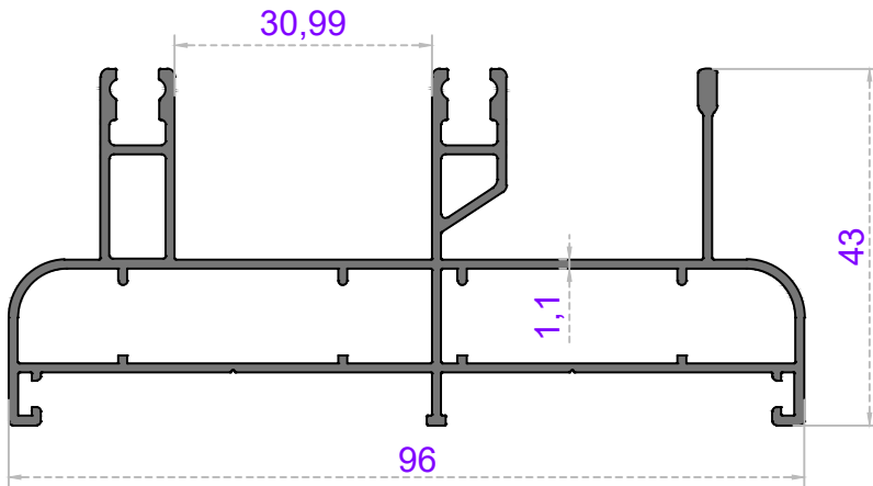
Sistem Kodu 49-4427 Ağırlık (kg/mt) 1,230
