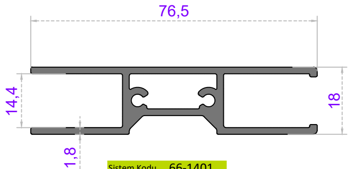
Sistem Kodu 66-1401 Ağırlık (kg/mt) 1,014
