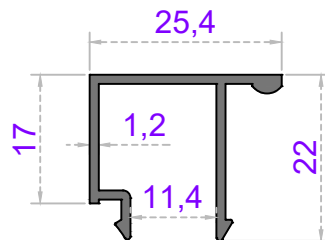
Sistem Kodu 60-1658 Ağırlık (kg/mt) 0,246
