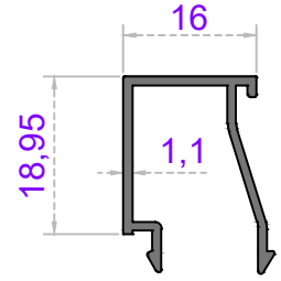
ISICAM ÇİTASI
