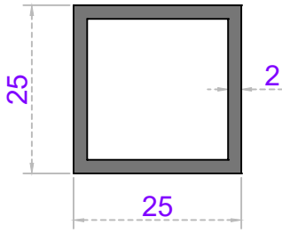
Sistem Kodu 20-110 Ağırlık (kg/mt) 0,500
