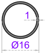
Sistem Kodu 22-258 Ağırlık (kg/mt) 0,130
