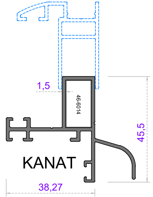
Sistem Kodu 50-11003 Ağırlık (kg/mt) 0,716
