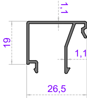
24 mm ISICAM ÇITA
