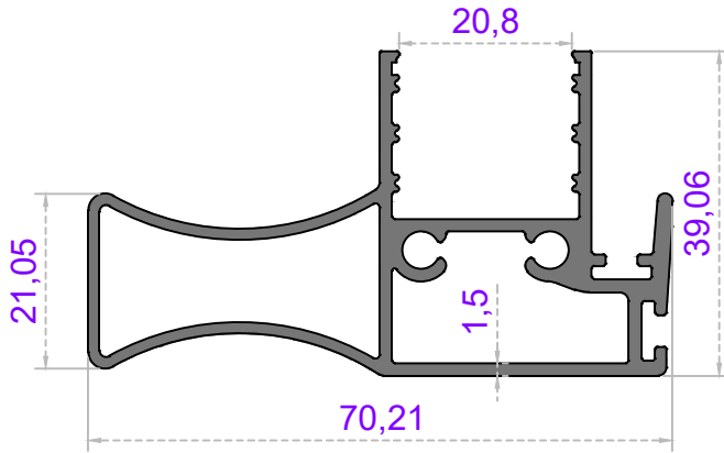
Sistem Kodu 59-7007 Ağırlık (kg/mt) 1,139
