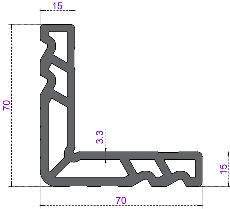
S.ÇERÇEVE TAKOZU
