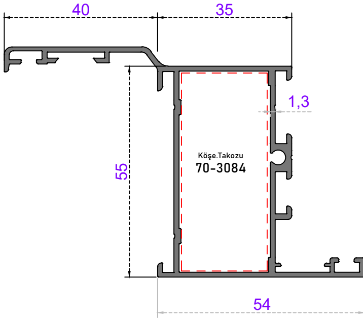
Sistem Kodu 55-2136 Ağırlık (kg/mt) 1,080
