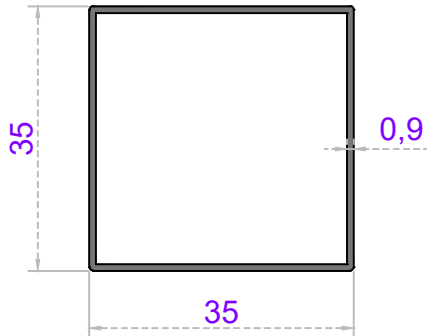
Sistem Kodu 20-153 Ağırlık (kg/mt) 0,335
