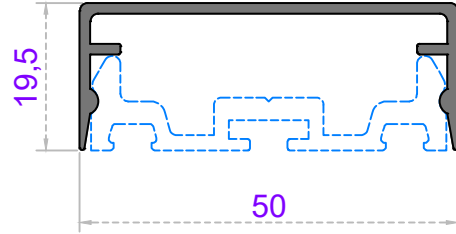
Sistem Kodu 50-1453 Ağırlık (kg/mt) 0,364
