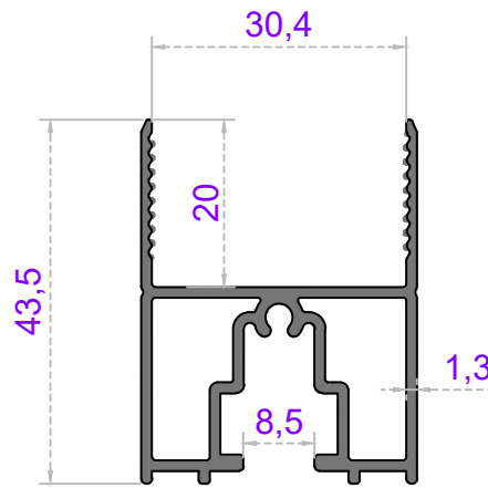
Sistem Kodu 41-2879 Ağırlık (kg/mt) 0,679
