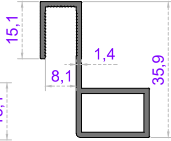
Sistem Kodu 41-2799 Ağırlık (kg/mt) 0,391
