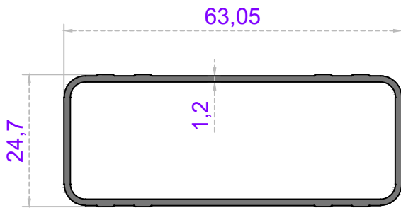
Sistem Kodu 20-201 Ağırlık (kg/mt) 0,550
