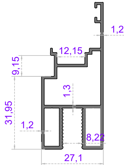
Sistem Kodu 41-2933 Ağırlık (kg/mt) 0,755
