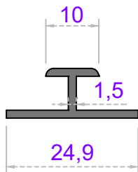
Sistem Kodu 39-1287 Ağırlık (kg/mt) 0,167
