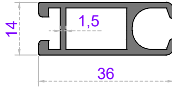
Sistem Kodu 48-4226 Ağırlık (kg/mt) 0,465
