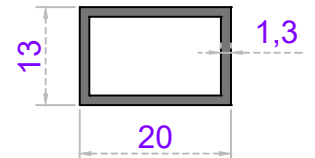
Sistem Kodu 20-116 Ağırlık (kg/mt) 0,215
