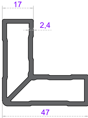
Sistem Kodu 36-1114 Ağırlık (kg/mt) 1,275
