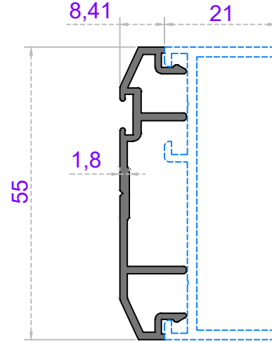
ÇARPMA KAPI ADAPTÖRÜ
