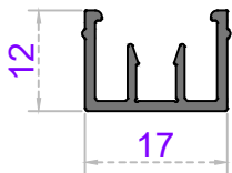
Sistem Kodu 50-1626 Ağırlık (kg/mt) 0,168
