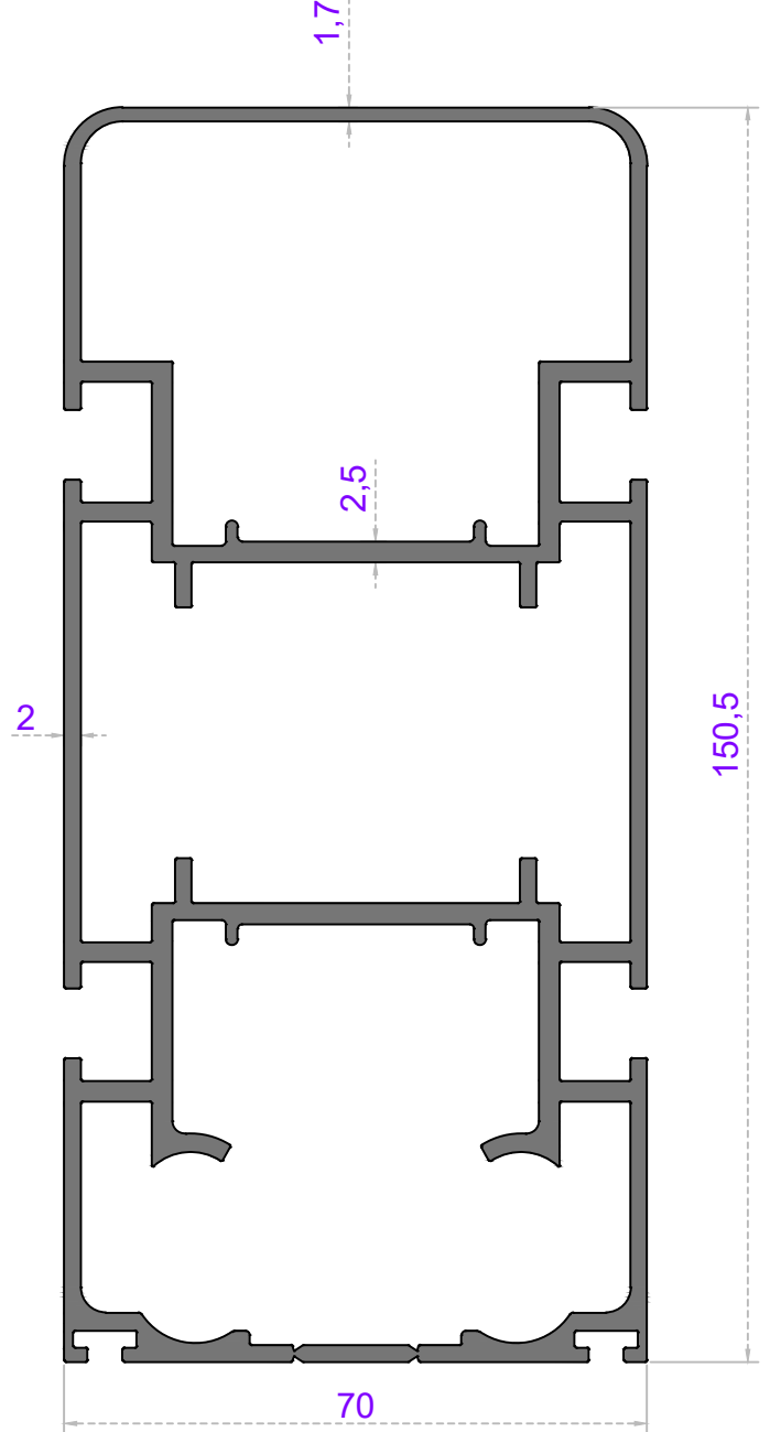
Sistem Kodu 57-2555 Ağırlık (kg/mt) 4,195
