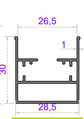
Sistem Kodu 40-1316 Ağırlık (kg/mt) 0,390
