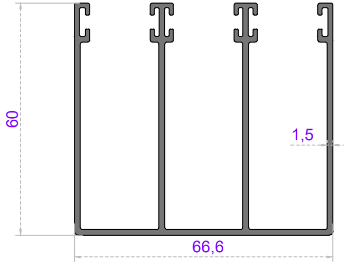
Sistem Kodu 66-1432 Ağırlık (kg/mt) 1,380
