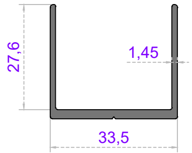
GENİŞ - U - (IRAK İÇİN)
