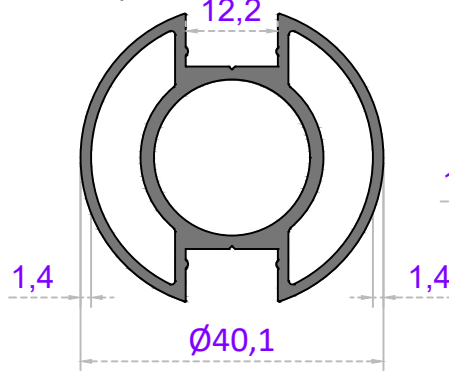
Ø 40'LIK DİKME
