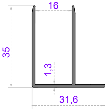
Sistem Kodu 66-1309 Ağırlık (kg/mt) 0,350
