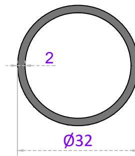
Sistem Kodu 22-201 Ağırlık (kg/mt) 0,586
