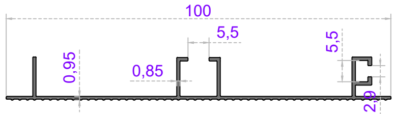
Sistem Kodu 48-4263 Ağırlık (kg/mt) 0,345
