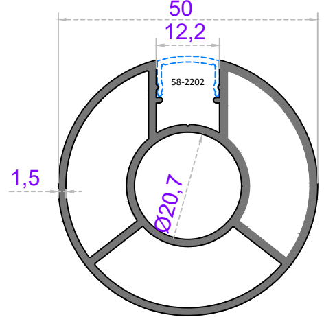
Ø 50'LUK DİKME
