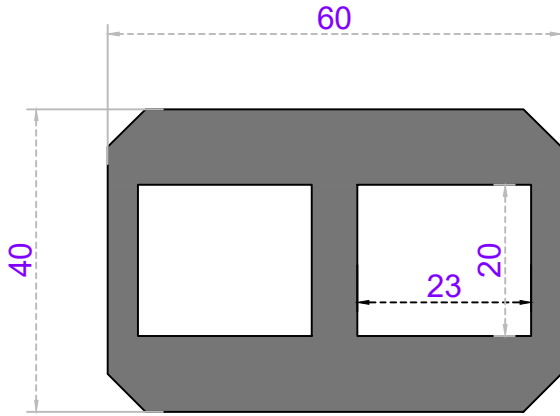
Sistem Kodu 58-2411 Ağırlık (kg/mt) 3,895
