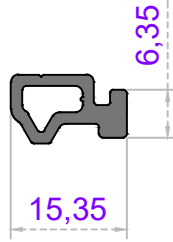
Sistem Kodu 50-1489 Ağırlık (kg/mt) 0,190
