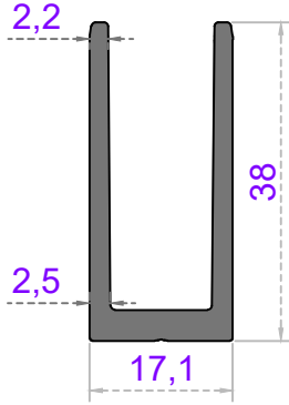
SÜRME - U -
