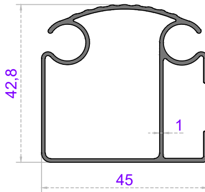
Sistem Kodu 57-2515 Ağırlık (kg/mt) 0,600
