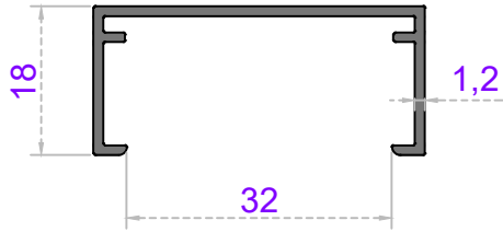
Sistem Kodu 50-1622 Ağırlık (kg/mt) 0,275
