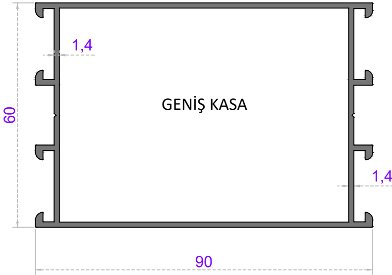
Sistem Kodu 62-1704 Ağırlık (kg/mt) 1,295
