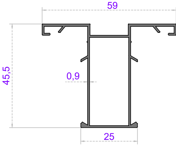
ORTA KAYIT
