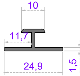
Sistem Kodu 39-1287 Ağırlık (kg/mt) 0,167
