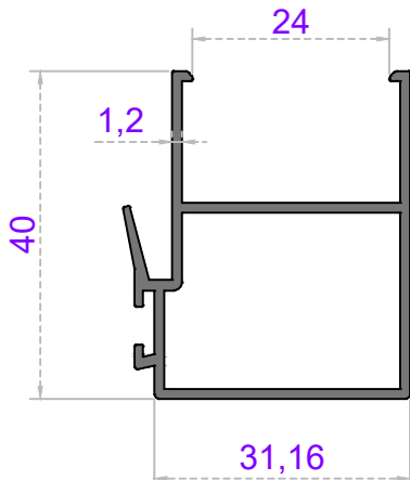
Sistem Kodu 49-4392 Ağırlık (kg/mt) 0,512
