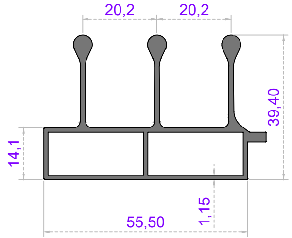
Sistem Kodu 41-2768 Ağırlık (kg/mt) 0,945
