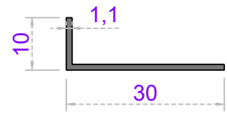
Sistem Kodu 24-322 Ağırlık (kg/mt) 0,116
