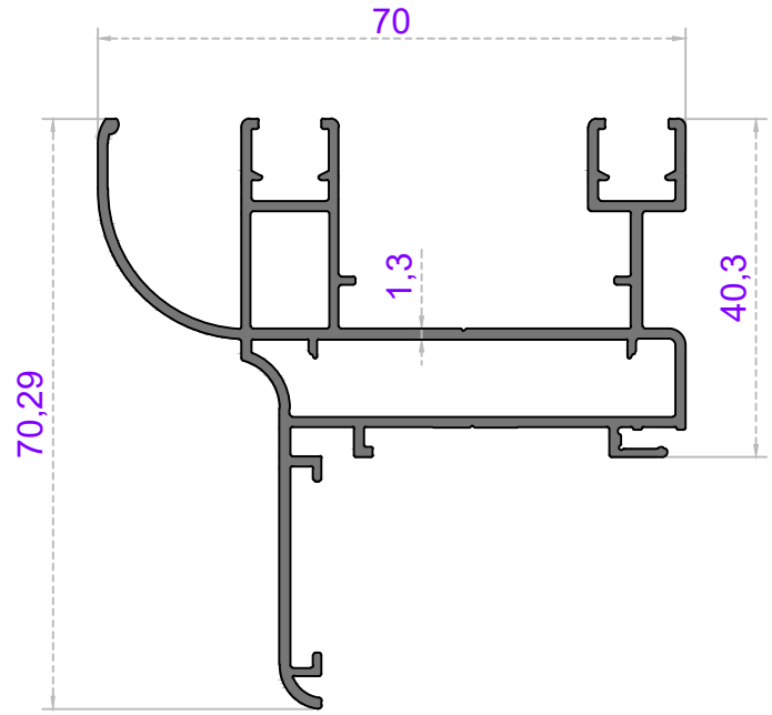
Sistem Kodu 49-4782 Ağırlık (kg/mt) 1,115
