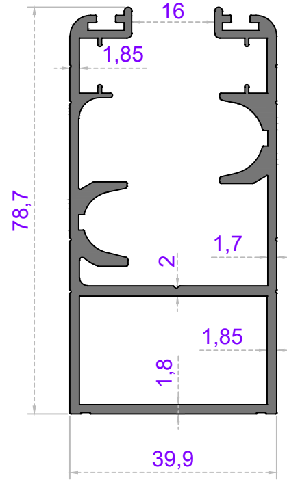
Sistem Kodu 41-2765 Ağırlık (kg/mt) 1,615
