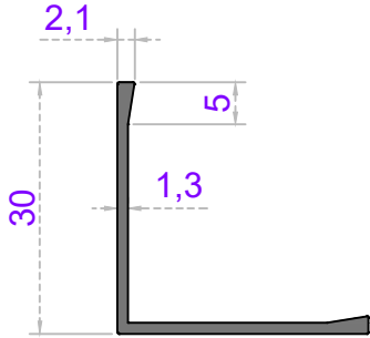
Sistem Kodu 39-1286 Ağırlık (kg/mt) 0,220
