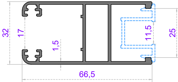
Sistem Kodu 47-4033 Ağırlık (kg/mt) 0,930
