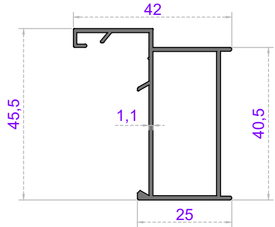
KASA
