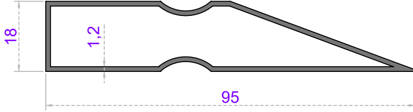
Sistem Kodu 80-5064 Ağırlık (kg/mt) 0,672
