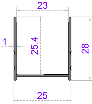
GENİŞ DUVAR DİKMESİ
