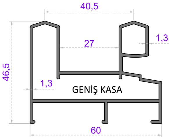
Sistem Kodu 47-4034 Ağırlık (kg/mt) 0,990
