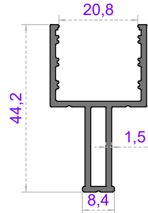
Sistem Kodu 59-7011 Ağırlık (kg/mt) 0,515
