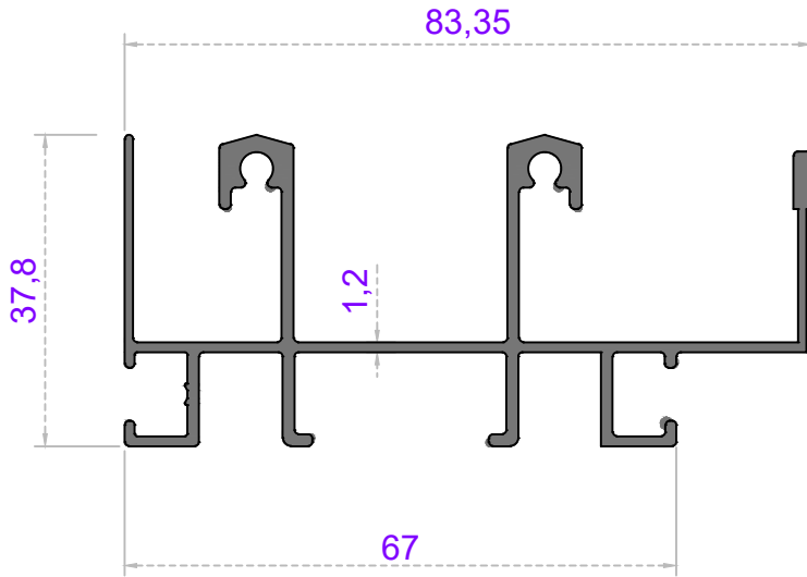
Sistem Kodu 54-4730 Ağırlık (kg/mt) 1,063
