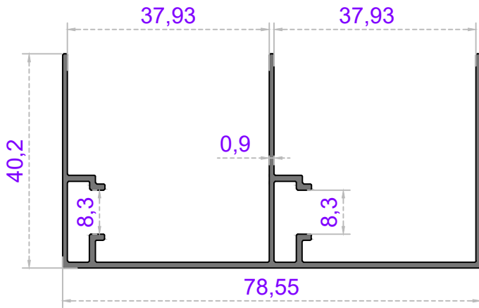
Sistem Kodu 48-4260 Ağırlık (kg/mt) 0,615
