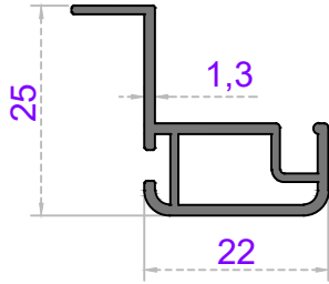
Sistem Kodu 40-1318 Ağırlık (kg/mt) 0,302
