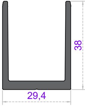
Sistem Kodu 36-1107 Ağırlık (kg/mt) 0,745
