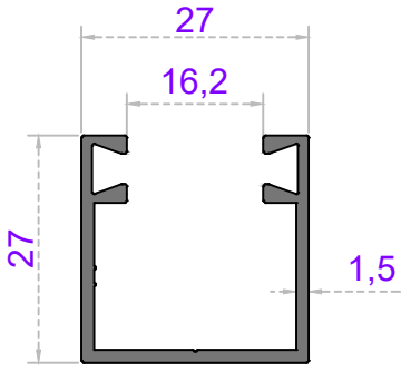
Sistem Kodu 54-4709 Ağırlık (kg/mt) 0,395
