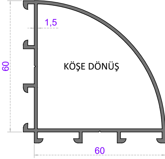
Sistem Kodu 62-1702 Ağırlık (kg/mt) 1,100
