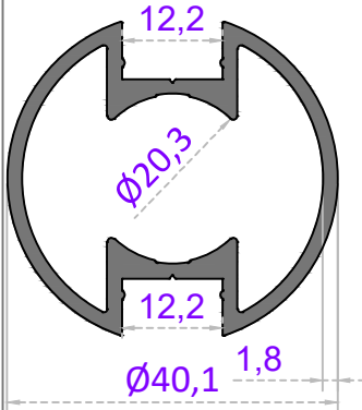
Ø 40'LIK DİKME
