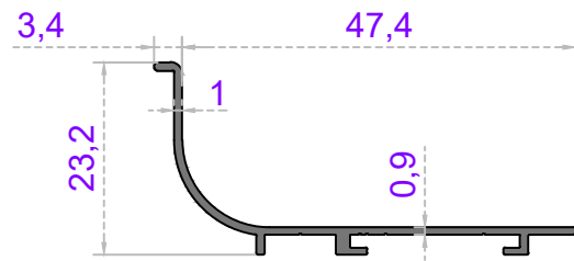
Sistem Kodu 48-4261 Ağırlık (kg/mt) 0,199
