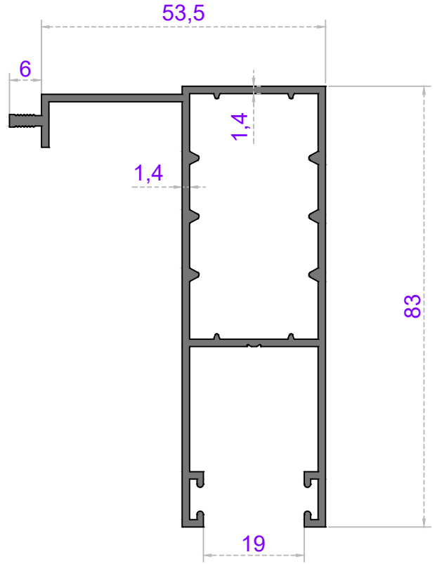
Sistem Kodu 54-4818 Ağırlık (kg/mt) 1,100
