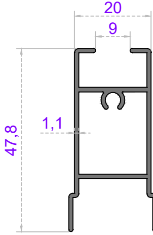
KANAT ÜST
