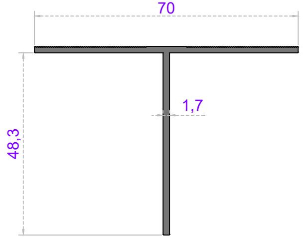
Sistem Kodu 26-407 Ağırlık (kg/mt) 0,525
