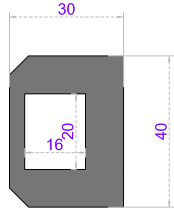
Sistem Kodu 58-2412 Ağırlık (kg/mt) 2,337
