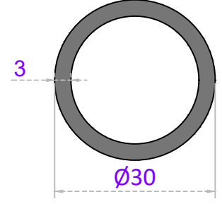
Sistem Kodu 22-209 Ağırlık (kg/mt) 0,690
