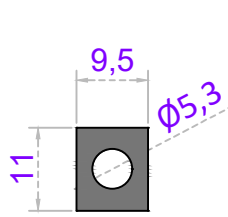
Sistem Kodu 58-2219 Ağırlık (kg/mt) 0,225
