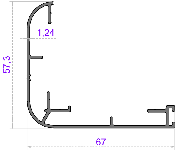
Sistem Kodu 54-4745 Ağırlık (kg/mt) 0,650
