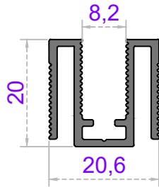
Sistem Kodu 59-7015 Ağırlık (kg/mt) 0,365
