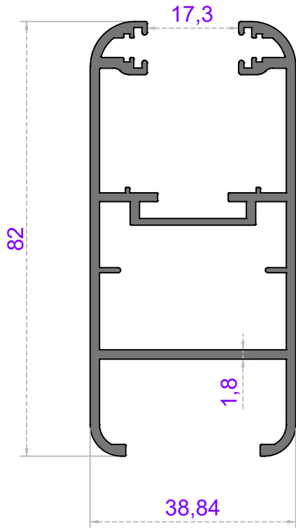
Sistem Kodu 49-4377 Ağırlık (kg/mt) 1,400
