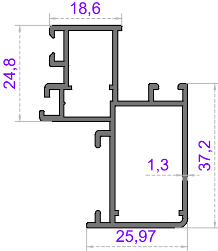
Sistem Kodu 50-1488 Ağırlık (kg/mt) 0,776
