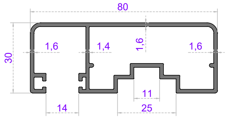
Sistem Kodu 58-2298 Ağırlık (kg/mt) 1,125
