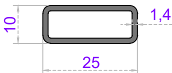
Sistem Kodu 58-2259 Ağırlık (kg/mt) 0,240
