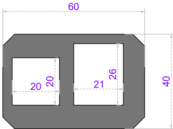
Sistem Kodu 58-2413 Ağırlık (kg/mt) 3,825
