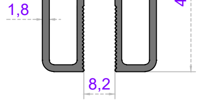
Sistem Kodu 41-2813 Ağırlık (kg/mt) 1,585
