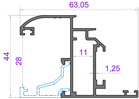
Sistem Kodu 49-4304 Ağırlık (kg/mt) 0,740
