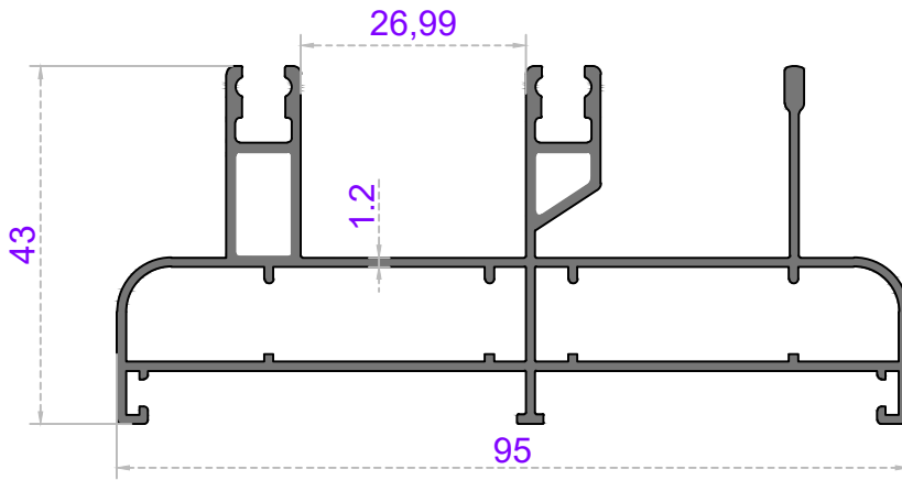
Sistem Kodu 49-4779 Ağırlık (kg/mt) 1.220
