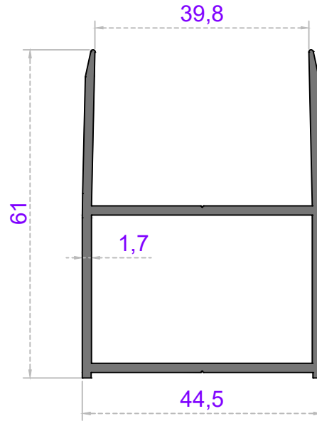
Sistem Kodu 41-2306 Ağırlık (kg/mt) 0,935
