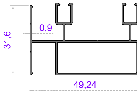
Sistem Kodu 49-4422 Ağırlık (kg/mt) 0,480
