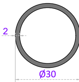
Sistem Kodu 22-200 Ağırlık (kg/mt) 0,480
