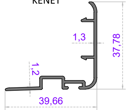
Sistem Kodu 47-4035 Ağırlık (kg/mt) 0,340
