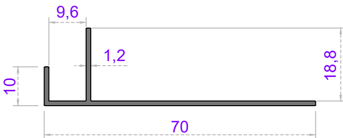
Sistem Kodu 26-415 Ağırlık (kg/mt) 0,290
