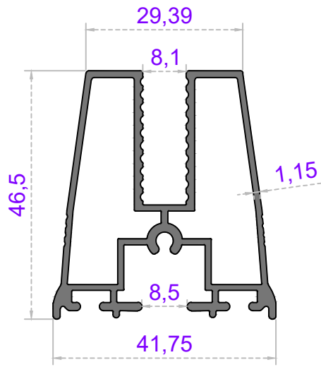
Sistem Kodu 41-2906 Ağırlık (kg/mt) 0,918
