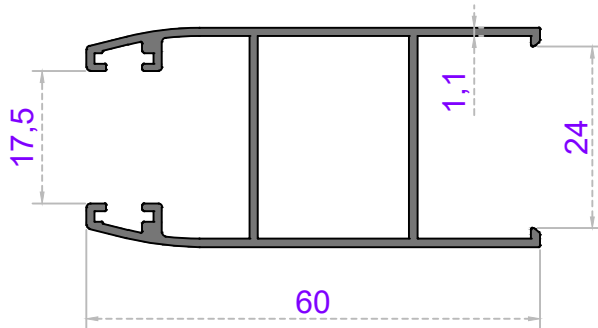
Sistem Kodu 49-4387 Ağırlık (kg/mt) 0,595
