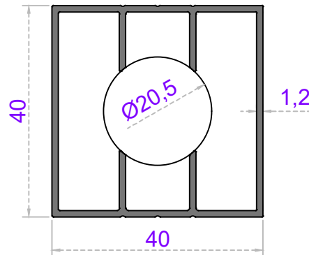
Sistem Kodu 58-2370 Ağırlık (kg/mt) 0,649
