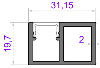
Sistem Kodu 58-2267 Ağırlık (kg/mt) 0,515
