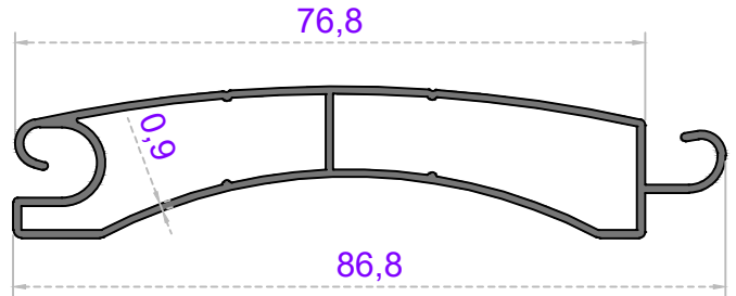
Sistem Kodu 38-1217 Ağırlık (kg/mt) 0,580
