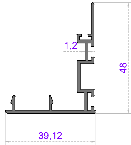
Sistem Kodu 49-4378 Ağırlık (kg/mt) 0,455
