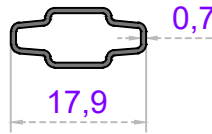
Sistem Kodu 47-4031 Ağırlık (kg/mt) 0,095
