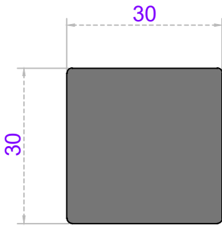
Sistem Kodu 80-5030 Ağırlık (kg/mt) 2,440
