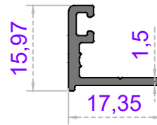
Sistem Kodu 54-4777 Ağırlık (kg/mt) 0,166
