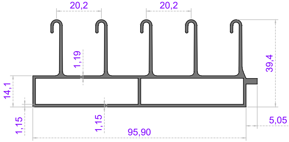
Sistem Kodu 41-2373 Ağırlık (kg/mt) 1,350
