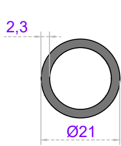
Sistem Kodu 22-245 Ağırlık (kg/mt) 0,370
