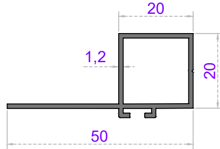
Sistem Kodu 39-1346 Ağırlık (kg/mt) 0,385
