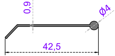
MENFEZ KANAT
