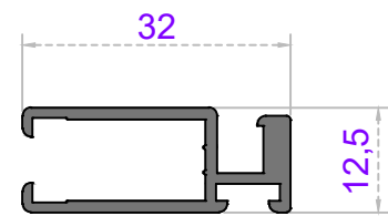
Sistem Kodu 49-4306 Ağırlık (kg/mt) 0,335
