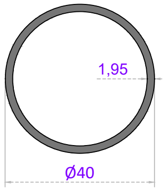
Ø 40'LUK BORU
