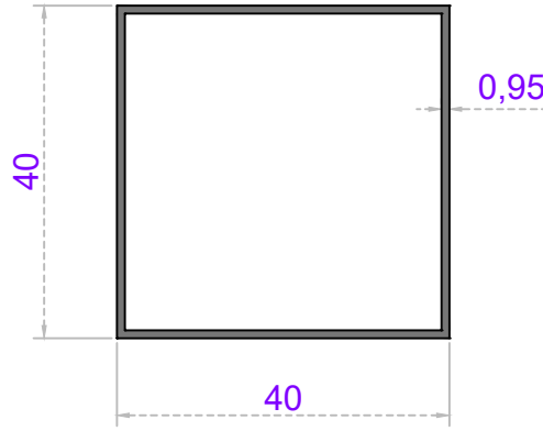
Sistem Kodu 20-103 Ağırlık (kg/mt) 0,410
