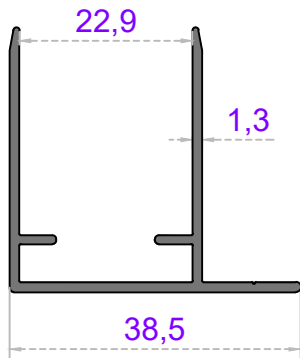
Sistem Kodu 66-1310 Ağırlık (kg/mt) 0,405
