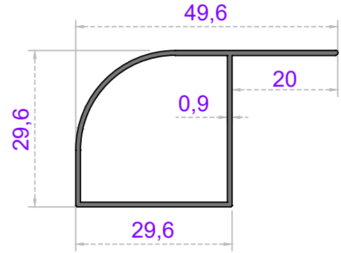
KULAKLI KÖŞE DÖNÜŞ
