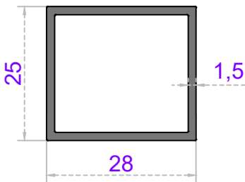
Sistem Kodu 20-200 Ağırlık (kg/mt) 0,410
