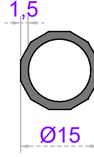
Sistem Kodu 22-233 Ağırlık (kg/mt) 0,185
