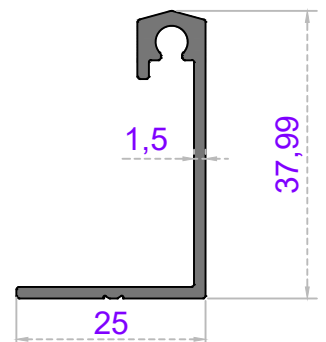
Sistem Kodu 54-4834 Ağırlık (kg/mt) 0,350
