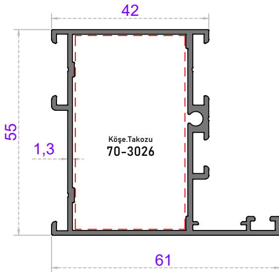
Sistem Kodu 55-2107 Ağırlık (kg/mt) 0,925
