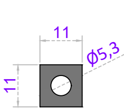
Sistem Kodu 58-2217 Ağırlık (kg/mt) 0,270
