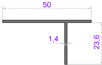
Sistem Kodu 26-402 Ağırlık (kg/mt) 0,280
