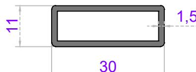
Sistem Kodu 20-117 Ağırlık (kg/mt) 0,315
