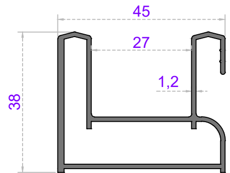
Sistem Kodu 49-4353 Ağırlık (kg/mt) 0,700
