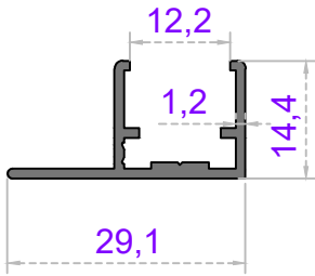
Sistem Kodu 54-4815 Ağırlık (kg/mt) 0,210
