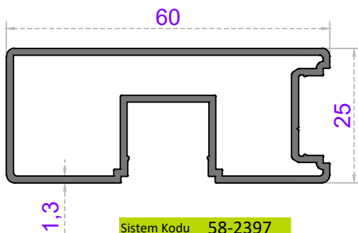
Sistem Kodu 58-2397 Ağırlık (kg/mt) 0,730
