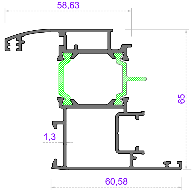
Sistem Kodu 70-3092 Ağırlık (kg/mt) 1,525
