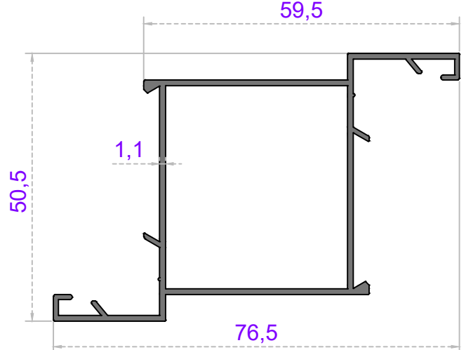
KANAT
