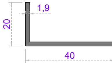
Sistem Kodu 24-306 Ağırlık (kg/mt) 0,300
