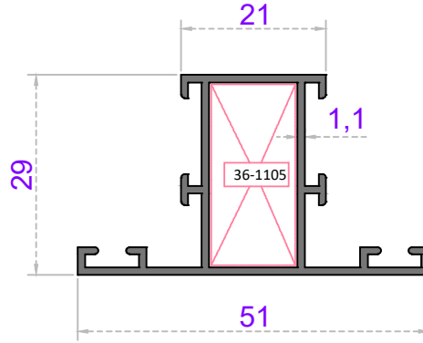
ORTA KAYIT
