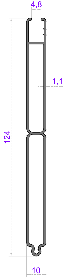
Sistem Kodu 49-4356 Ağırlık (kg/mt) 0,800
