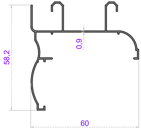
Sistem Kodu 49-4380 Ağırlık (kg/mt) 0,480
