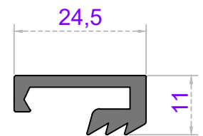
Sistem Kodu 56-1508 Ağırlık (kg/mt) 0,315
