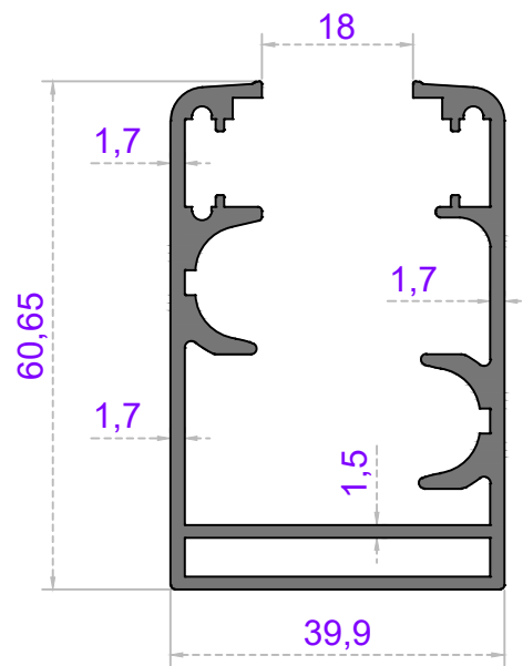
Sistem Kodu 41-2384 Ağırlık (kg/mt) 1,300
