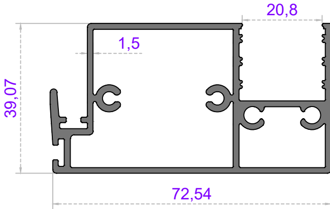
Sistem Kodu 59-7008 Ağırlık (kg/mt) 1,410
