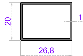
Sistem Kodu 20-184 Ağırlık (kg/mt) 0,245
