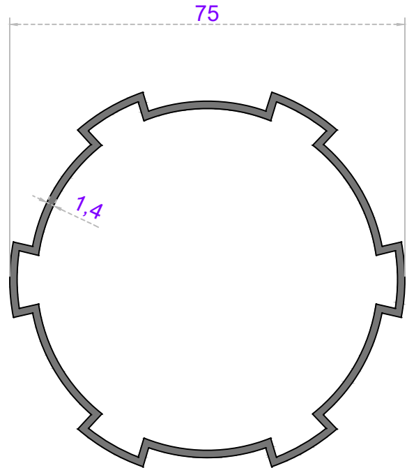
Sistem Kodu 59-7014 Ağırlık (kg/mt) 0,180
