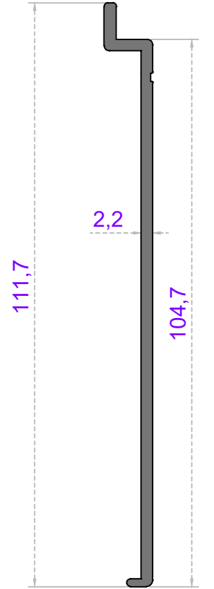
Sistem Kodu 56-1506 Ağırlık (kg/mt) 0,720
