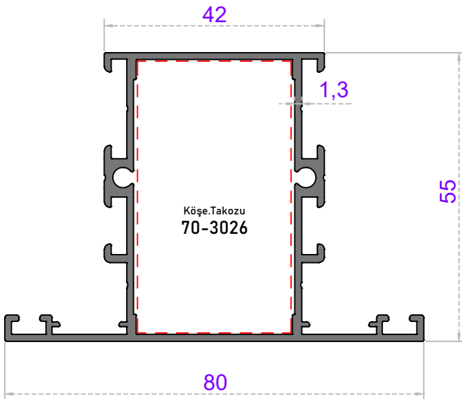
Sistem Kodu 55-2105 Ağırlık (kg/mt) 1,100
