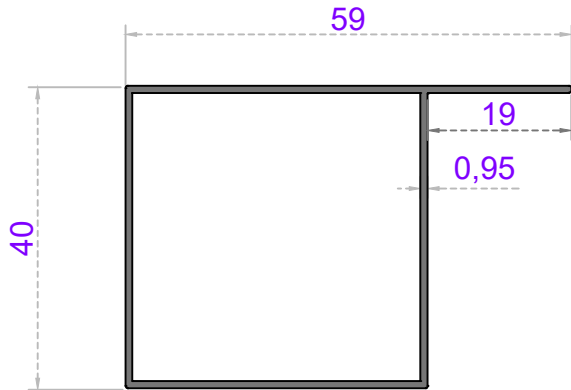
Sistem Kodu 33-1047 Ağırlık (kg/mt) 0,455
