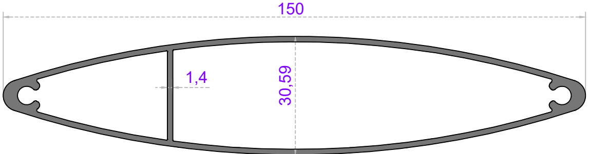
GÜNEŞ KIRICI
