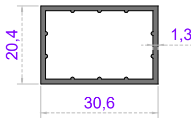
Sistem Kodu 20-120 Ağırlık (kg/mt) 0,355
