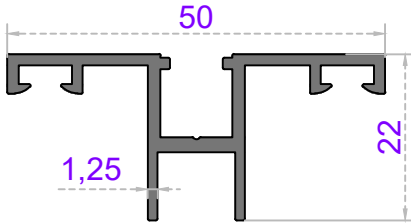
Sistem Kodu 50-1605 Ağırlık (kg/mt) 0,465
