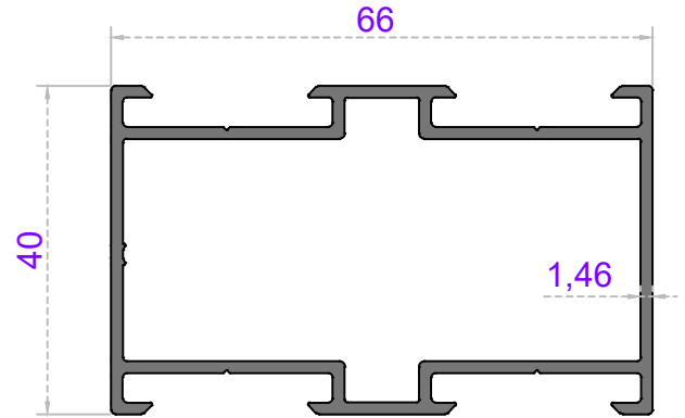
Sistem Kodu 54-4743 Ağırlık (kg/mt) 0,985
