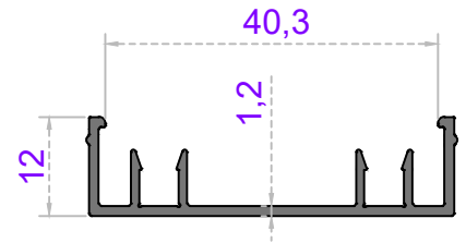
Sistem Kodu 50-1625 Ağırlık (kg/mt) 0,292
