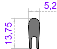
SÜRME RAY
