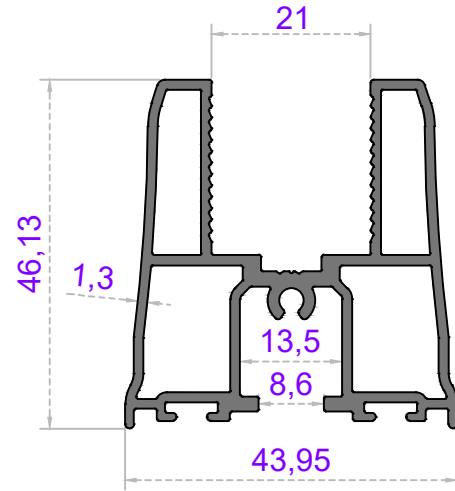
Sistem Kodu 41-2703 Ağırlık (kg/mt) 1,026
