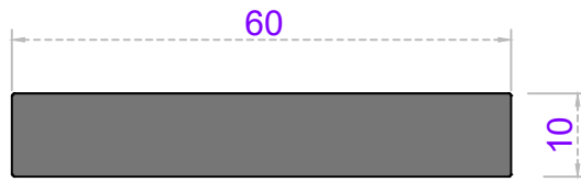
Sistem Kodu 80-5121 Ağırlık (kg/mt) 1,630
