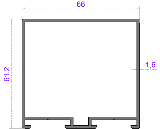
Sistem Kodu 54-4743 Ağırlık (kg/mt) 0,985
