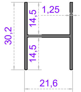
Sistem Kodu 62-1719 Ağırlık (kg/mt) 0,270
