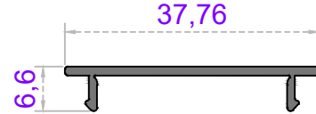
Sistem Kodu 59-7014 Ağırlık (kg/mt) 0,180
