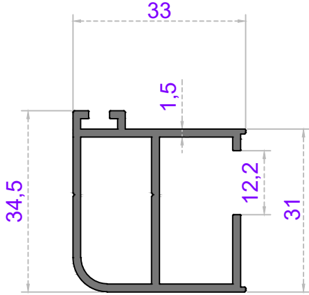
Sistem Kodu 39-1329 Ağırlık (kg/mt) 0,590
