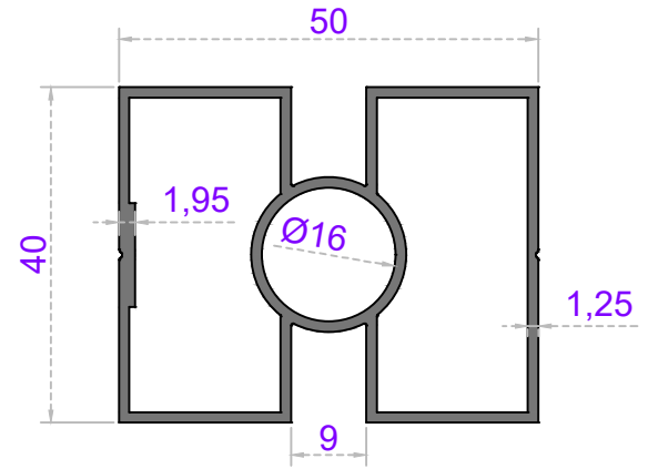
Sistem Kodu 58-2315 Ağırlık (kg/mt) 0,890
