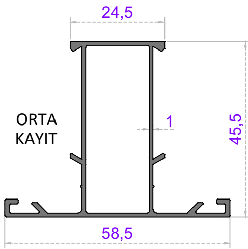
ORTA KAYIT
