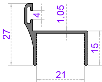
Sistem Kodu 41-2706 Ağırlık (kg/mt) 0,241
