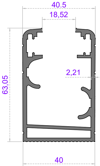
Sistem Kodu 41-2462 Ağırlık (kg/mt) 1,471
