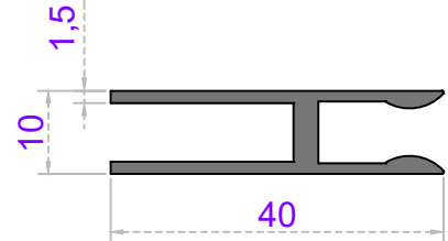
Sistem Kodu 34-1066 Ağırlık (kg/mt) 0,380
