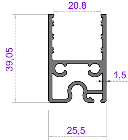
Sistem Kodu 59-7009 Ağırlık (kg/mt) 0,700
