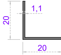
Sistem Kodu 24-301 Ağırlık (kg/mt) 0,116
