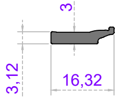
Sistem Kodu 57-2523 Ağırlık (kg/mt) 0,125
