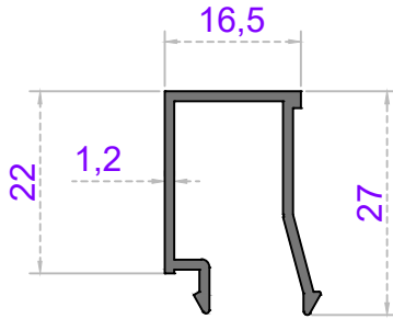
KASA ISICAM ÇITA
