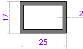
Sistem Kodu 20-151 Ağırlık (kg/mt) 0,415
