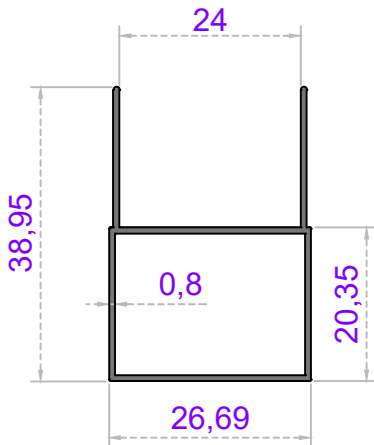
Sistem Kodu 40-1321 Ağırlık (kg/mt) 0,280
