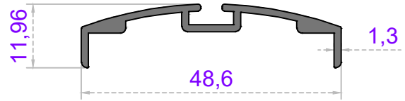
ÇARPMA KAPI DIŞ
