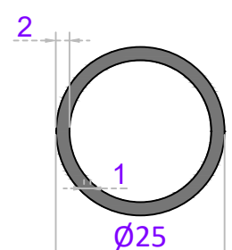
Sistem Kodu 22-263 Ağırlık (kg/mt) 0,392
