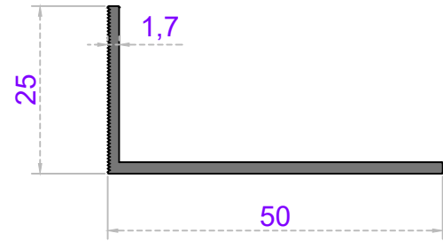
Sistem Kodu 24-316 Ağırlık (kg/mt) 0,330
