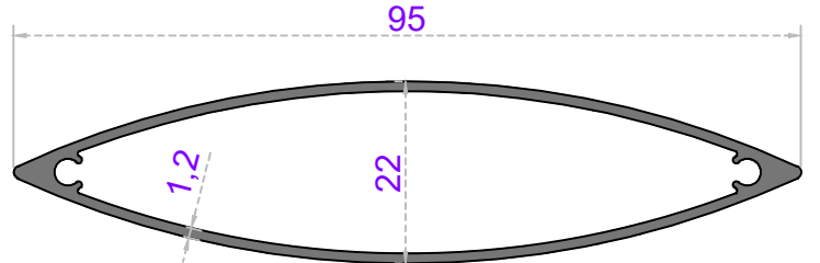
GÜNEŞ KIRICI
