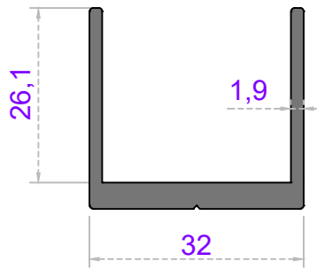
GENİŞ - U -
