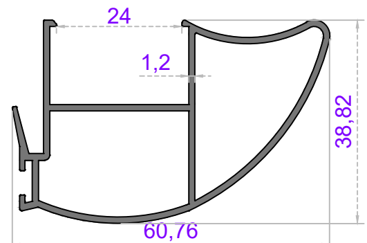
Sistem Kodu 49-4780 Ağırlık (kg/mt) 0,720
