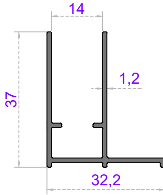
DUVAR DİKMESİ
