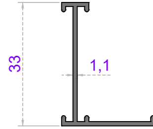
TAŞIYICI -L-
