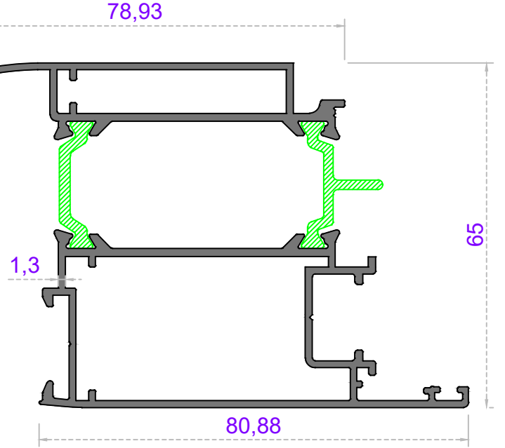
Sistem Kodu 70-3091 Ağırlık (kg/mt) 1,850
