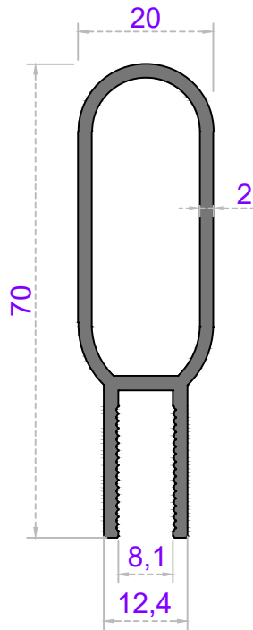
Sistem Kodu 80-5109 Ağırlık (kg/mt) 0,870
