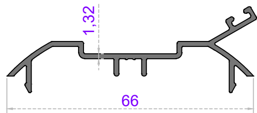
Sistem Kodu 54-4744 Ağırlık (kg/mt) 0,433
