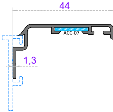
PERVAZ
