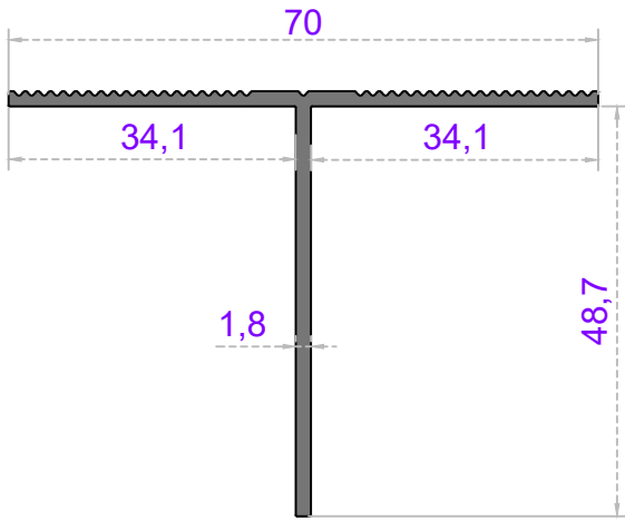
Sistem Kodu 50-1640 Ağırlık (kg/mt) 0,540
