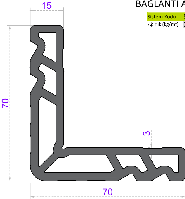
Sistem Kodu 50-1615 Ağırlık (kg/mt) 2,400
