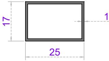
Sistem Kodu 20-100 Ağırlık (kg/mt) 0,220
