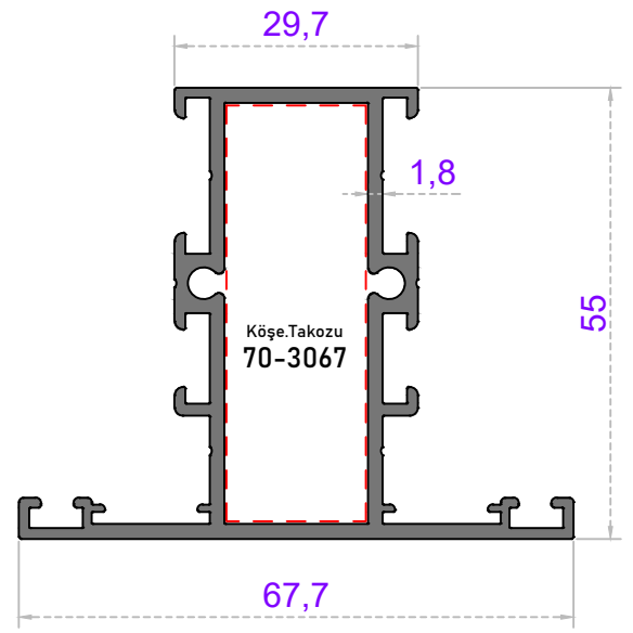
Sistem Kodu 55-2126 Ağırlık (kg/mt) 1,215
