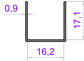
ASMA TAVAN -U-
