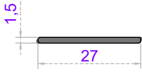
Sistem Kodu 41-2831 Ağırlık (kg/mt) 0,110
