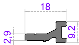
Sistem Kodu 50-1620 Ağırlık (kg/mt) 0,195
