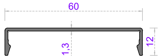
Sistem Kodu 50-11005 Ağırlık (kg/mt) 0,305
