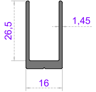
DAR - U - (IRAK İÇİN)
