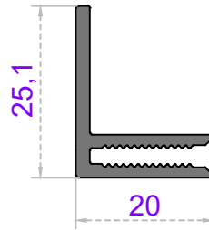
Sistem Kodu 50-1667 Ağırlık (kg/mt) 0,315
