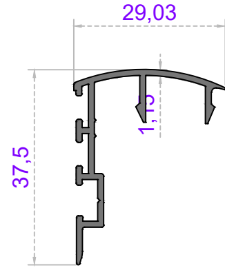
Sistem Kodu 49-4354 Ağırlık (kg/mt) 0,305
