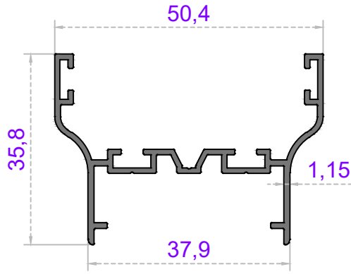
Sistem Kodu 41-2959 Ağırlık (kg/mt) 0,458
