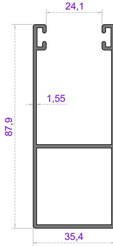
Sistem Kodu 38-1210 Ağırlık (kg/mt) 1,095
