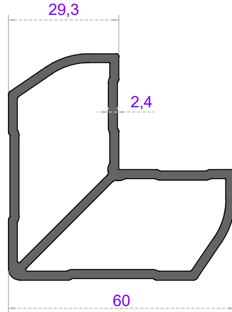
Sistem Kodu 36-1117 Ağırlık (kg/mt) 1,645
