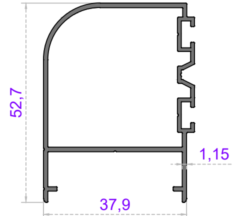
Sistem Kodu 41-2964 Ağırlık (kg/mt) 0,617
