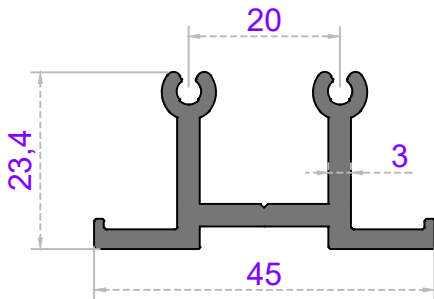
Sistem Kodu 50-1621 Ağırlık (kg/mt) 0,730
