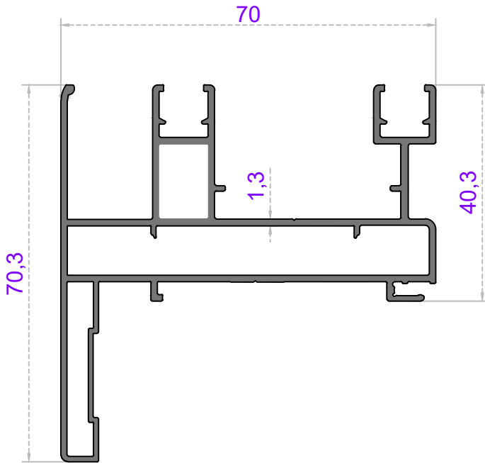
Sistem Kodu 49-4783 Ağırlık (kg/mt) 1,248
