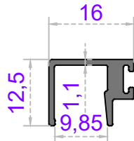
Sistem Kodu 66-1402 Ağırlık (kg/mt) 0,165
