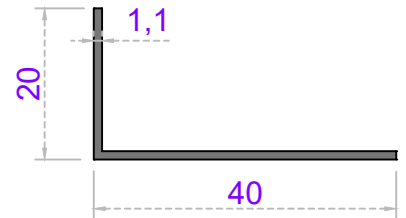
Sistem Kodu 24-304 Ağırlık (kg/mt) 0,175
