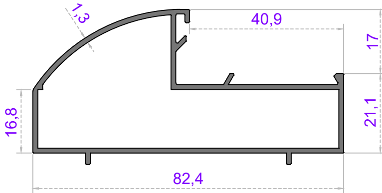
Sistem Kodu 38-1236 Ağırlık (kg/mt) 0,865
