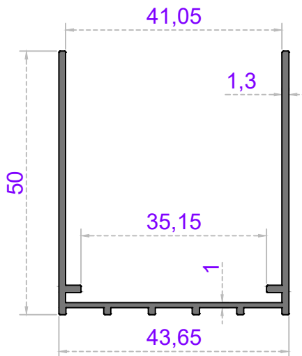
Sistem Kodu 41-2717 Ağırlık (kg/mt) 0,510
