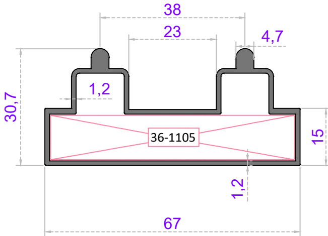
RAYLI KASA
