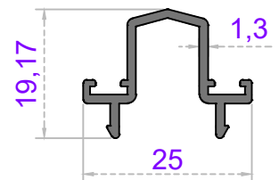
Sistem Kodu 47-4037 Ağırlık (kg/mt) 0,225
