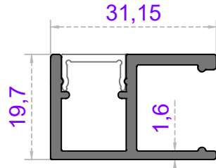
Sistem Kodu 58-2252 Ağırlık (kg/mt) 0,445
