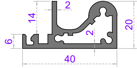
Sistem Kodu 57-2522 Ağırlık (kg/mt) 0,715
