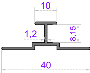
Sistem Kodu 26-418 Ağırlık (kg/mt) 0,207
