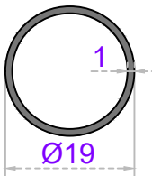
Sistem Kodu 22-257 Ağırlık (kg/mt) 0,155
