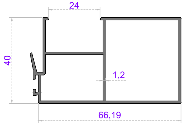
Sistem Kodu 49-4393 Ağırlık (kg/mt) 0,872
