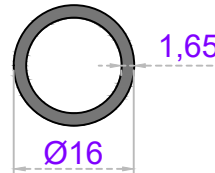
Sistem Kodu 22-208 Ağırlık (kg/mt) 0,210
