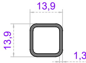
Sistem Kodu 58-2235 Ağırlık (kg/mt) 0,160
