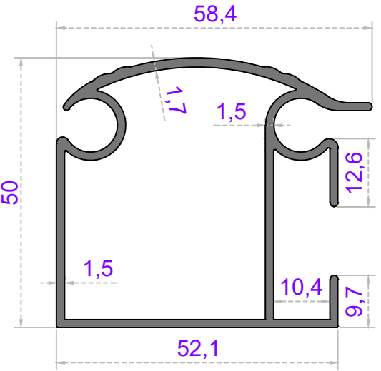
Sistem Kodu 57-2530 Ağırlık (kg/mt) 1,055
