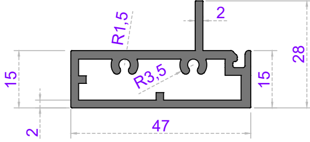
Sistem Kodu 57-2521 Ağırlık (kg/mt) 0,870
