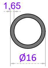
Sistem Kodu 22-208 Ağırlık (kg/mt) 0,205
