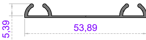
Sistem Kodu 48-4237 Ağırlık (kg/mt) 0,215
