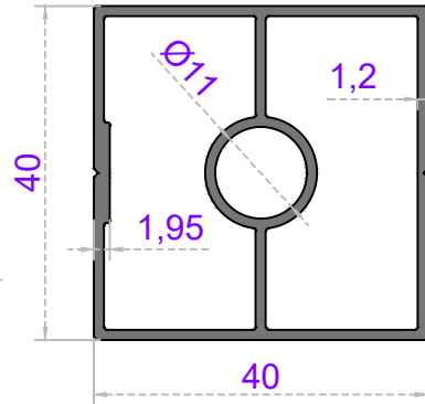
Sistem Kodu 58-2317 Ağırlık (kg/mt) 0,735
