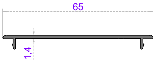
Sistem Kodu 54-4708 Ağırlık (kg/mt) 0,285
