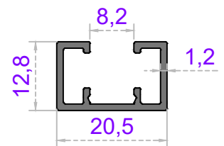
Sistem Kodu 41-2875 Ağırlık (kg/mt) 0,200
