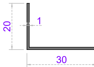
Sistem Kodu 24-317 Ağırlık (kg/mt) 0,135
