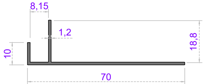
Sistem Kodu 39-416 Ağırlık (kg/mt) 0,322
