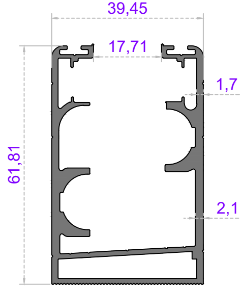
Sistem Kodu 41-2937 Ağırlık (kg/mt) 1.295
