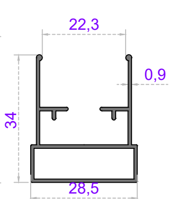
Sistem Kodu 40-1315 Ağırlık (kg/mt) 0,355
