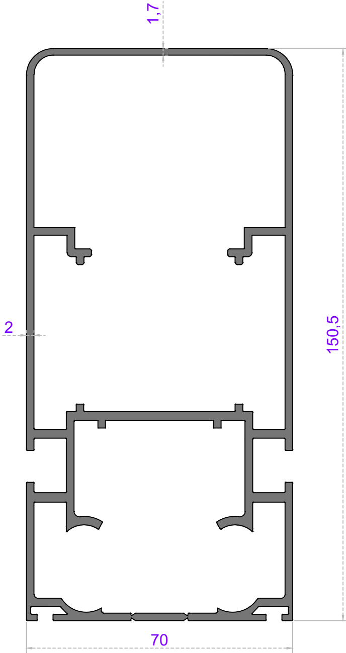
Sistem Kodu 57-2554 Ağırlık (kg/mt) 3,475
