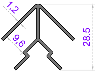
Sistem Kodu 26-420 Ağırlık (kg/mt) 0,315
