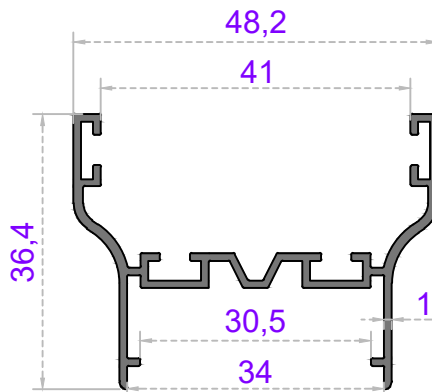
Sistem Kodu 41-2942 Ağırlık (kg/mt) 0,450
