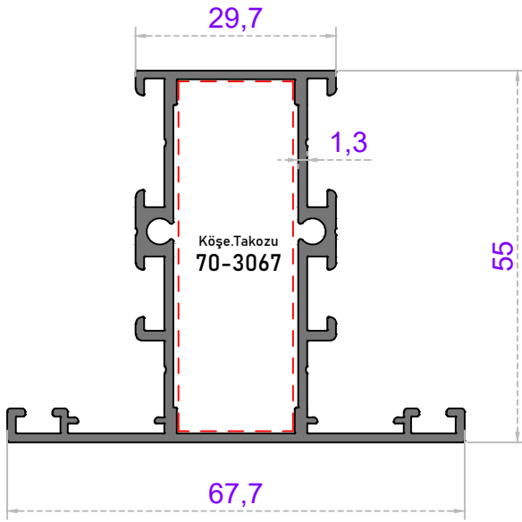
Sistem Kodu 55-2101 Ağırlık (kg/mt) 1,000
