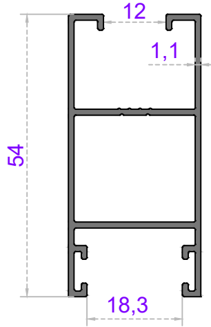
Sistem Kodu 54-4772 Ağırlık (kg/mt) 0,554
