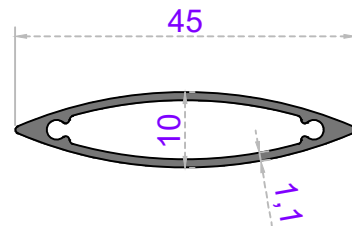
GÜNEŞ KIRICI
