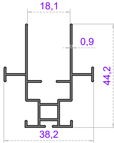
Sistem Kodu 40-1314-Ö Ağırlık (kg/mt) 0,425
