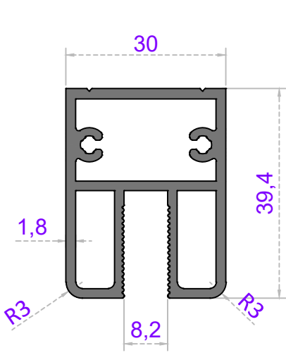
Sistem Kodu 41-2810 Ağırlık (kg/mt) 1,003
