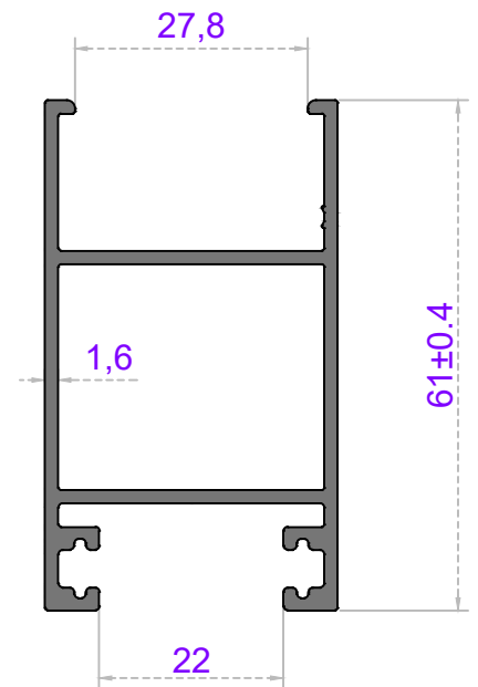
Sistem Kodu 54-4835 Ağırlık (kg/mt) 0,960
