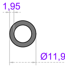
Sistem Kodu 22-239 Ağırlık (kg/mt) 0,166
