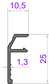
ÖZEL KASA ÇİTASI
