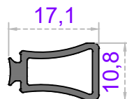
Sistem Kodu 41-2877 Ağırlık (kg/mt) 0,165
