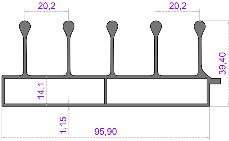
Sistem Kodu 41-2911 Ağırlık (kg/mt) 1,490
