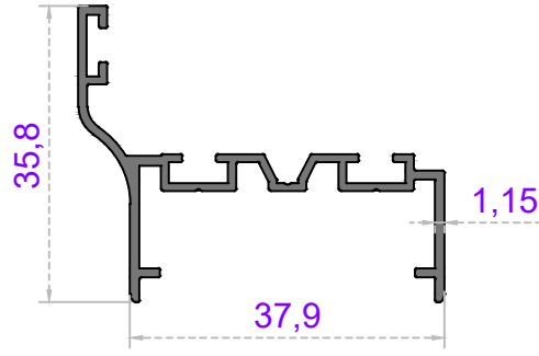
Sistem Kodu 41-2960 Ağırlık (kg/mt) 0,380
