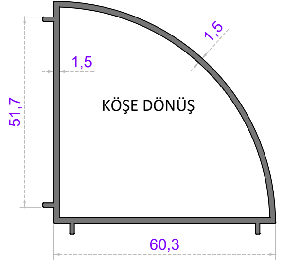
Sistem Kodu 62-1717 Ağırlık (kg/mt) 0,895
