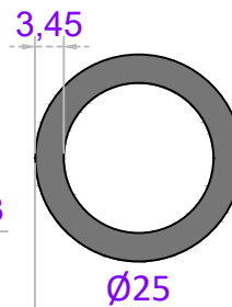
Sistem Kodu 22-240 Ağırlık (kg/mt) 0,635
