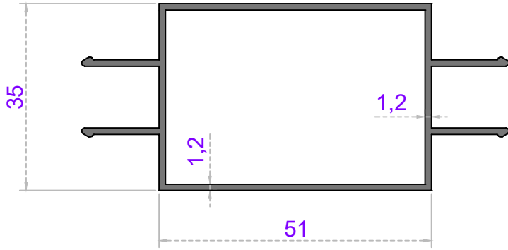
Sistem Kodu 38-1203 Ağırlık (kg/mt) 0,740
