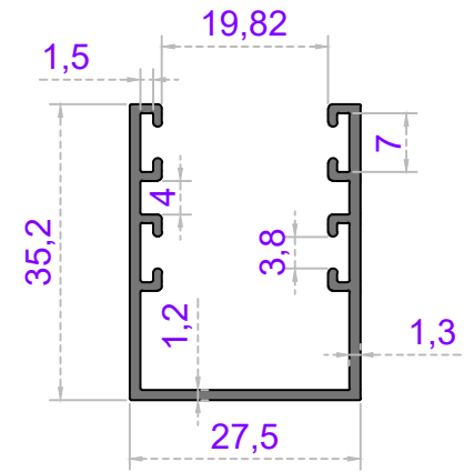
Sistem Kodu 41-2760 Ağırlık (kg/mt) 0,421
