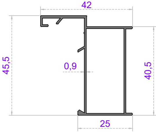
KASA
