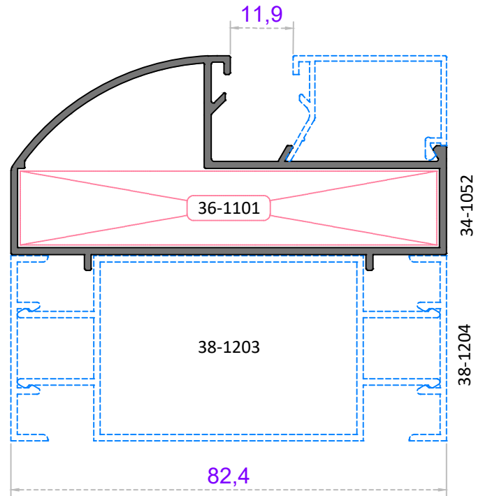
MONTAJ DETAYI
