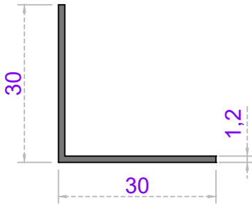
Sistem Kodu 24-303 Ağırlık (kg/mt) 0,191
