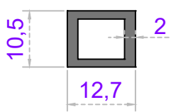
Sistem Kodu 41-2381 Ağırlık (kg/mt) 0,190
