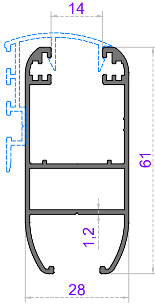
Sistem Kodu 49-4352 Ağırlık (kg/mt) 0,710
