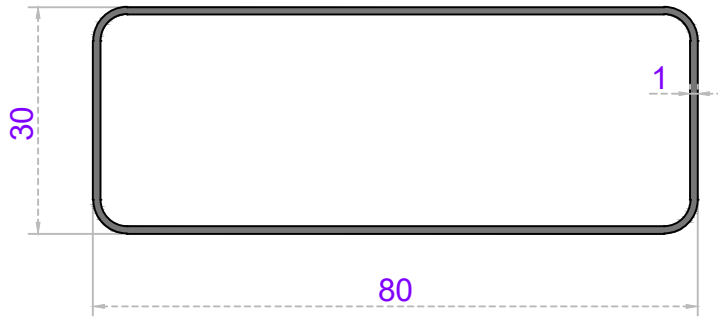
Sistem Kodu 20-119 Ağırlık (kg/mt) 0,570
