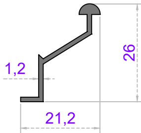
SİNEKLİK RAY
