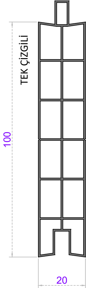
TEK ÇİZGİLİ ÇİFT ODACIKLI 10'LUK KAPI LAMBRI
