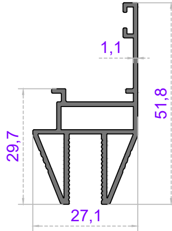
Sistem Kodu 41-2904 Ağırlık (kg/mt) 0,558
