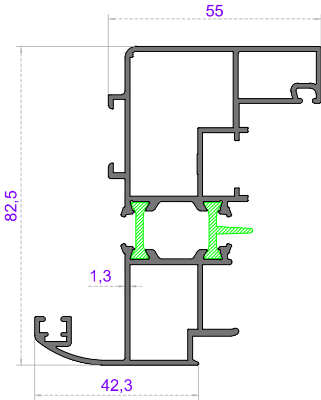
Sistem Kodu 70-3072 Ağırlık (kg/mt) 1,660
