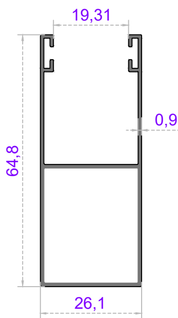
Sistem Kodu 38-1243 Ağırlık (kg/mt) 0,480
