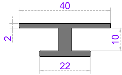
Sistem Kodu 26-409 Ağırlık (kg/mt) 0,530
