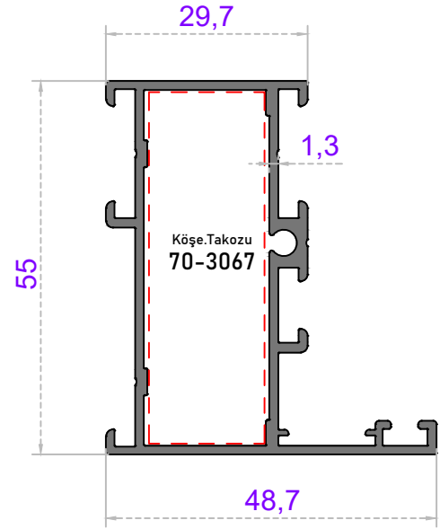
Sistem Kodu 55-2103 Ağırlık (kg/mt) 0,960
