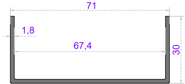
Sistem Kodu 66-1433 Ağırlık (kg/mt) 0,625
