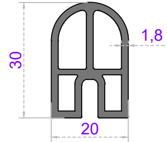
Sistem Kodu 20-170 Ağırlık (kg/mt) 0,645
