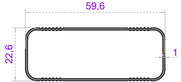
Sistem Kodu 20-187 Ağırlık (kg/mt) 0,410
