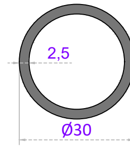
Sistem Kodu 22-201 Ağırlık (kg/mt) 0,586
