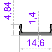
Sistem Kodu 58-2322 Ağırlık (kg/mt) 0,072
