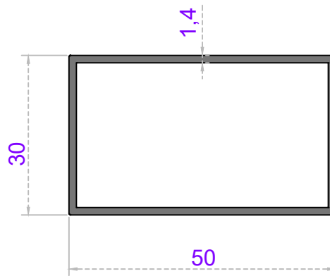
Sistem Kodu 20-150 Ağırlık (kg/mt) 0,590
