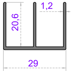
Sistem Kodu 62-1716 Ağırlık (kg/mt) 0,310
