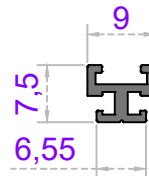
Sistem Kodu 48-4241 Ağırlık (kg/mt) 0,085
