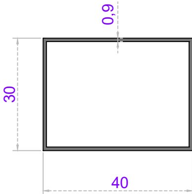
Sistem Kodu 20-102 Ağırlık (kg/mt) 0,335
