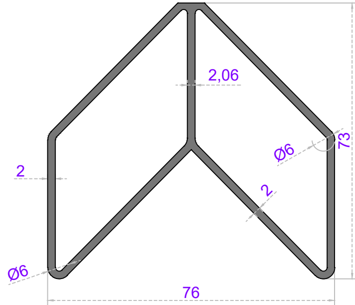
Sistem Kodu 62-1734 Ağırlık (kg/mt) 1,700
