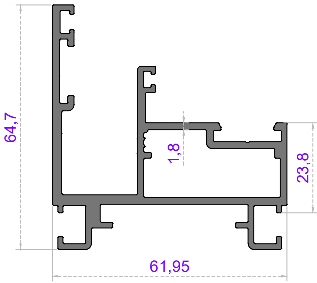
Sistem Kodu 54-4796 Ağırlık (kg/mt) 1,505
