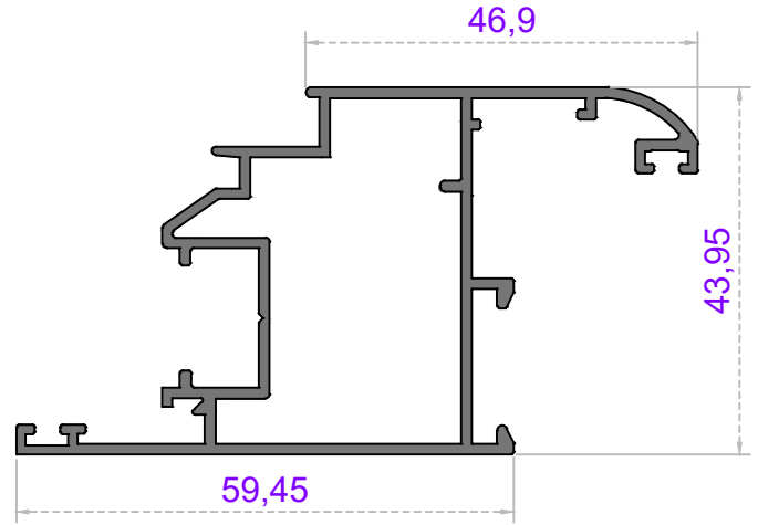
Sistem Kodu 49-4413 Ağırlık (kg/mt) 0,960
