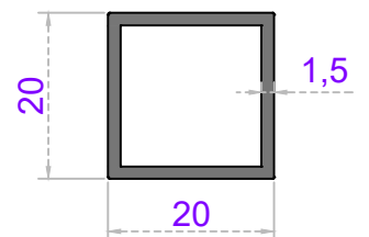
Sistem Kodu 20-167 Ağırlık (kg/mt) 0,310
