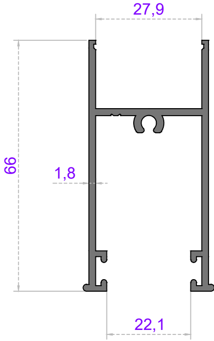
Sistem Kodu 54-4817 Ağırlık (kg/mt) 0,920
