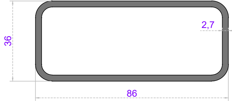
Sistem Kodu 58-2245 Ağırlık (kg/mt) 1,630
