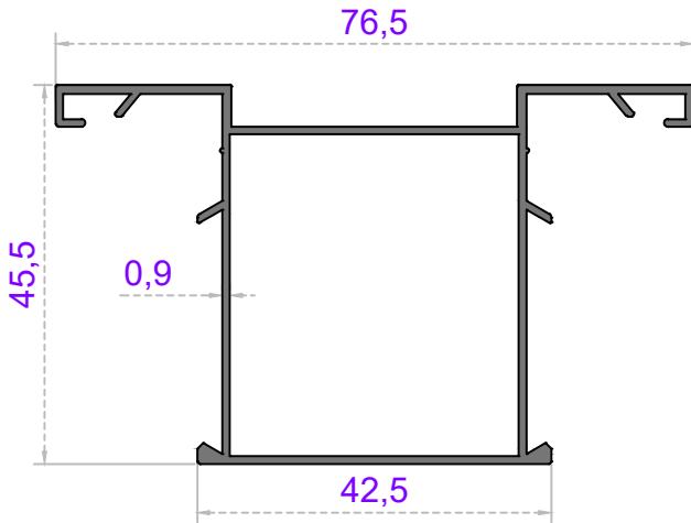
ORTA KAYIT
