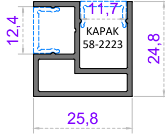
Sistem Kodu 41-2856 Ağırlık (kg/mt) 0,395
