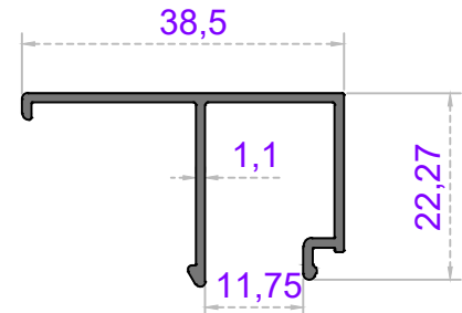
TEK CAM ÇITA
