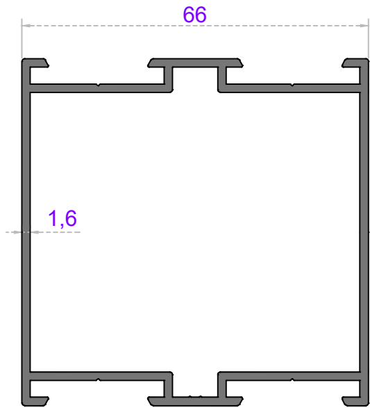
Sistem Kodu 54-4704 Ağırlık (kg/mt) 1,335
