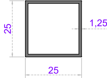
Sistem Kodu 20-126 Ağırlık (kg/mt) 0,325
