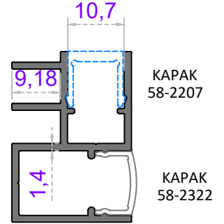
Sistem Kodu 58-2367 Ağırlık (kg/mt) 0,420
