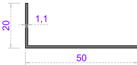
Sistem Kodu 24-305 Ağırlık (kg/mt) 0,205
