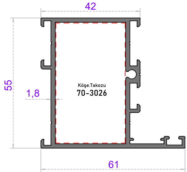
Sistem Kodu 55-2132 Ağırlık (kg/mt) 1,150
