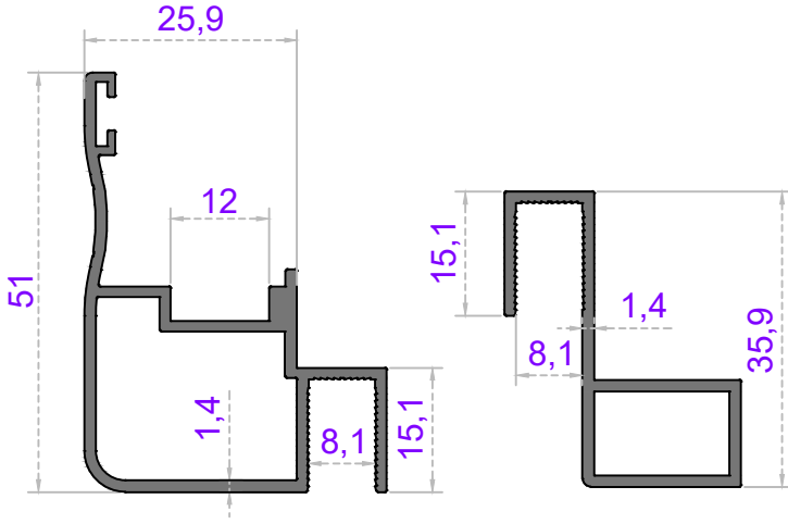
Sistem Kodu 41-2798 Ağırlık (kg/mt) 0,615
