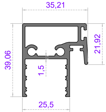
Sistem Kodu 59-7010 Ağırlık (kg/mt) 0,820
