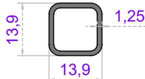
Sistem Kodu 58-2235 Ağırlık (kg/mt) 0,160
