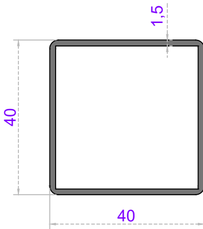
Sistem Kodu 20-132 Ağırlık (kg/mt) 0,625
