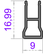
Sistem Kodu 50-1668 Ağırlık (kg/mt) 0,120
