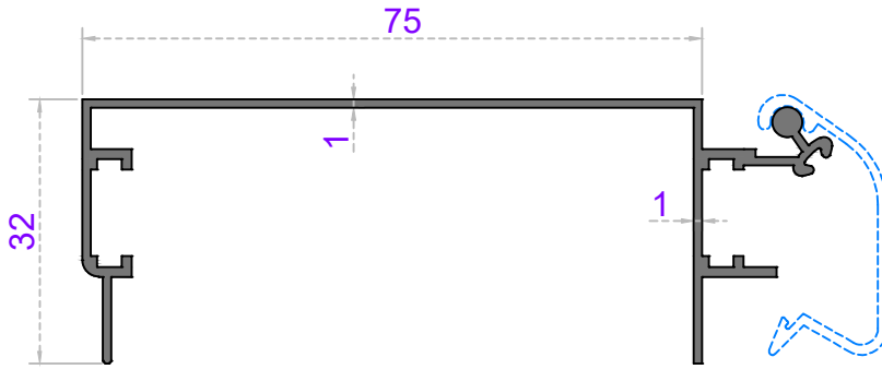
ÖZEL KASA
