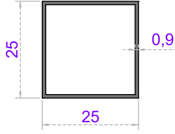
Sistem Kodu 20-143 Ağırlık (kg/mt) 0,236
