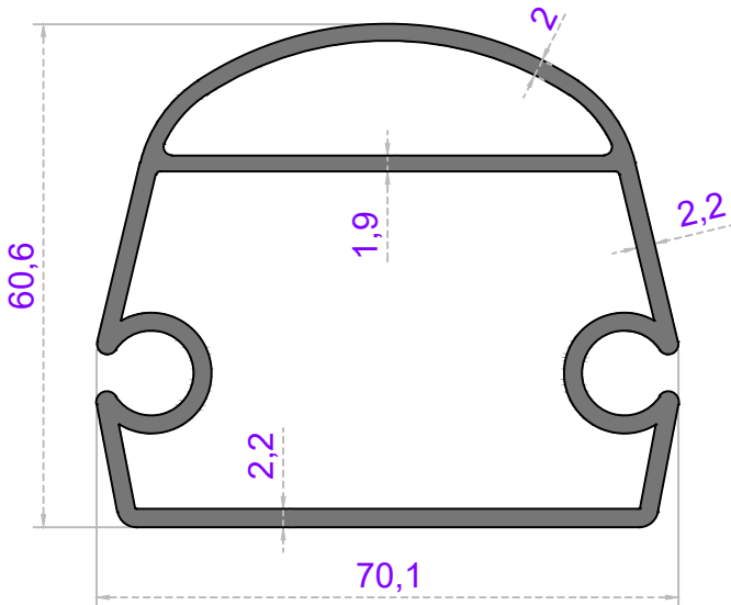
Sistem Kodu 57-2513 Ağırlık (kg/mt) 1,840
