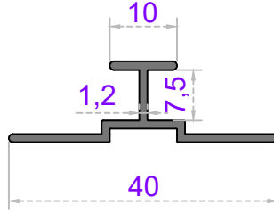
Sistem Kodu 26-413 Ağırlık (kg/mt) 0,205
