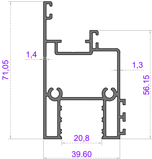
Sistem Kodu 59-7012 Ağırlık (kg/mt) 1,183
