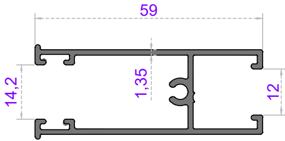
Sistem Kodu 54-4735 Ağırlık (kg/mt) 0,642
