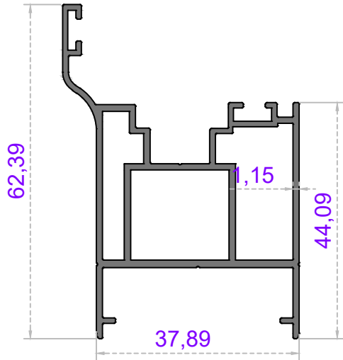
Sistem Kodu 41-2963 Ağırlık (kg/mt) 0,842
