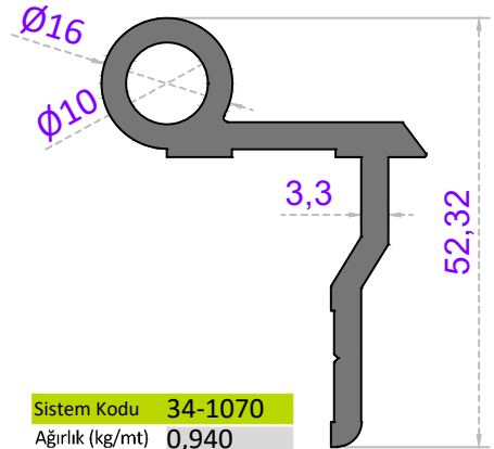
ALDOKS DÜZ KANAT MENTEŞE
