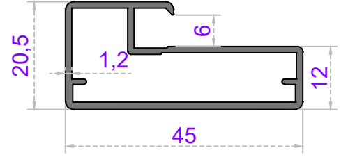
Sistem Kodu 48-4227 Ağırlık (kg/mt) 0,475
