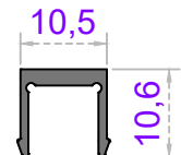
Sistem Kodu 58-2207 Ağırlık (kg/mt) 0,105
