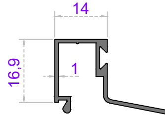
ISICAM ÇITA
