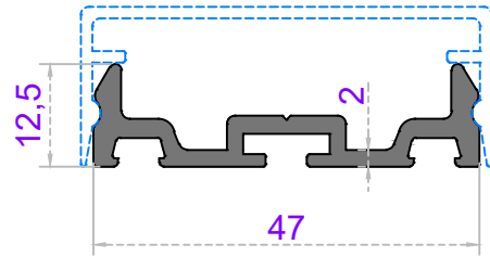
Sistem Kodu 50-1454 Ağırlık (kg/mt) 0,512
