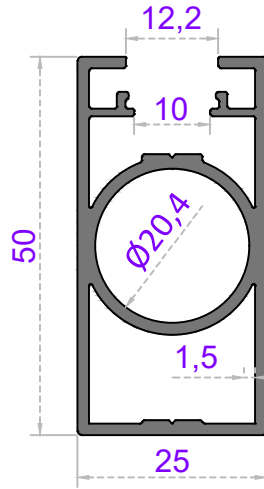
Sistem Kodu 58-2299 Ağırlık (kg/mt) 0,885
