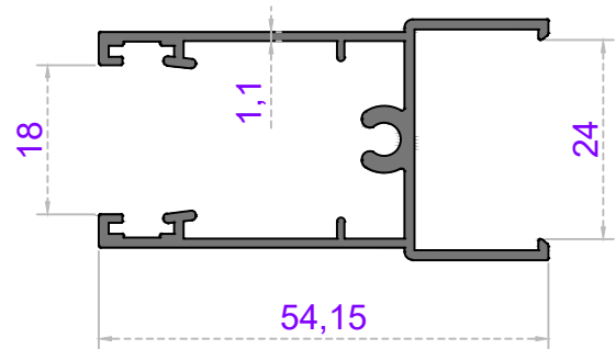
Sistem Kodu 49-4388 Ağırlık (kg/mt) 0,575
