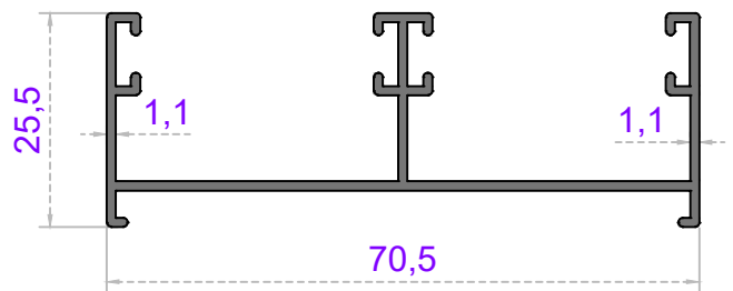
KASA ÜST
