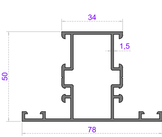
ORTA KAYIT
