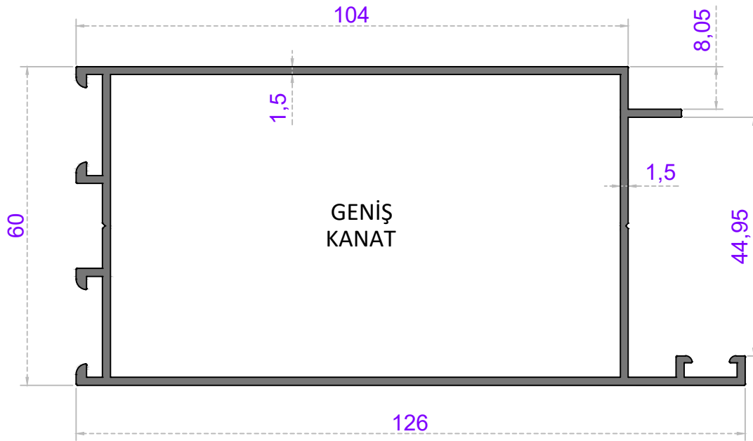
Sistem Kodu 62-1714 Ağırlık (kg/mt) 1,565
