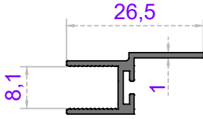
Sistem Kodu 41-2388 Ağırlık (kg/mt) 0,156
