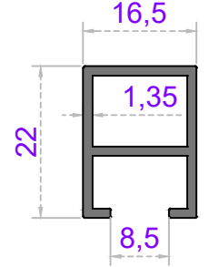
Sistem Kodu 58-2281 Ağırlık (kg/mt) 0,285
