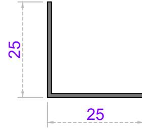
Sistem Kodu 24-302 Ağırlık (kg/mt) 0,132
