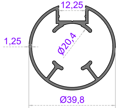
Ø 40'LIK DİKME
