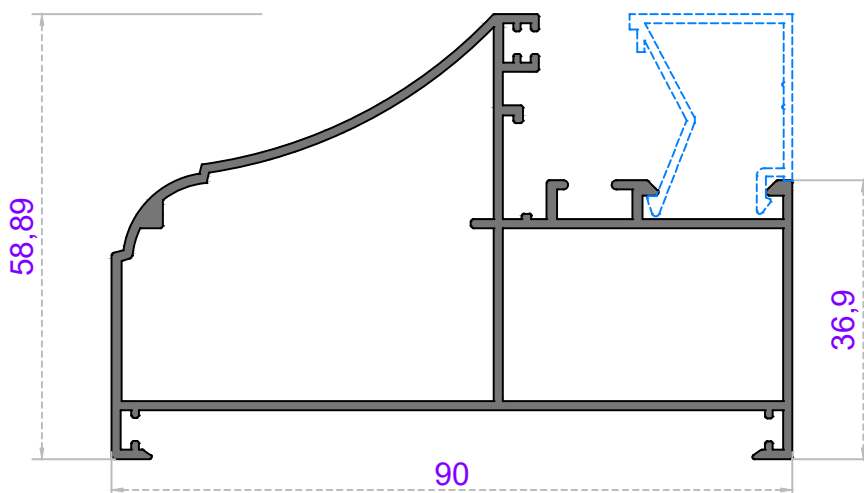
Sistem Kodu 49-4411 Ağırlık (kg/mt) 1,181
