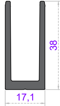
Sistem Kodu 36-1106 Ağırlık (kg/mt) 0,620
