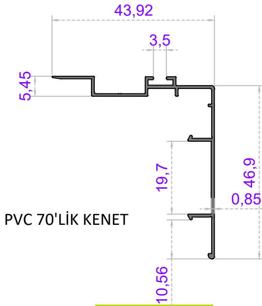
Sistem Kodu 64-1570 Ağırlık (kg/mt) 0,260
