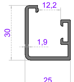
Sistem Kodu 58-2289 Ağırlık (kg/mt) 0,420
