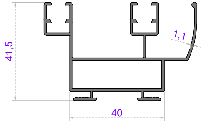
Sistem Kodu 49-4386 Ağırlık (kg/mt) 0,830
