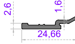
Sistem Kodu 54-4784 Ağırlık (kg/mt) 0,133
