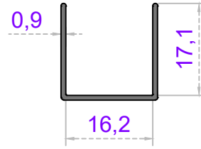
ASMA TAVAN -U-
