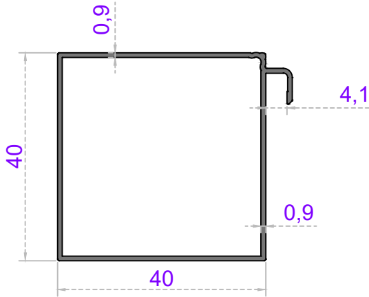
Sistem Kodu 48-4258 Ağırlık (kg/mt) 0,410
