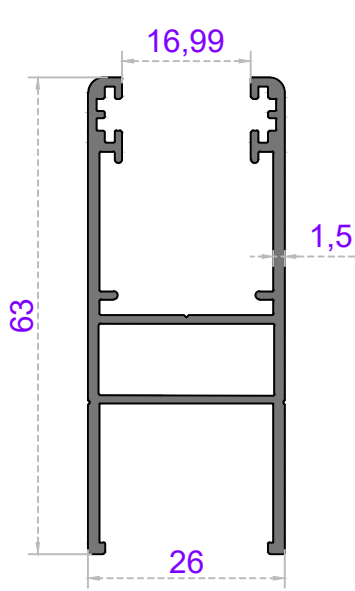
Sistem Kodu 53-4582 Ağırlık (kg/mt) 0,735
