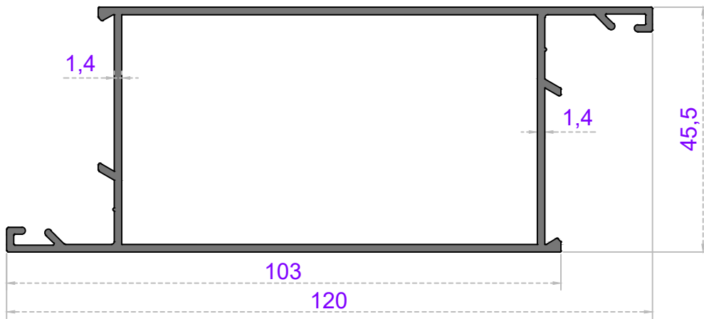
Sistem Kodu 32-1008 Ağırlık (kg/mt) 1,200
