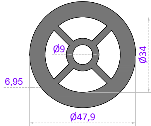
Sistem Kodu 58-2231 Ağırlık (kg/mt) 3,010
