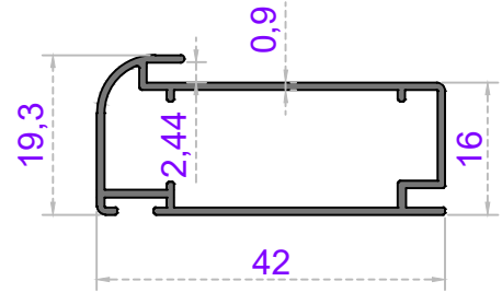
Sistem Kodu 48-4244 Ağırlık (kg/mt) 0,330
