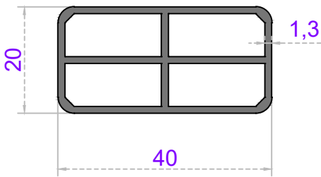
Sistem Kodu 20-138 Ağırlık (kg/mt) 0,590
