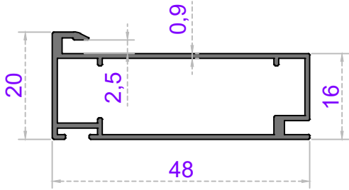
Sistem Kodu 48-4243 Ağırlık (kg/mt) 0,385
