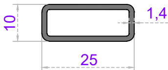
Sistem Kodu 58-2259 Ağırlık (kg/mt) 0,240
