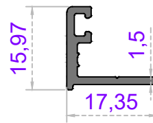
Sistem Kodu 54-4777 Ağırlık (kg/mt) 0,166
