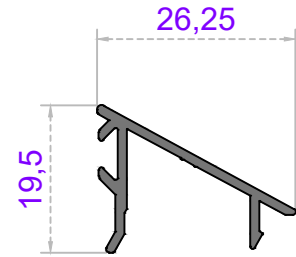
Sistem Kodu 54-4707 Ağırlık (kg/mt) 0,200
