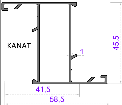
Sistem Kodu 32-1002 Ağırlık (kg/mt) 0,565
