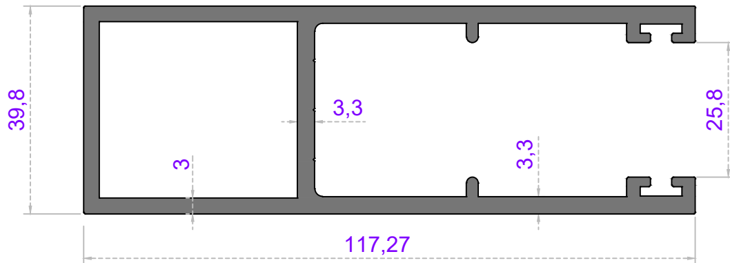
Sistem Kodu 38-1229 Ağırlık (kg/mt) 2,800
