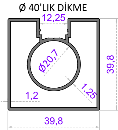
Sistem Kodu 58-2222 Ağırlık (kg/mt) 0,770
