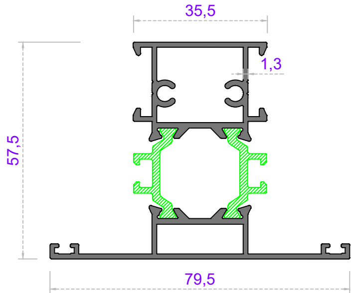
Sistem Kodu 70-3088 Ağırlık (kg/mt) 1,400
