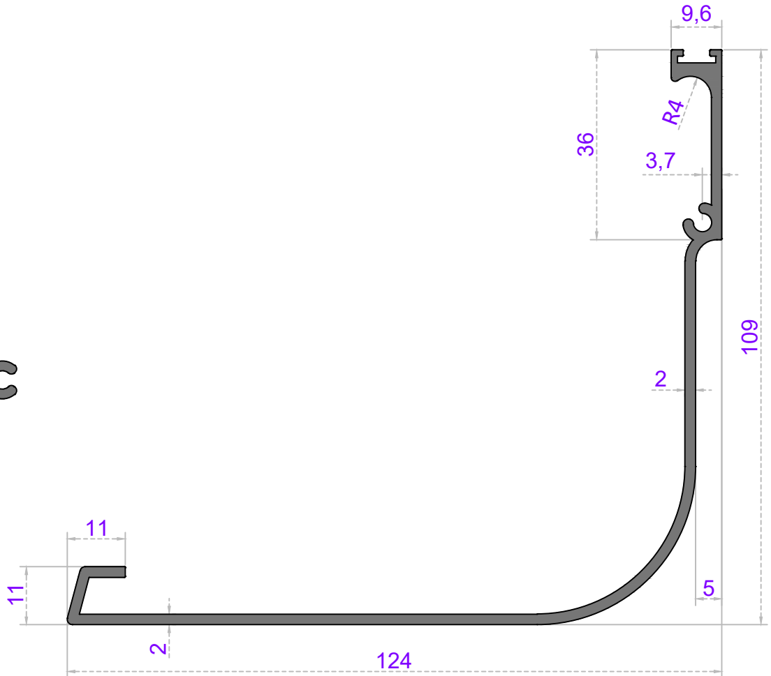
Sistem Kodu 39-1303 Ağırlık (kg/mt) 1,370
