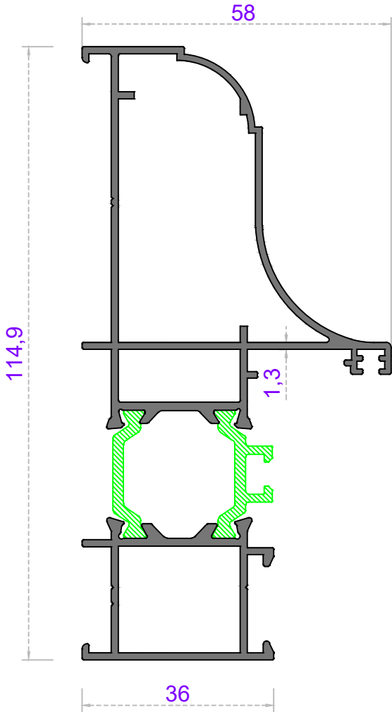
Sistem Kodu 70-3087 Ağırlık (kg/mt) 1,760
