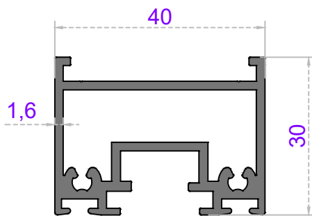
Sistem Kodu 32-1057 Ağırlık (kg/mt) 0,855
