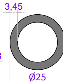
Sistem Kodu 22-240 Ağırlık (kg/mt) 0,635
