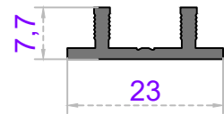
Sistem Kodu 54-4814 Ağırlık (kg/mt) 0,180
