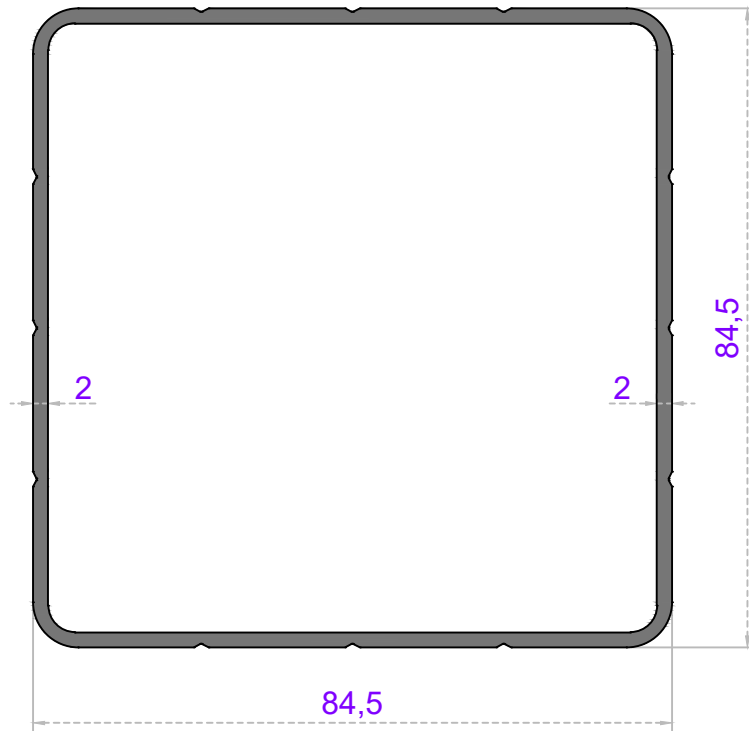
Sistem Kodu 57-2502 Ağırlık (kg/mt) 1,720
