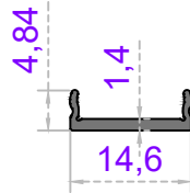
Sistem Kodu 58-2322 Ağırlık (kg/mt) 0,072
