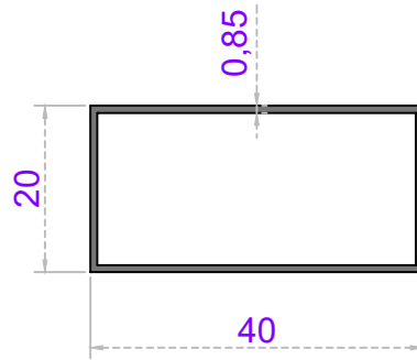
Sistem Kodu 20-101 Ağırlık (kg/mt) 0,275
