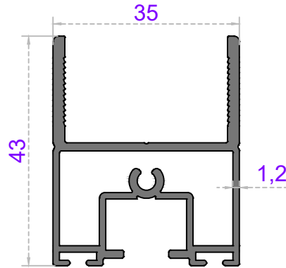
Sistem Kodu 41-2962 Ağırlık (kg/mt) 0,799
