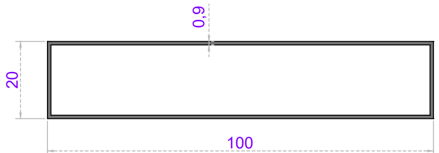
Sistem Kodu 20-156 Ağırlık (kg/mt) 0,580
