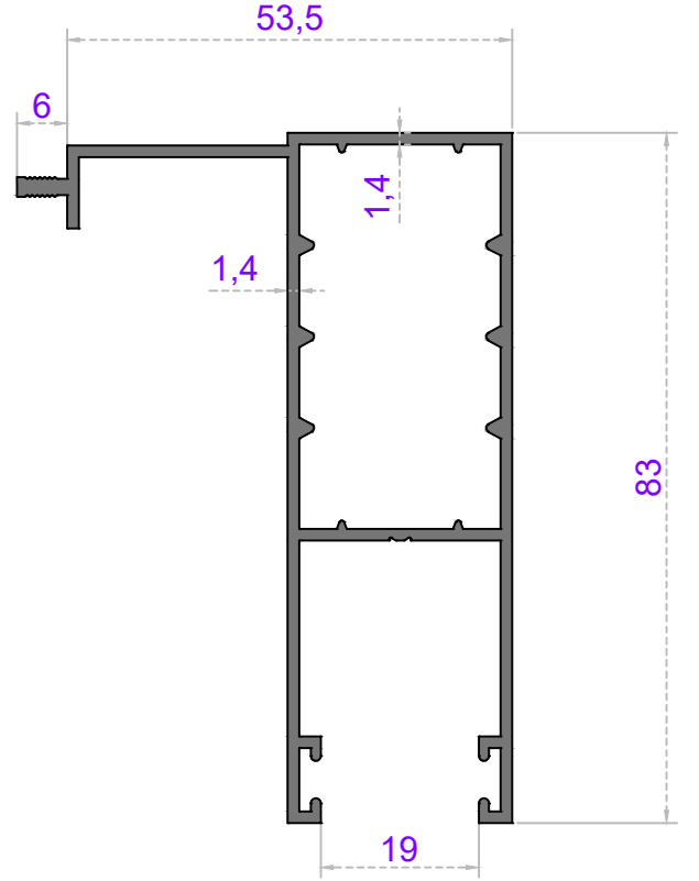
Sistem Kodu 54-4818 Ağırlık (kg/mt) 1,100
