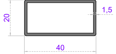
Sistem Kodu 20-213 Ağırlık (kg/mt) 0,465
