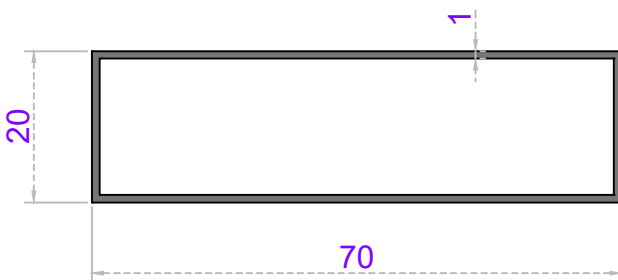
Sistem Kodu 20-160 Ağırlık (kg/mt) 0,480
