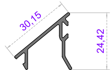
Sistem Kodu 54-4764 Ağırlık (kg/mt) 0,218
