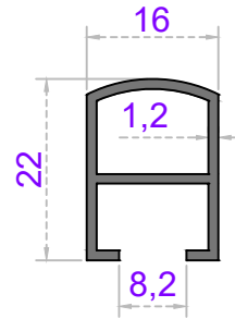
Sistem Kodu 58-2249 Ağırlık (kg/mt) 0,240
