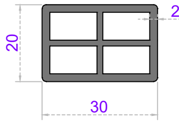
Sistem Kodu 20-141 Ağırlık (kg/mt) 0,665
