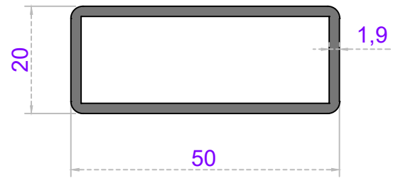
Sistem Kodu 20-130 Ağırlık (kg/mt) 0,677
