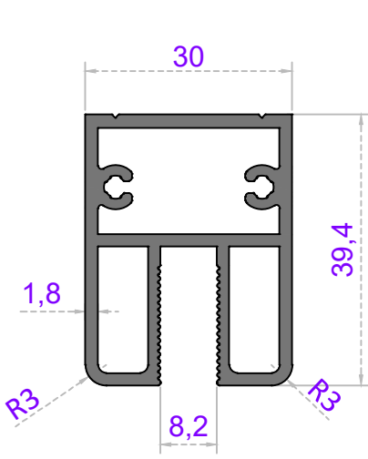
Sistem Kodu 41-2810 Ağırlık (kg/mt) 1,003
