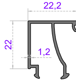
Sistem Kodu 49-4419 Ağırlık (kg/mt) 0,280
