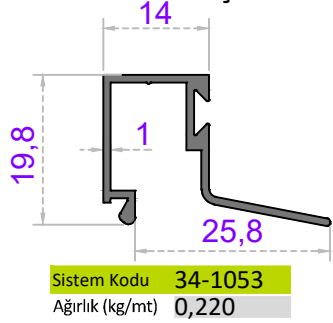
TEK CAM ÇONTASIZ ÇITA
