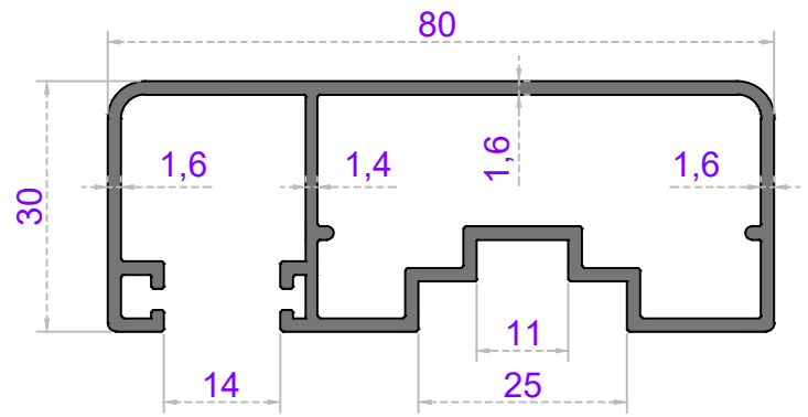
Sistem Kodu 58-2298 Ağırlık (kg/mt) 1,125
