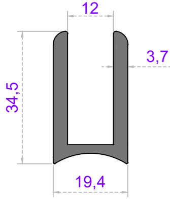
Sistem Kodu 58-2239 Ağırlık (kg/mt) 0,750
