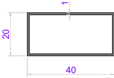
Sistem Kodu 20-161 Ağırlık (kg/mt) 0,315
