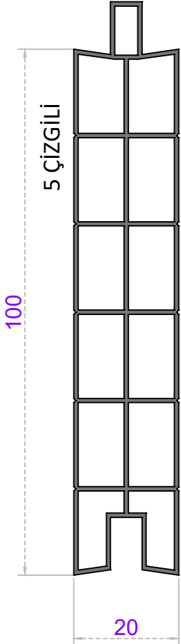
ÇİFT ODACIKLI 10'LUK KAPI LAMBRI
