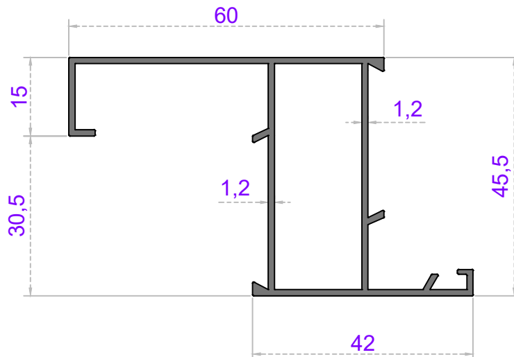
Sistem Kodu 32-1027 Ağırlık (kg/mt) 0,735
