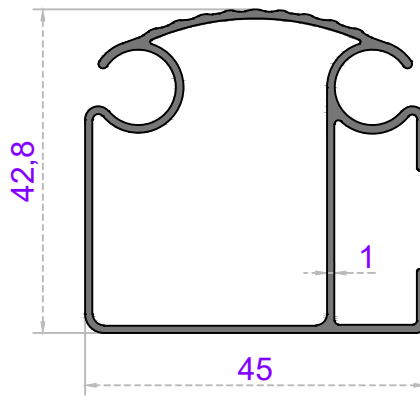
Sistem Kodu 57-2515 Ağırlık (kg/mt) 0,600
