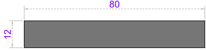
Sistem Kodu 58-2276 Ağırlık (kg/mt) 2,605
