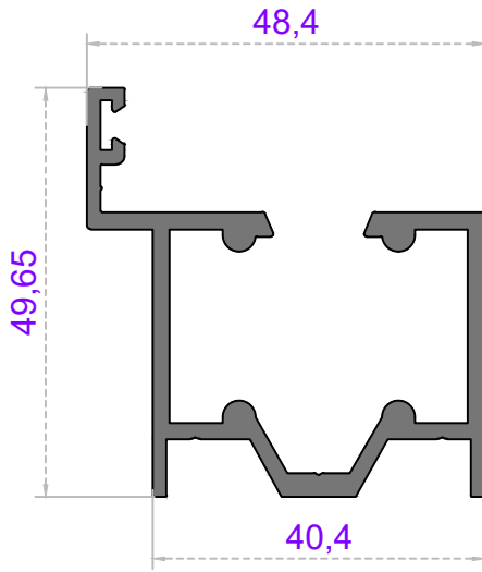
Sistem Kodu 32-1061 Ağırlık (kg/mt) 1,040
