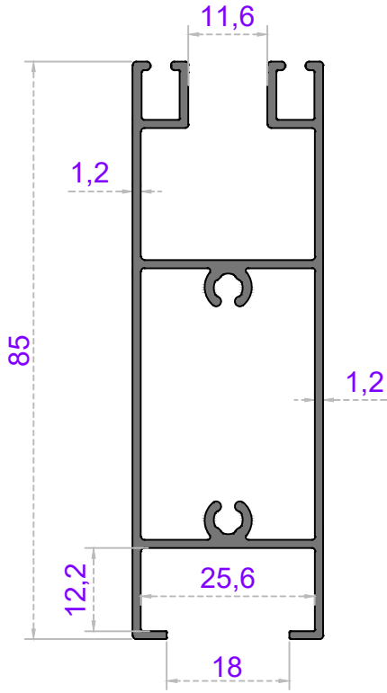
Sistem Kodu 39-1317 Ağırlık (kg/mt) 0,980
