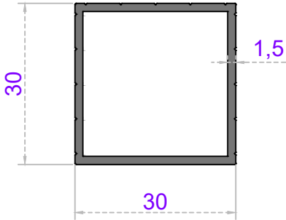
Sistem Kodu 20-127 Ağırlık (kg/mt) 0,465
