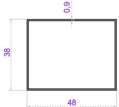
Sistem Kodu 20-113 Ağırlık (kg/mt) 0,415
