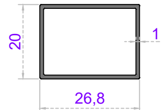
Sistem Kodu 20-184 Ağırlık (kg/mt) 0,245
