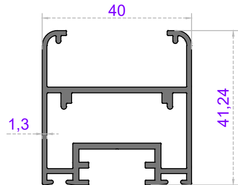
Sistem Kodu 32-1058 Ağırlık (kg/mt) 0,500
