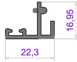
Sistem Kodu 32-1060 Ağırlık (kg/mt) 0,260
