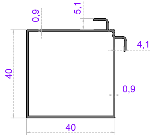
Sistem Kodu 48-4257 Ağırlık (kg/mt) 0,435
