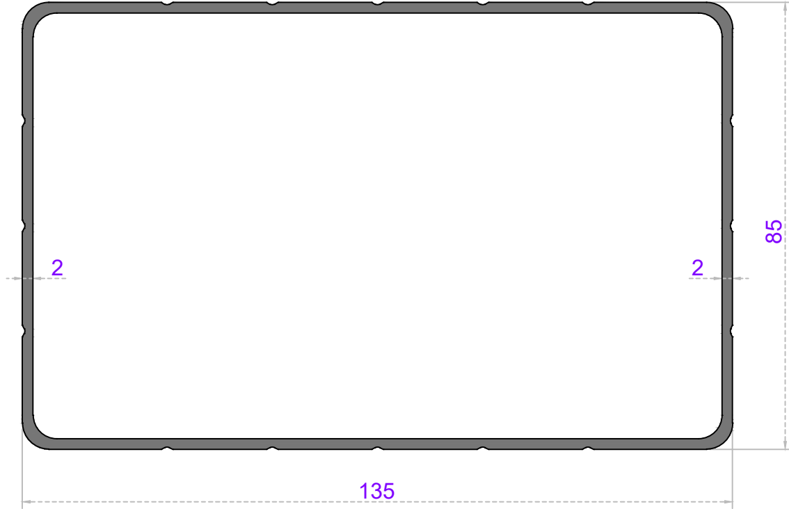
Sistem Kodu 57-2501 Ağırlık (kg/mt) 2,305
