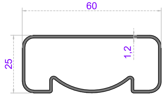
Sistem Kodu 58-2298 Ağırlık (kg/mt) 1,125
