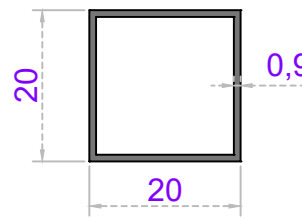
Sistem Kodu 20-182 Ağırlık (kg/mt) 0,190
