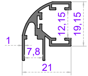
Sistem Kodu 41-2459 Ağırlık (kg/mt) 0,250
