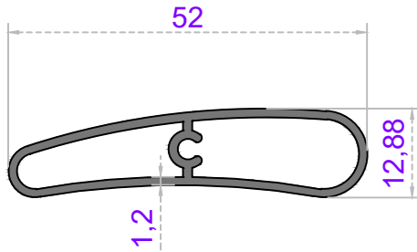
Sistem Kodu 32-1059 Ağırlık (kg/mt) 0,426
