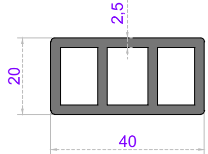
Sistem Kodu 20-129 Ağırlık (kg/mt) 0,950
