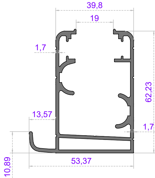
Sistem Kodu 41-2841 Ağırlık (kg/mt) 1,345
