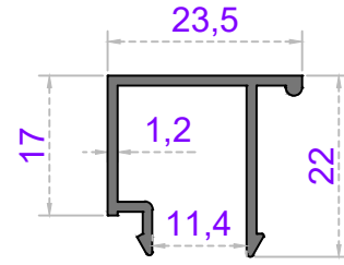
Sistem Kodu 60-1655 Ağırlık (kg/mt) 0,235
