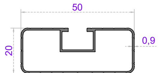
Sistem Kodu 58-2398 Ağırlık (kg/mt) 0,395
