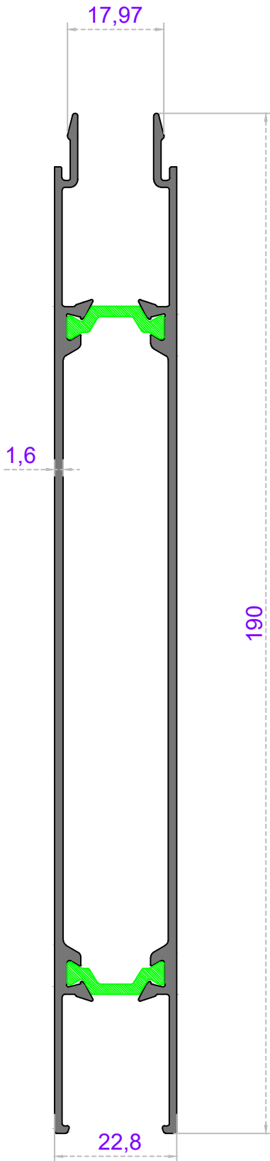
Sistem Kodu 66-1311 Ağırlık (kg/mt) 2,111
