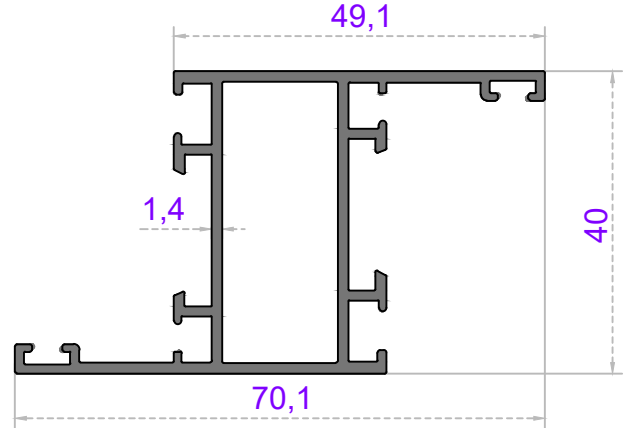
Sistem Kodu 53-4594 Ağırlık (kg/mt) 0,844
