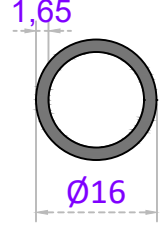
Sistem Kodu 22-208 Ağırlık (kg/mt) 0,205
