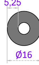
Sistem Kodu 22-207 Ağırlık (kg/mt) 0,480
