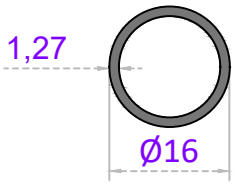
Sistem Kodu 22-220 Ağırlık (kg/mt) 0,160
