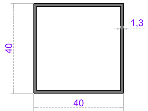
Sistem Kodu 20-226 Ağırlık (kg/mt) 0,550
