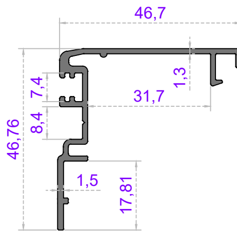
Sistem Kodu 47-4107 Ağırlık (kg/mt) 0,495
