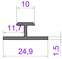
Sistem Kodu 39-1287 Ağırlık (kg/mt) 0,167
