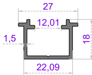
Sistem Kodu 47-4109 Ağırlık (kg/mt) 0,286
