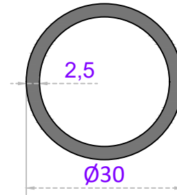
Sistem Kodu 22-201 Ağırlık (kg/mt) 0,586
