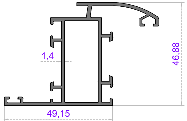
Sistem Kodu 53-4593 Ağırlık (kg/mt) 0,930
