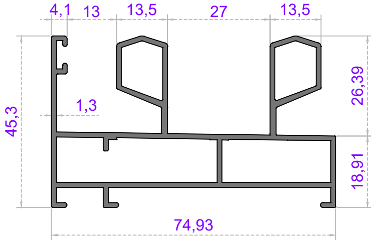
Sistem Kodu 47-4108 Ağırlık (kg/mt) 1,305
