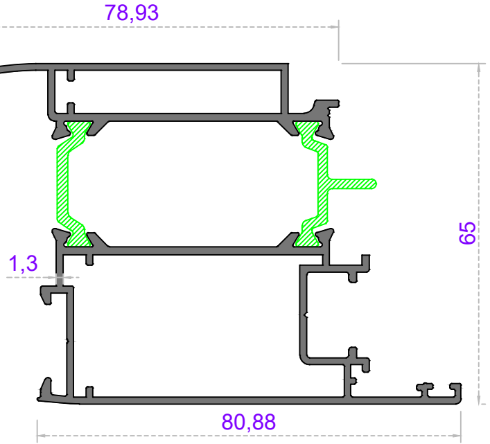
Sistem Kodu 70-3091 Ağırlık (kg/mt) 1,850
