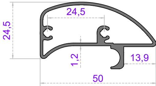
Sistem Kodu 65-1917 Ağırlık (kg/mt) 0,575
