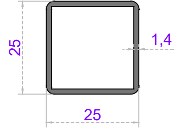
Sistem Kodu 20-131 Ağırlık (kg/mt) 0,350
