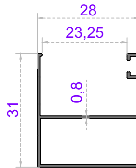
Sistem Kodu 40-1331 Ağırlık (kg/mt) 0,265
