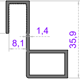
Sistem Kodu 41-2799 Ağırlık (kg/mt) 0,391
