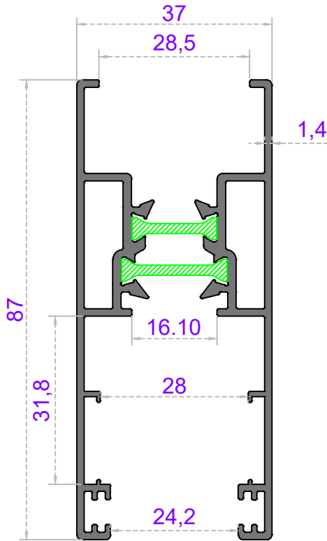
Sistem Kodu 47-4106 Ağırlık (kg/mt) 1,310
