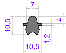
Sistem Kodu 64-1574 Ağırlık (kg/mt) 0,170
