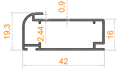
Sistem Kodu 48-4244 Ağırlık (kg/mt) 0,330
