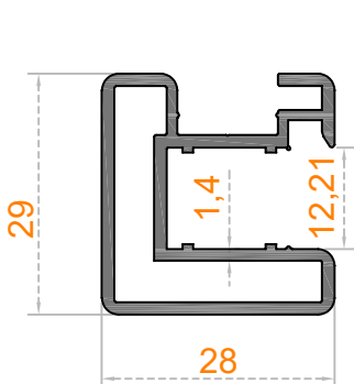
Sistem Kodu 41-2382 Ağırlık (kg/mt) 0,575
