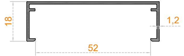
Sistem Kodu 50-1623 Ağırlık (kg/mt) 0,340
