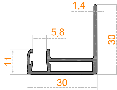
Sistem Kodu 30-543 Ağırlık (kg/mt) 0,370
