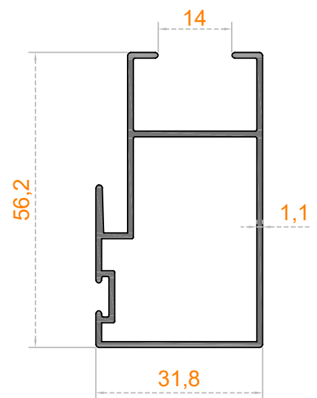
Sistem Kodu 49-4391 Ağırlık (kg/mt) 0,595
