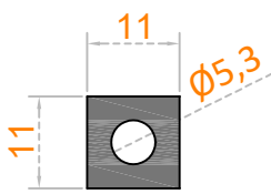
Sistem Kodu 58-2217 Ağırlık (kg/mt) 0,270
