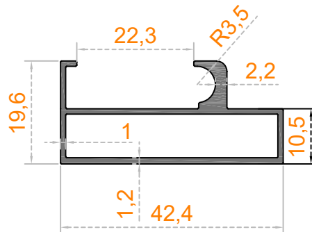
Sistem Kodu 65-1920 Ağırlık (kg/mt) 0,415
