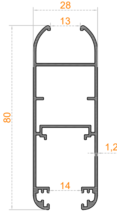
Sistem Kodu 85-1006 Ağırlık (kg/mt) 0,870
