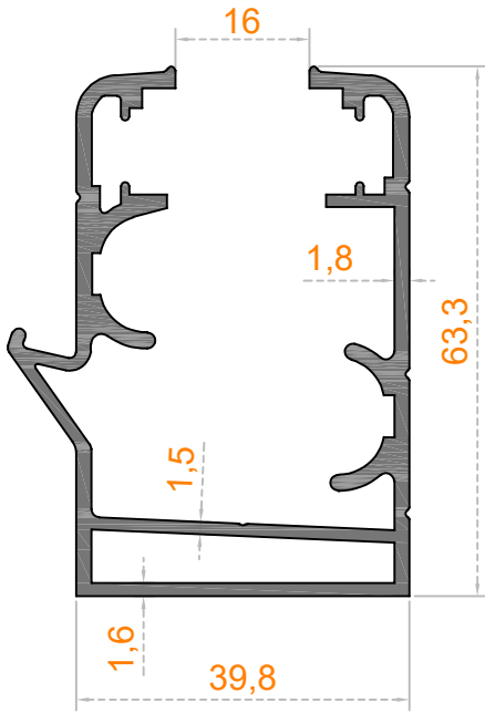
Sistem Kodu 41-2451 Ağırlık (kg/mt) 1,365
