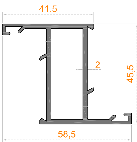
Sistem Kodu 32-1017 Ağırlık (kg/mt) 0,955
