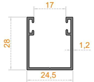
Sistem Kodu 53-4518 Ağırlık (kg/mt) 0,305
