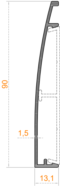
Sistem Kodu 48-4219 Ağırlık (kg/mt) 0,480
