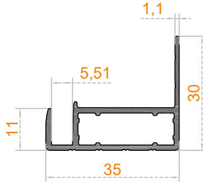
Sistem Kodu 30-546 Ağırlık (kg/mt) 0,402
