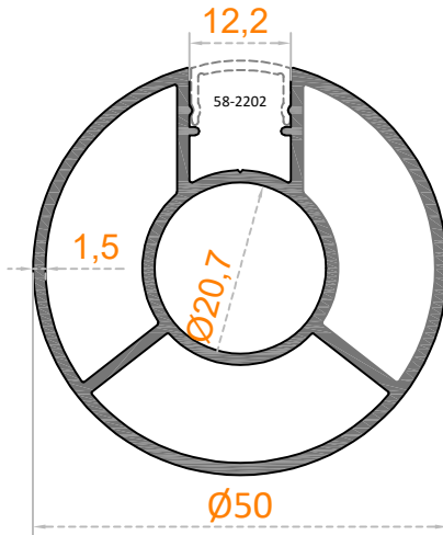
Ø 50'LİK DİKME
