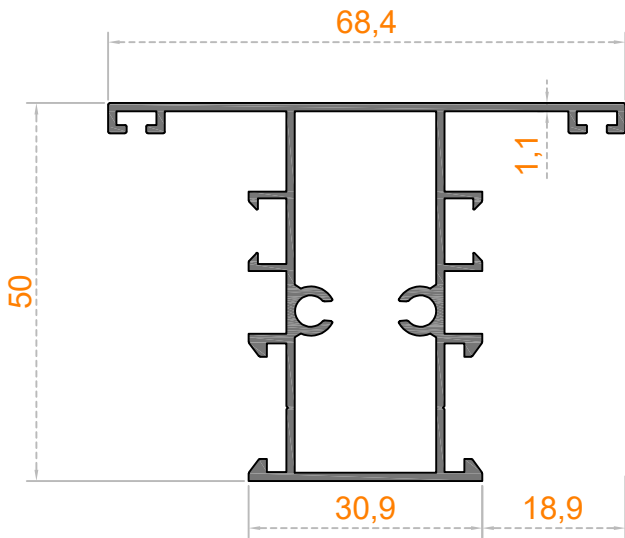
Sistem Kodu 53-4597 Ağırlık (kg/mt) 0,850
