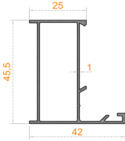
Sistem Kodu 32-1000 Ağırlık (kg/mt) 0,475
