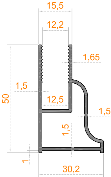
Sistem Kodu 58-2290 Ağırlık (kg/mt) 0,660
