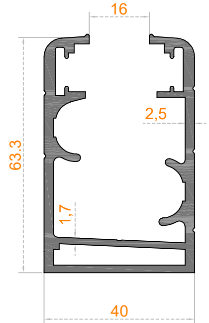
Sistem Kodu 41-2450 Ağırlık (kg/mt) 1,625
