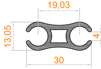
Sistem Kodu 57-2526 Ağırlık (kg/mt) 0,420
