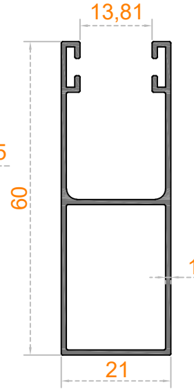
Sistem Kodu 38-1242 Ağırlık (kg/mt) 0,487
