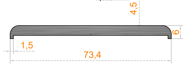
Sistem Kodu 58-2260 Ağırlık (kg/mt) 0,900
