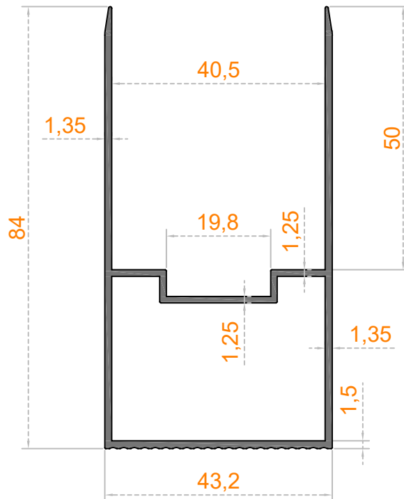
Sistem Kodu 41-2786 Ağırlık (kg/mt) 0,930
