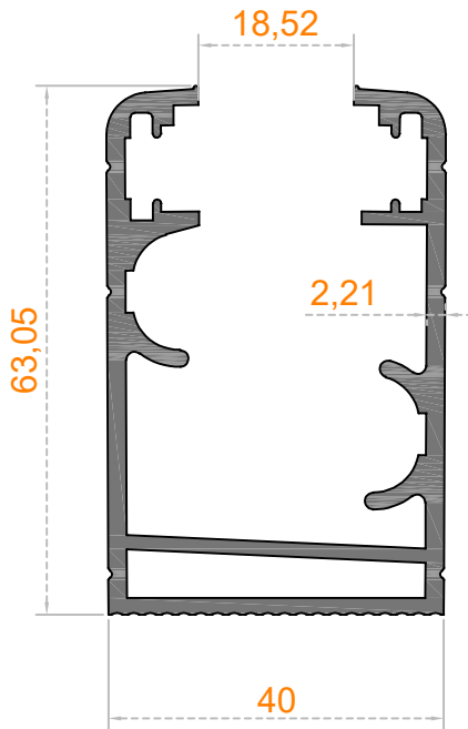
Sistem Kodu 41-2462 Ağırlık (kg/mt) 1,471
