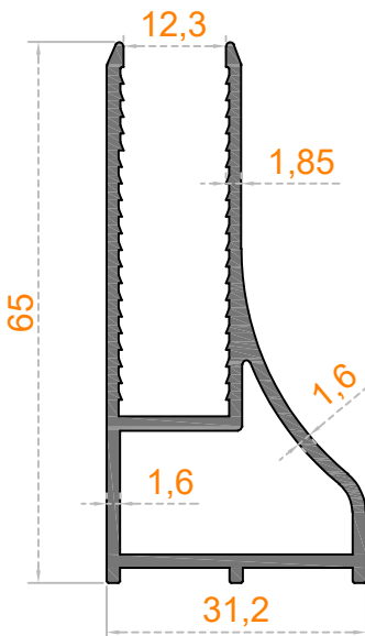
Sistem Kodu 58-2278 Ağırlık (kg/mt) 0,835
