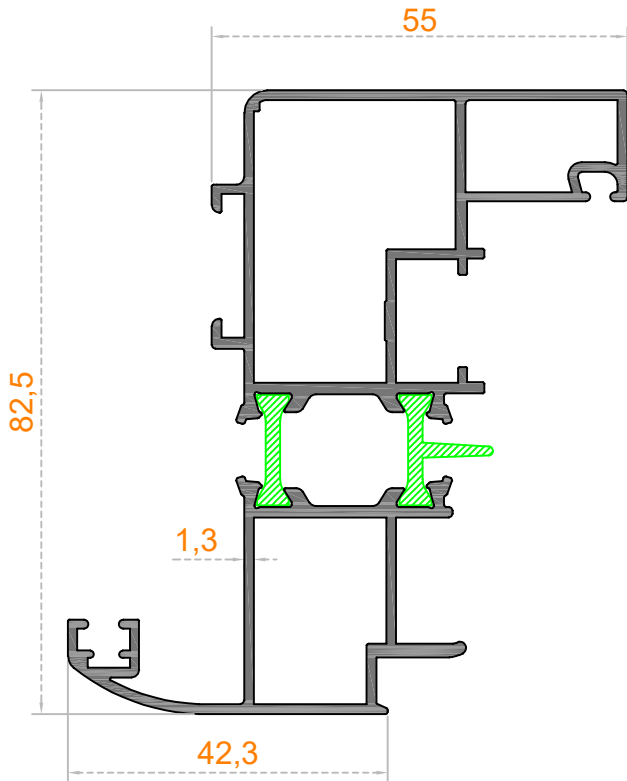
Sistem Kodu 70-3072 Ağırlık (kg/mt) 1,660
