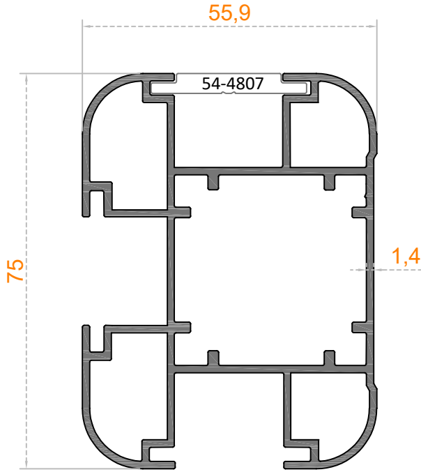
Sistem Kodu 54-4806 Ağırlık (kg/mt) 1,685
