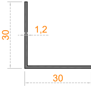
Sistem Kodu 24-303 Ağırlık (kg/mt) 0,191
