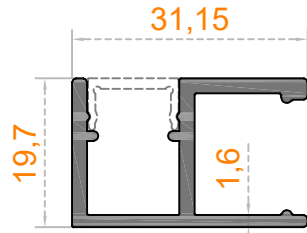
Sistem Kodu 58-2252 Ağırlık (kg/mt) 0,445
