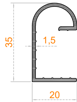
Sistem Kodu 48-4224 Ağırlık (kg/mt) 0,335
