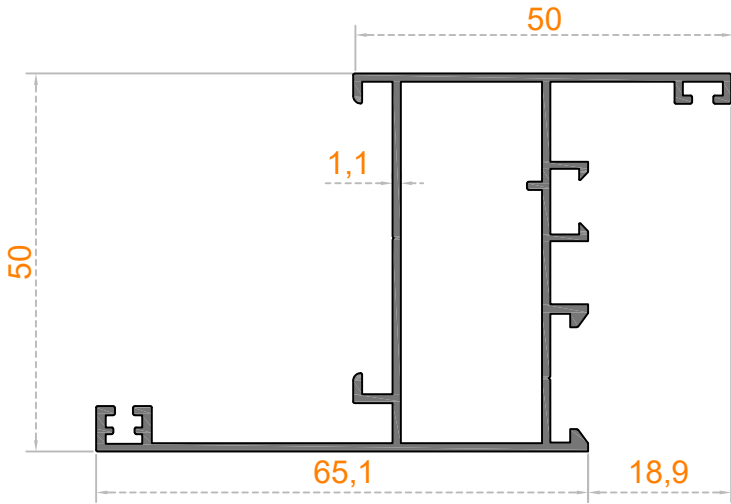
Sistem Kodu 53-4595 Ağırlık (kg/mt) 0,818
