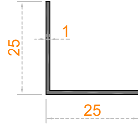
Sistem Kodu 24-302 Ağırlık (kg/mt) 0,132
