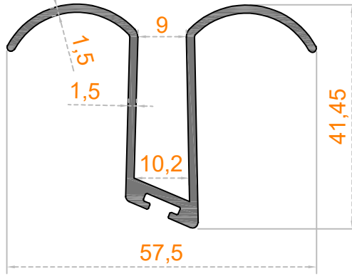
Sistem Kodu 41-2790 Ağırlık (kg/mt) 0,590
