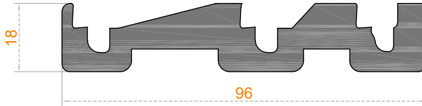
WİNAS PVC CAM ÇİTASI KESME KALIBI
