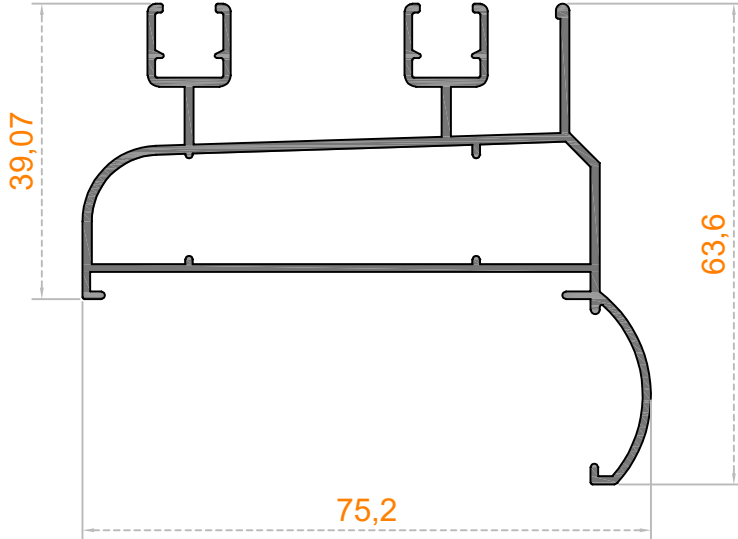
Sistem Kodu 49-4384 Ağırlık (kg/mt) 0,931
