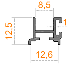
Sistem Kodu 41-2379 Ağırlık (kg/mt) 0,138
