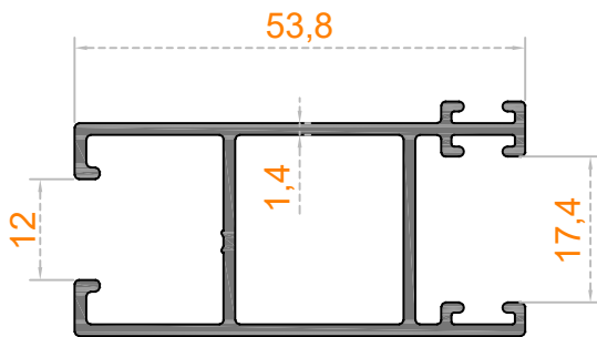
Sistem Kodu 54-4750 Ağırlık (kg/mt) 0,715
