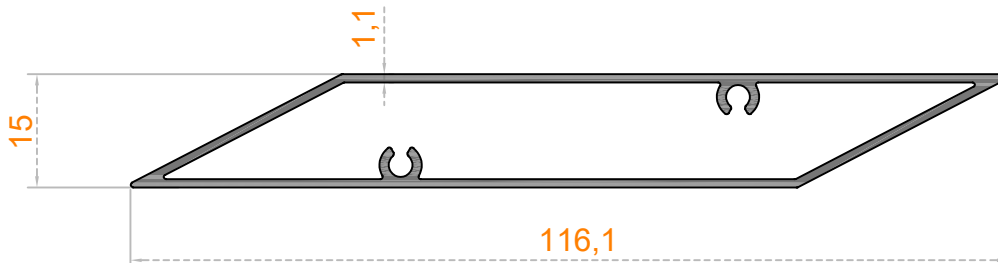
Sistem Kodu 20-145 Ağırlık (kg/mt) 0,586
