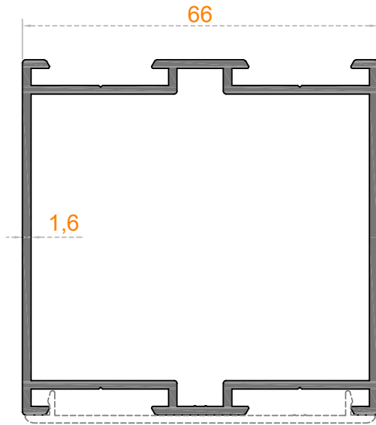
Sistem Kodu 54-4704 Ağırlık (kg/mt) 1,335
