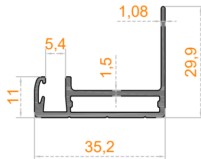
Sistem Kodu 30-549 Ağırlık (kg/mt) 0,418
