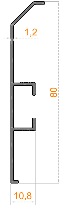
Sistem Kodu 48-4255 Ağırlık (kg/mt) 0,390
