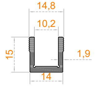
Sistem Kodu 41-2377 Ağırlık (kg/mt) 0,231
