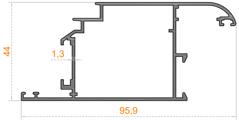
Sistem Kodu 85-1012 Ağırlık (kg/mt) 0,325
