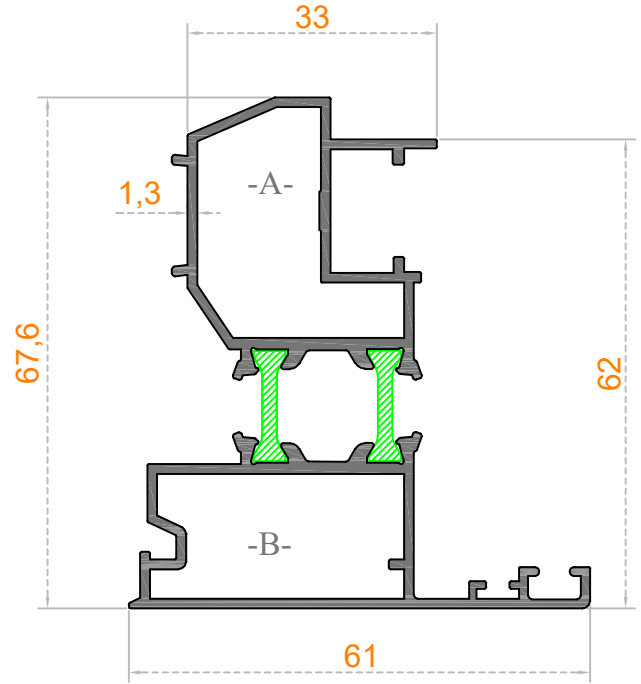
Sistem Kodu 70-3075 Ağırlık (kg/mt) 1,320
