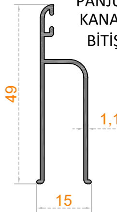
Sistem Kodu 47-4024 Ağırlık (kg/mt) 0,300
