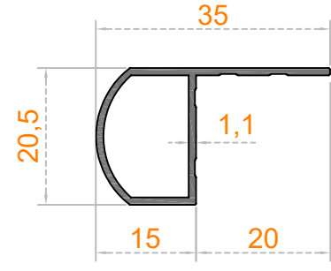
Sistem Kodu 48-4236 Ağırlık (kg/mt) 0,231
