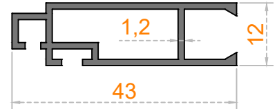
SİNEKLİK
