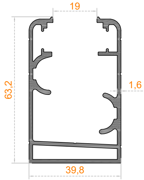
Sistem Kodu 41-2968 Ağırlık (kg/mt) 1,238
