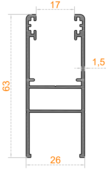
Sistem Kodu 53-4582 Ağırlık (kg/mt) 0,735
