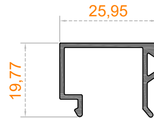
Sistem Kodu 54-4762 Ağırlık (kg/mt) 0,251
