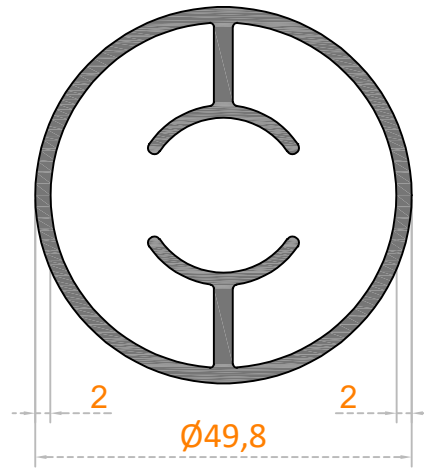
Ø 50'LİK DİKME
