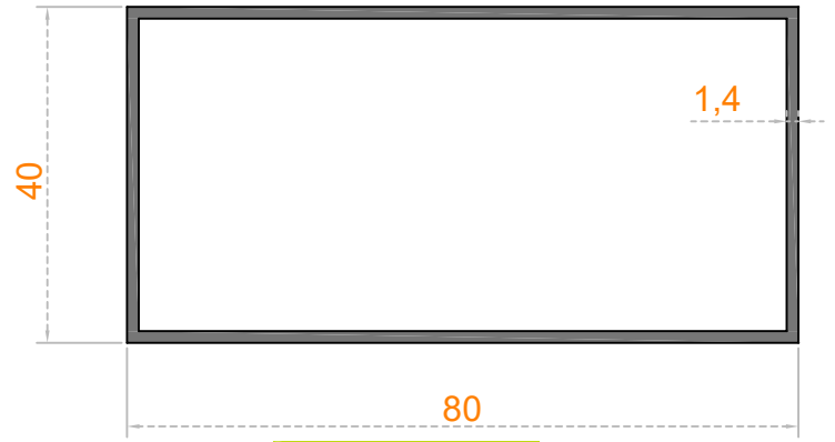
Sistem Kodu 20-108 Ağırlık (kg/mt) 0,910
