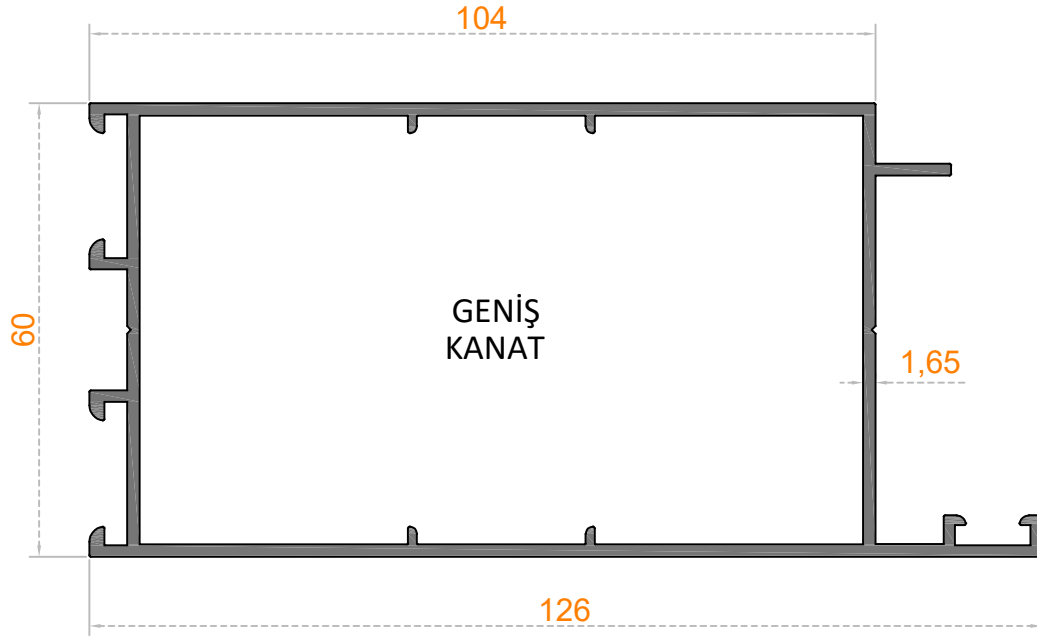
Sistem Kodu 62-1714 Ağırlık (kg/mt) 1,734
