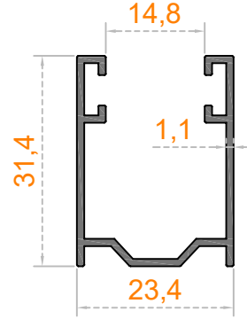
Sistem Kodu 53-4520 Ağırlık (kg/mt) 0,320
