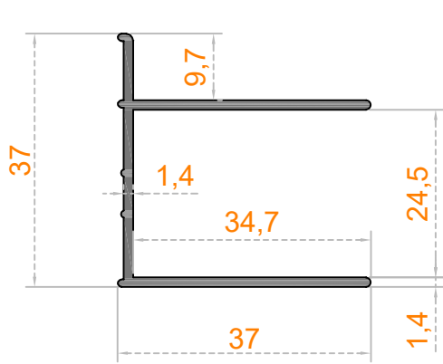
Sistem Kodu 65-1915 Ağırlık (kg/mt) 0,415
