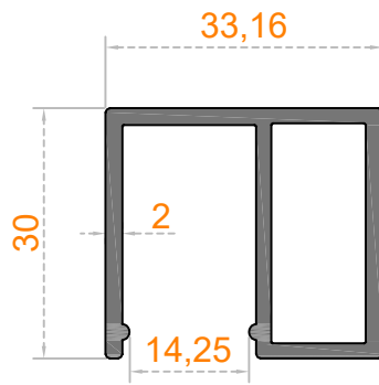
Sistem Kodu 58-2269 Ağırlık (kg/mt) 0,680
