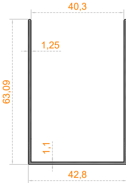
Sistem Kodu 41-2477 Ağırlık (kg/mt) 0,553
