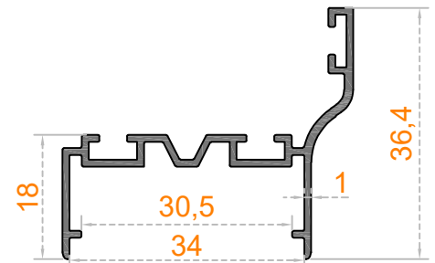
Sistem Kodu 41-2941 Ağırlık (kg/mt) 0,355
