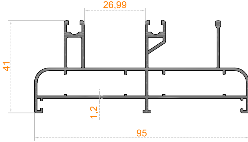
Sistem Kodu 85-1004 Ağırlık (kg/mt) 1,260
