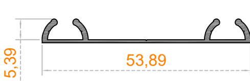
Sistem Kodu 48-4237 Ağırlık (kg/mt) 0,215
