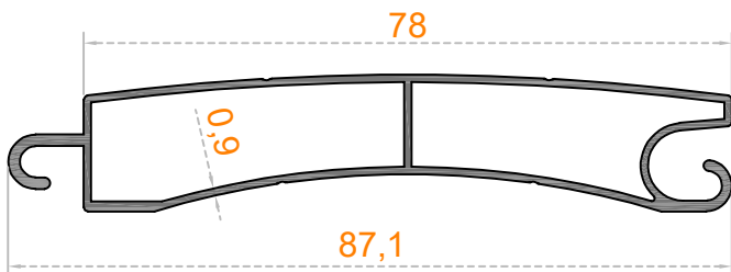
Sistem Kodu 38-1223 Ağırlık (kg/mt) 0,580
