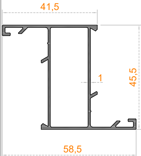
Sistem Kodu 32-1002 Ağırlık (kg/mt) 0,565
