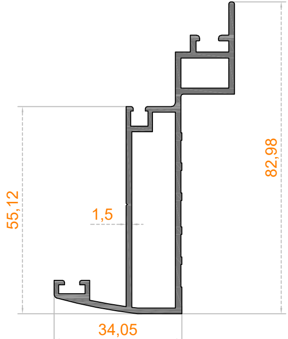
KAPAKLI CEPHE DIŞA AÇILIR KASA
