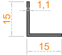
Sistem Kodu 24-300 Ağırlık (kg/mt) 0,086
