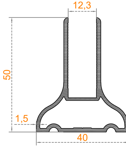
Sistem Kodu 58-2422 Ağırlık (kg/mt) 0,760
