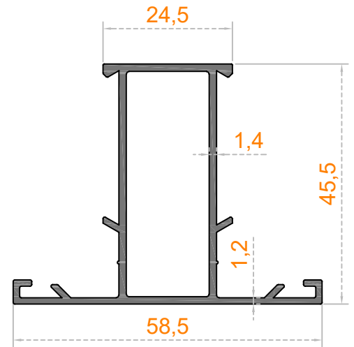
Sistem Kodu 32-1028 Ağırlık (kg/mt) 0,710
