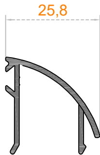
Sistem Kodu 54-4703 Ağırlık (kg/mt) 0,285
