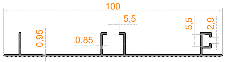
Sistem Kodu 48-4263 Ağırlık (kg/mt) 0,345
