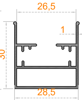
Sistem Kodu 40-1316 Ağırlık (kg/mt) 0,390
