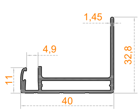
Sistem Kodu 30-547 Ağırlık (kg/mt) 0,432
