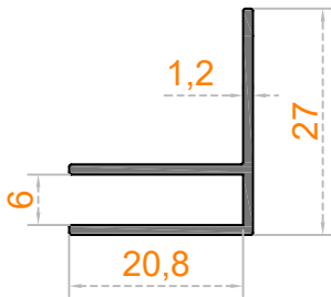
Sistem Kodu 62-1715 Ağırlık (kg/mt) 0,225
