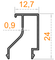
Sistem Kodu 53-4558 Ağırlık (kg/mt) 0,165
