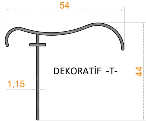
Sistem Kodu 26-403 Ağırlık (kg/mt) 0,360
