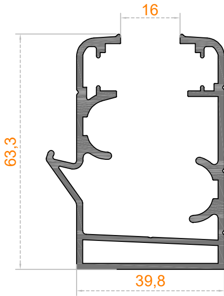
Sistem Kodu 41-2969 Ağırlık (kg/mt) 1,333
