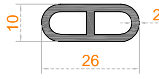
Sistem Kodu 48-4248 Ağırlık (kg/mt) 0,345
