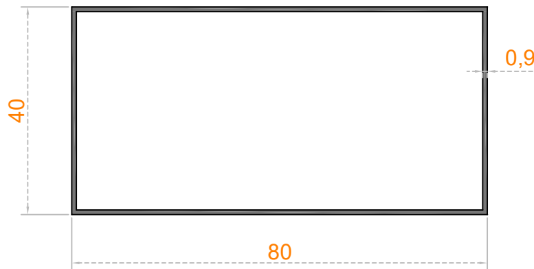
Sistem Kodu 20-145 Ağırlık (kg/mt) 0,586
