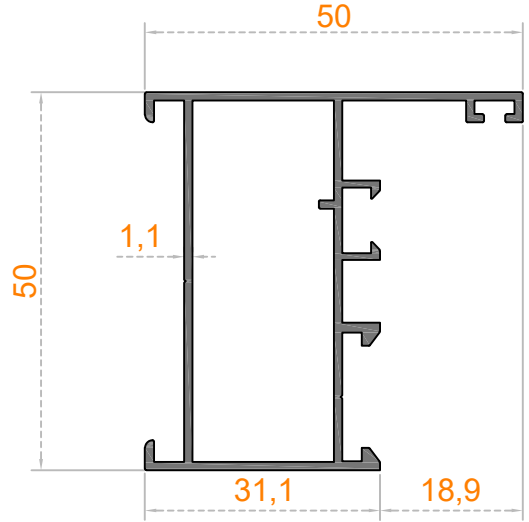
Sistem Kodu 53-4596 Ağırlık (kg/mt) 0,655
