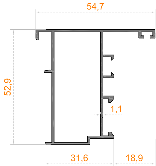
Sistem Kodu 53-4598 Ağırlık (kg/mt) 0,680
