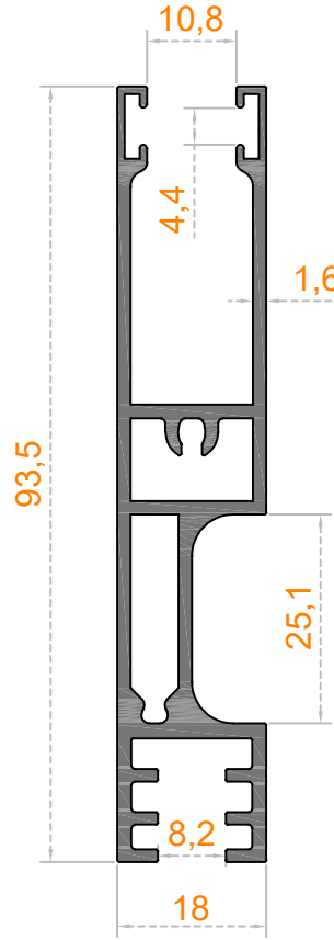
Sistem Kodu 41-2387 Ağırlık (kg/mt) 1,210
