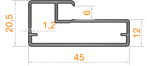
Sistem Kodu 48-4227 Ağırlık (kg/mt) 0,475
