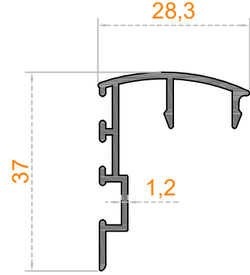
Sistem Kodu 85-1007 Ağırlık (kg/mt) 0,325
