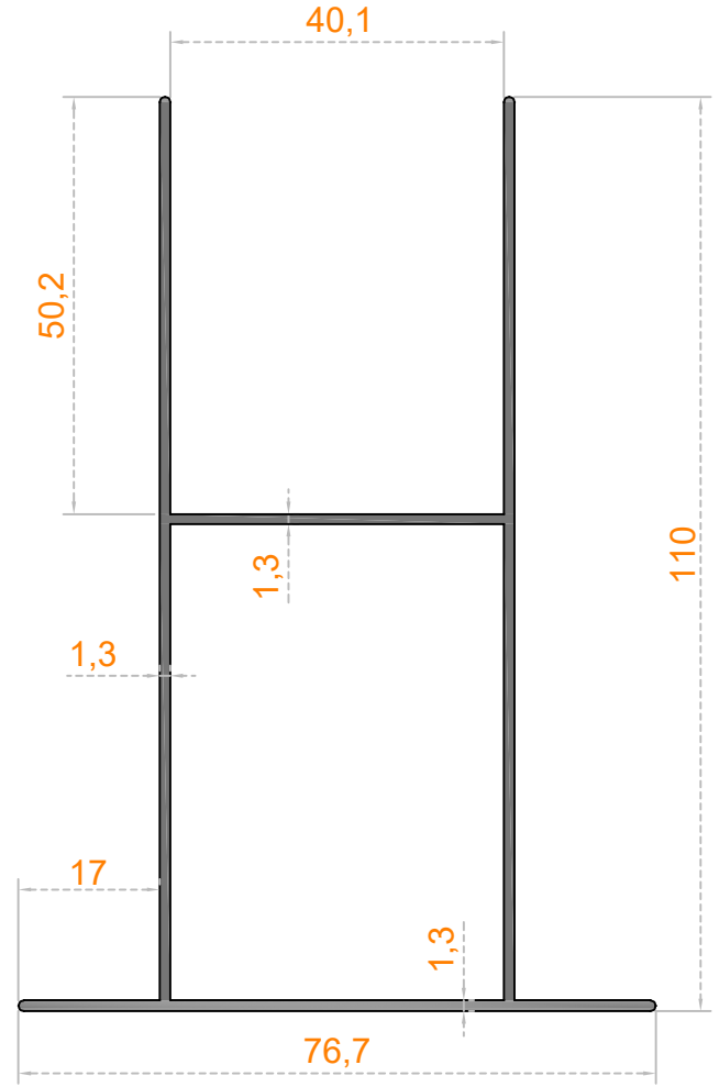
Sistem Kodu 41-2463 Ağırlık (kg/mt) 1,186
