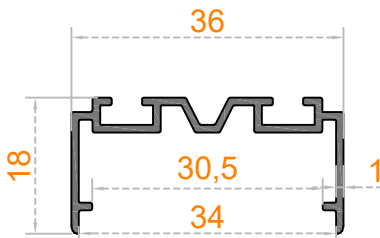
Sistem Kodu 41-2940 Ağırlık (kg/mt) 0,265
