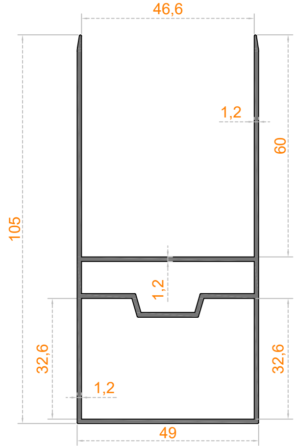
Sistem Kodu 41-2495 Ağırlık (kg/mt) 1,170
