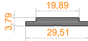
Sistem Kodu 54-4807 Ağırlık (kg/mt) 0,260
