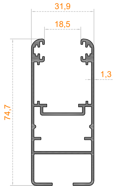
Sistem Kodu 46-6026 Ağırlık (kg/mt) 0,120
