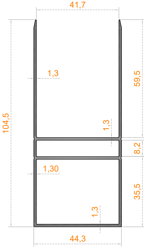
Sistem Kodu 41-2492 Ağırlık (kg/mt) 1,170
