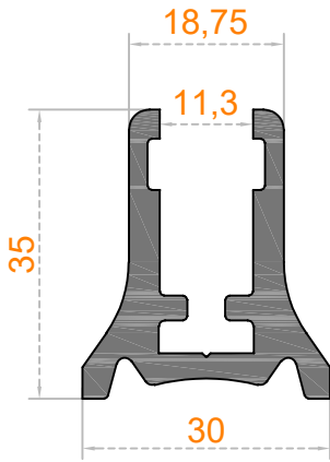
Sistem Kodu 58-2237 Ağırlık (kg/mt) 0,945
