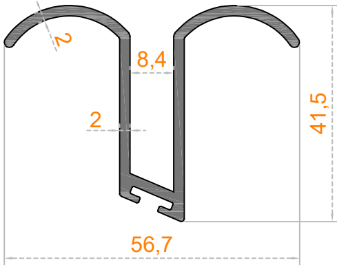
Sistem Kodu 41-2787 Ağırlık (kg/mt) 0,715
