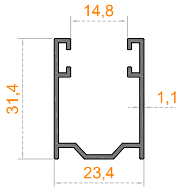
Sistem Kodu 53-4520 Ağırlık (kg/mt) 0,320
