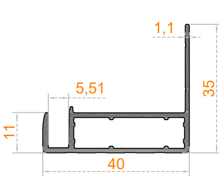
Sistem Kodu 30-545 Ağırlık (kg/mt) 0,428
