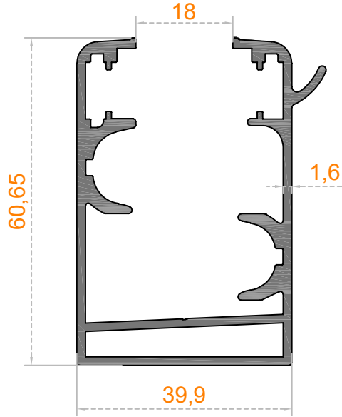
Sistem Kodu 41-2971 Ağırlık (kg/mt) 1,320
