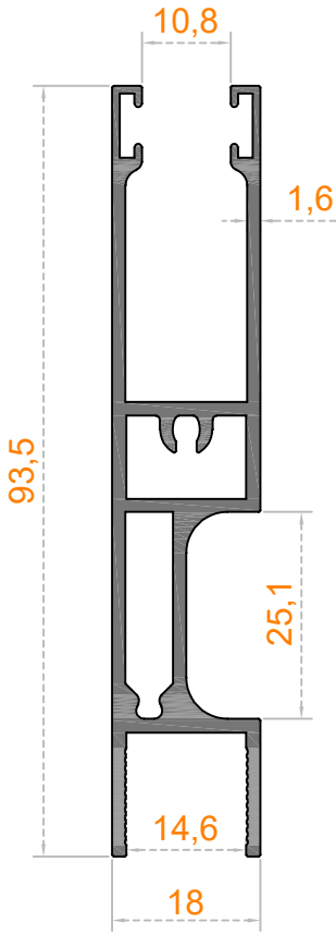
Sistem Kodu 41-2375 Ağırlık (kg/mt) 1,125
