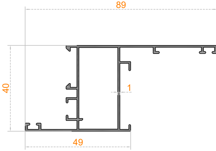
Sistem Kodu 53-4562 Ağırlık (kg/mt) 0,665
