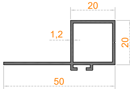
Sistem Kodu 39-1346 Ağırlık (kg/mt) 0,385
