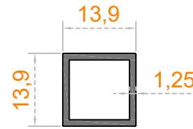
Sistem Kodu 58-2420 Ağırlık (kg/mt) 0,176
