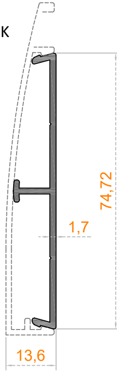
Sistem Kodu 48-4220 Ağırlık (kg/mt) 0,450
