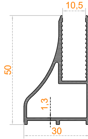
Sistem Kodu 58-2365 Ağırlık (kg/mt) 0,620
