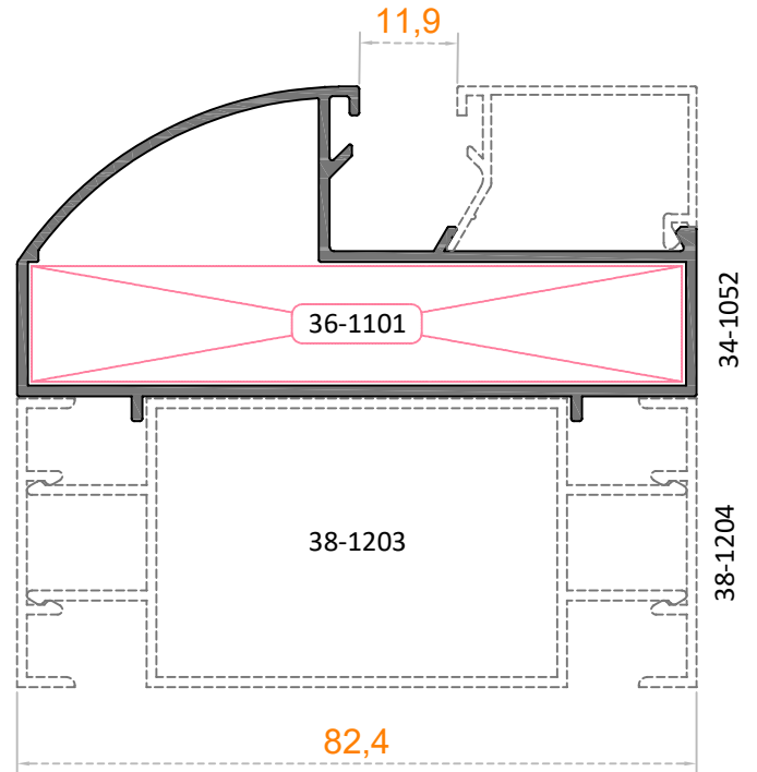
MONTAJ DETAYI
