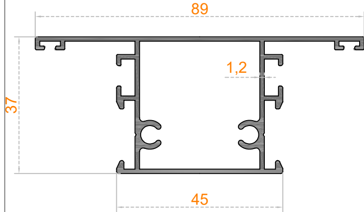
Sistem Kodu 49-4408 Ağırlık (kg/mt) 0,945
