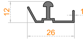
Sistem Kodu 45-1432 Ağırlık (kg/mt) 0,180
