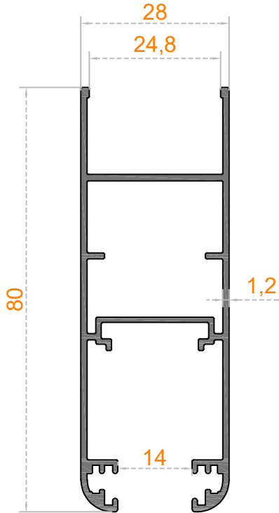
Sistem Kodu 85-1005 Ağırlık (kg/mt) 0,855
