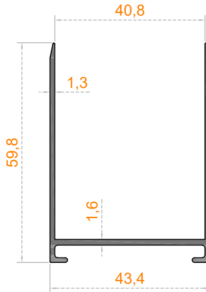
Sistem Kodu 41-2491 Ağırlık (kg/mt) 0,615
