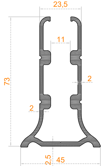
Sistem Kodu 58-2211 Ağırlık (kg/mt) 1,490
