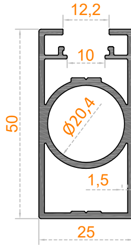
Sistem Kodu 58-2299 Ağırlık (kg/mt) 0,885
