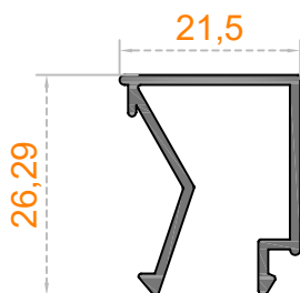
Sistem Kodu 85-1014 Ağırlık (kg/mt) 0,325
