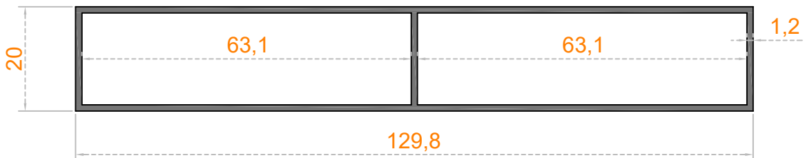
Sistem Kodu 20-158 Ağırlık (kg/mt) 1,020
