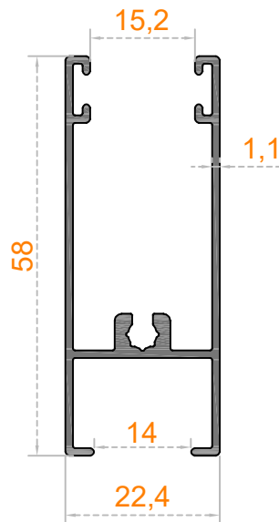
Sistem Kodu 49-4390 Ağırlık (kg/mt) 0,531
