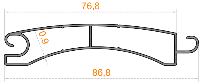
Sistem Kodu 38-1217 Ağırlık (kg/mt) 0,580
