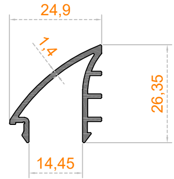
Sistem Kodu 58-2286 Ağırlık (kg/mt) 0,290
