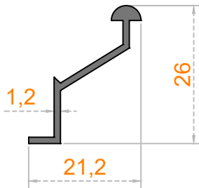
Sistem Kodu 45-1433 Ağırlık (kg/mt) 0,152
