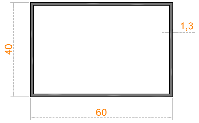
Sistem Kodu 20-122 Ağırlık (kg/mt) 0,700
