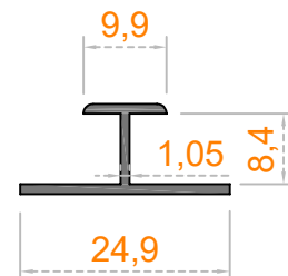
Sistem Kodu 39-1288 Ağırlık (kg/mt) 0,132
