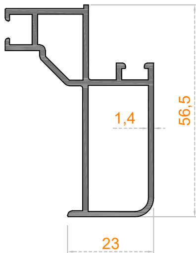
KAPAKLI CEPHE DIŞA AÇILIR KANAT
