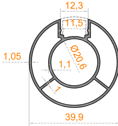
Ø 40'LİK DİKME
