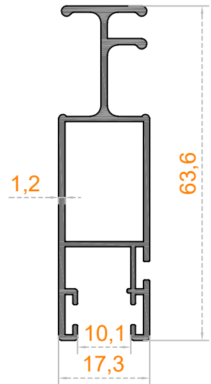
Sistem Kodu 85-1009 Ağırlık (kg/mt) 0,585
