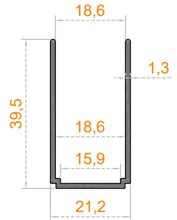
Sistem Kodu 41-2793 Ağırlık (kg/mt) 0,345
