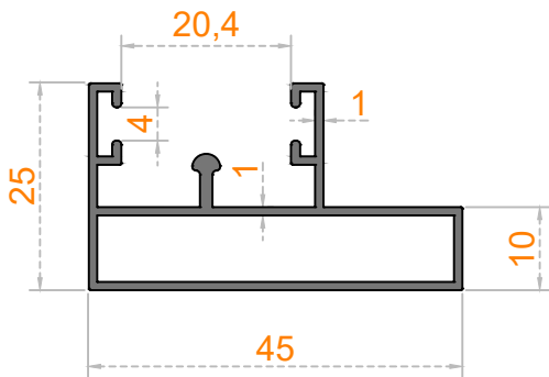
Sistem Kodu 45-1436 Ağırlık (kg/mt) 0,455
