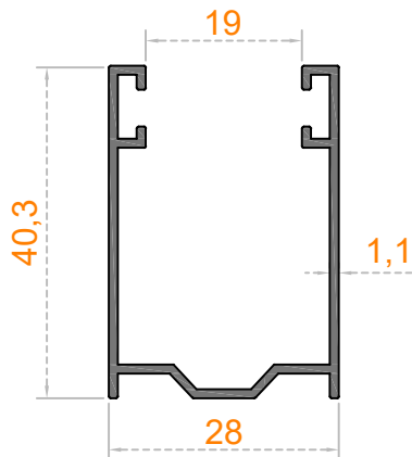
Sistem Kodu 53-4521 Ağırlık (kg/mt) 0,390
