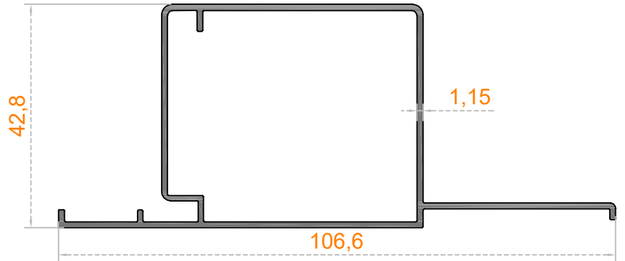
Sistem Kodu 50-1653 Ağırlık (kg/mt) 0,780
