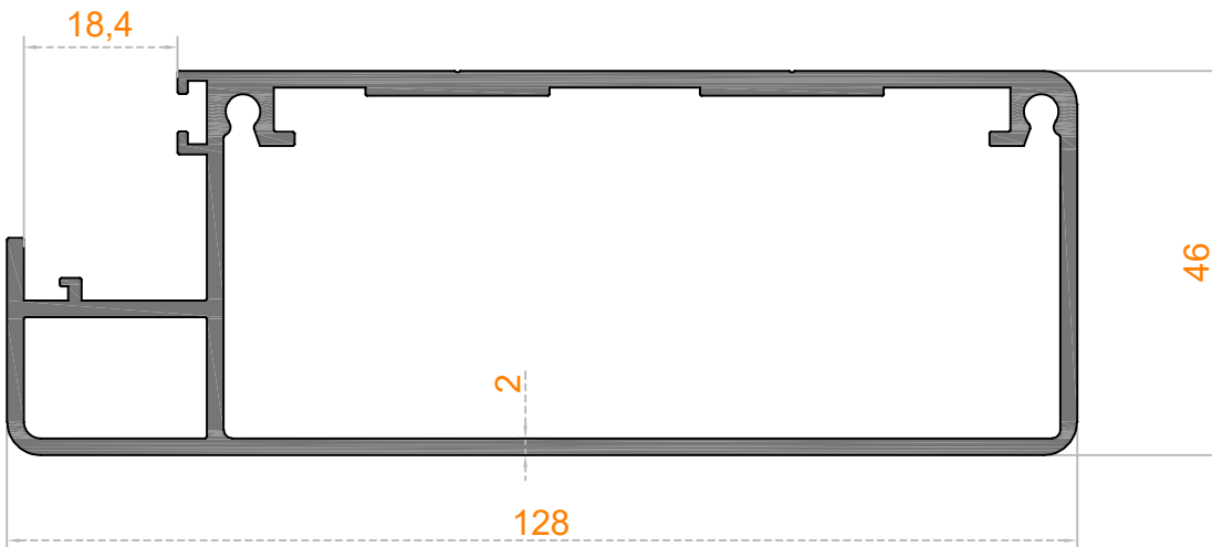
Sistem Kodu 54-4724 Ağırlık (kg/mt) 2,030
