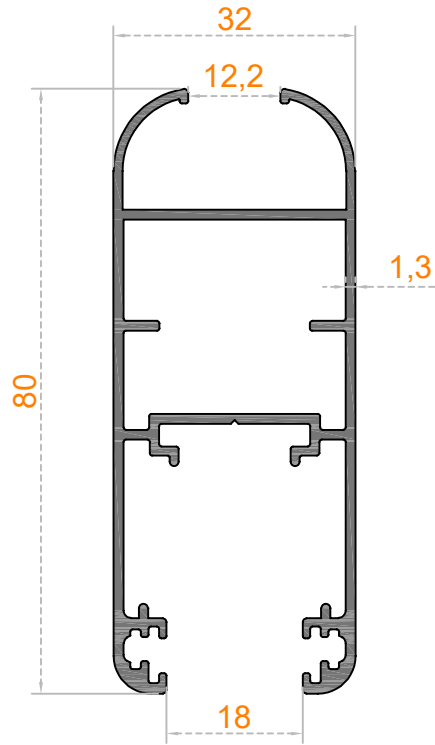
Sistem Kodu 49-4429 Ağırlık (kg/mt) 1,025
