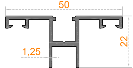
Sistem Kodu 50-1605 Ağırlık (kg/mt) 0,465
