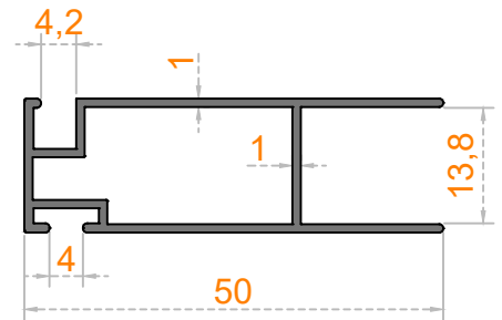
Sistem Kodu 45-1437 Ağırlık (kg/mt) 0,390
