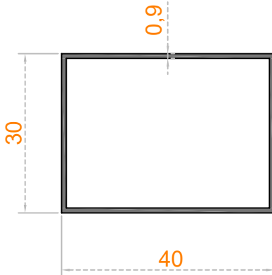
Sistem Kodu 20-102 Ağırlık (kg/mt) 0,335
