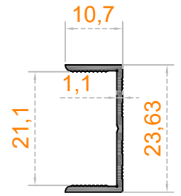
Sistem Kodu 48-4256 Ağırlık (kg/mt) 0,130
