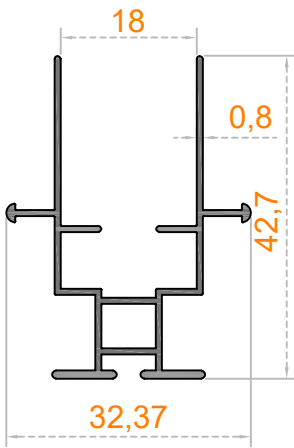
Sistem Kodu 40-1314 Ağırlık (kg/mt) 0,345
