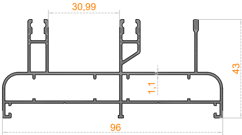
Sistem Kodu 49-4427 Ağırlık (kg/mt) 1,230
