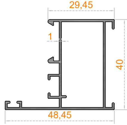
Sistem Kodu 53-4554 Ağırlık (kg/mt) 0,520
