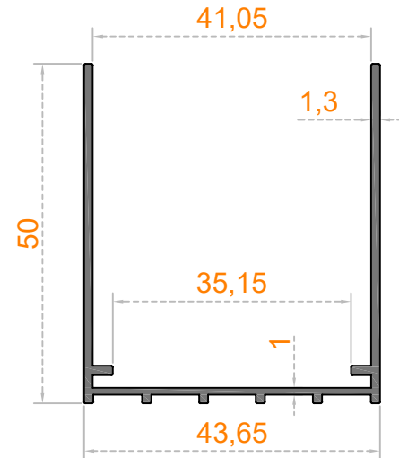
Sistem Kodu 41-2717 Ağırlık (kg/mt) 0,510
