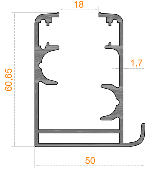
Sistem Kodu 41-2970 Ağırlık (kg/mt) 1,386
