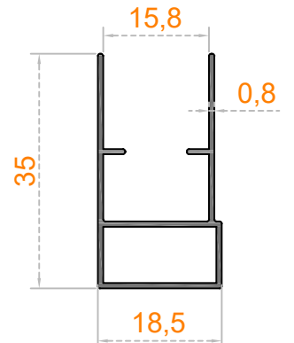
Sistem Kodu 40-1323 Ağırlık (kg/mt) 0,240
