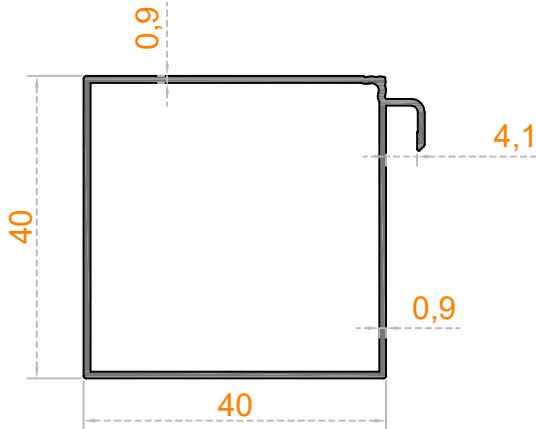
Sistem Kodu 48-4258 Ağırlık (kg/mt) 0,410
