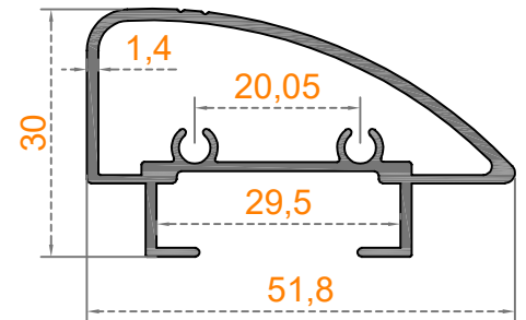
Sistem Kodu 65-1924 Ağırlık (kg/mt) 0,613
