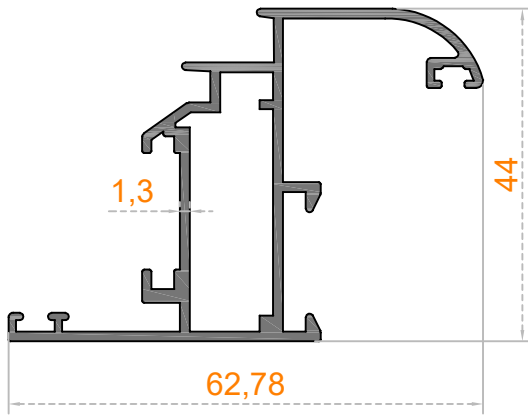
Sistem Kodu 85-1011 Ağırlık (kg/mt) 0,325
